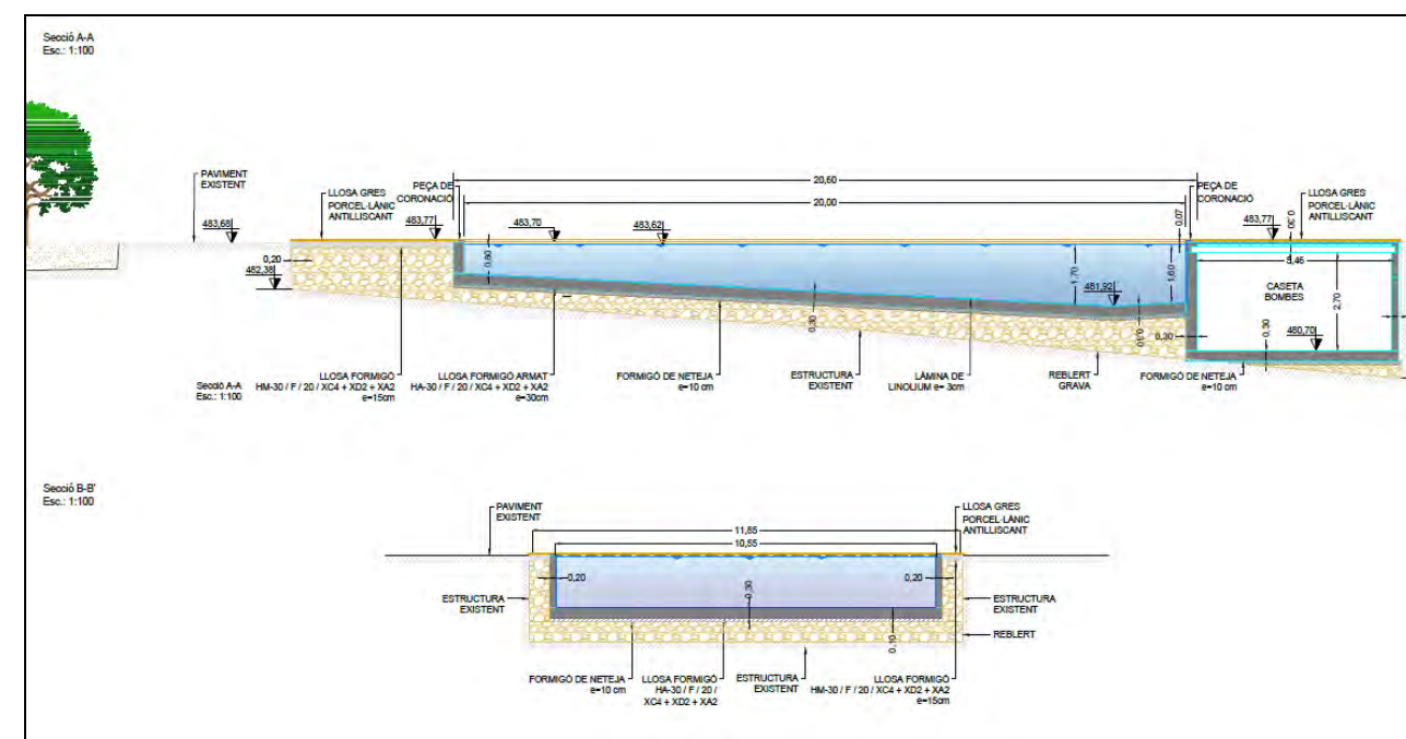
Figura núm. 15 Seccions Longitudinal i Transversal
