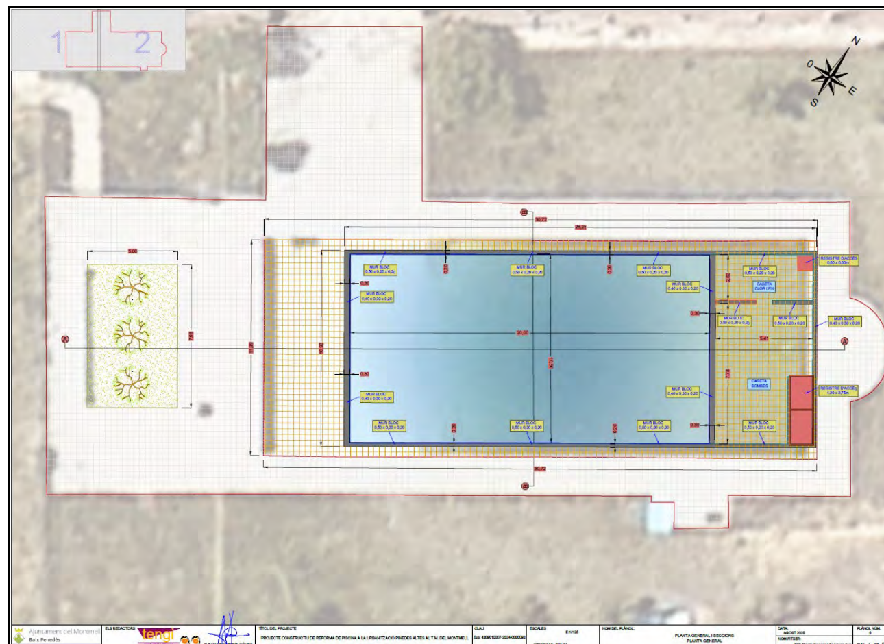
Figura núm. 14 Planta General actuacions
