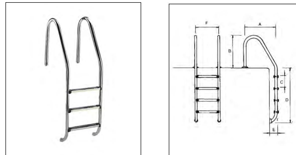
Figura núm. 22 Escala per accés i sortida de la piscina
