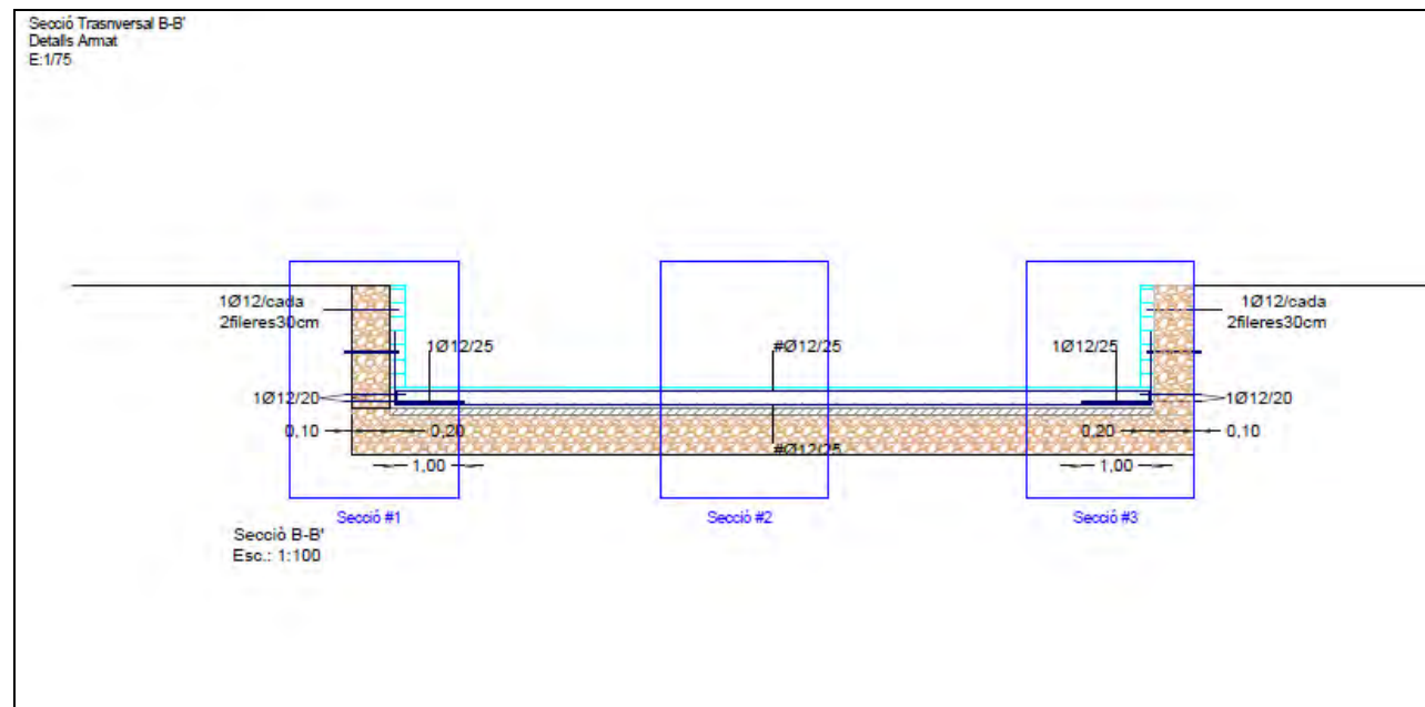
Figura núm. 17 Secció Transversal Armat
