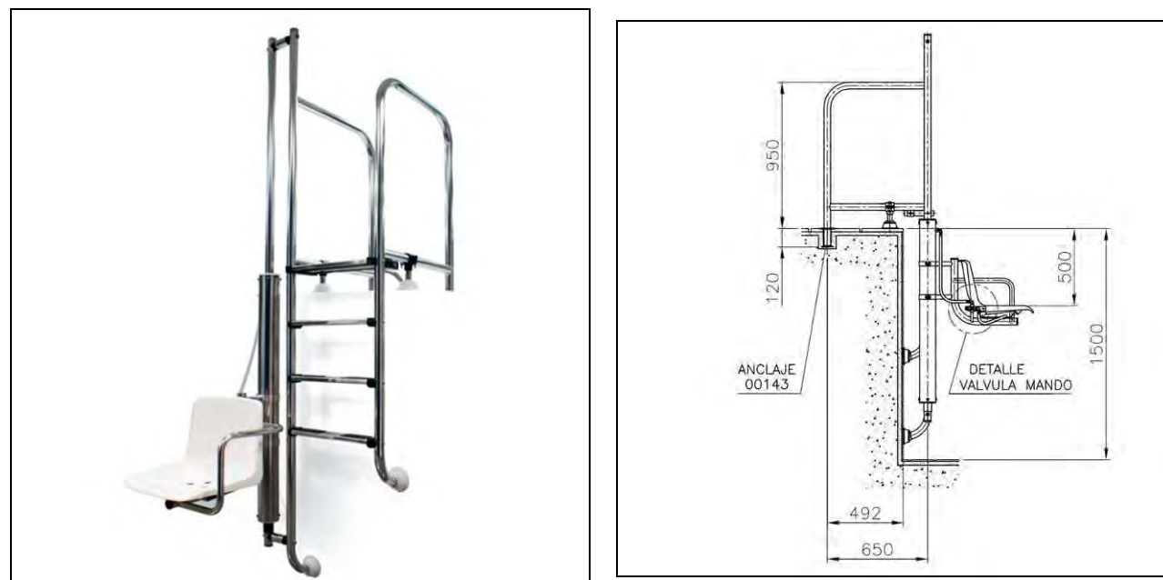
Figura núm. 21 Escala amb seient i elevador hidràulic per a minusvàlids.
