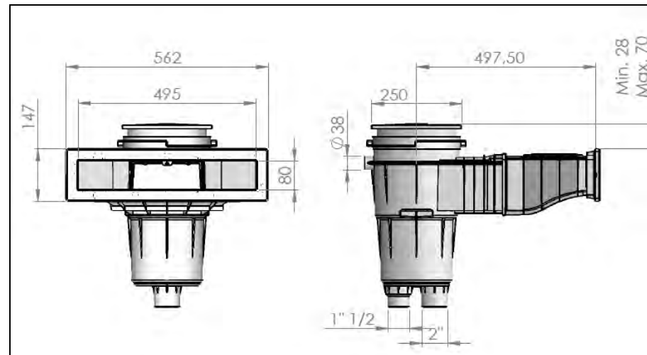
Figura núm. 19 Dimensions de perfil del Skimmer.
