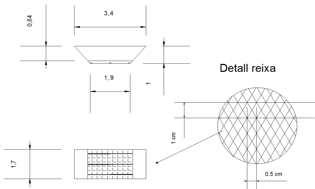
Imatge 1. Croquis tipus contenidor 5 m 3
