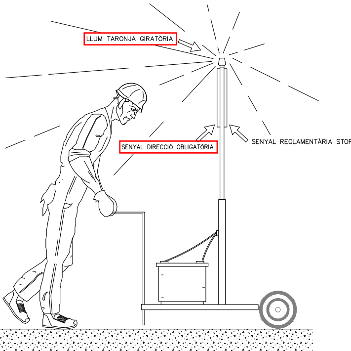
VISTA LATERAL
