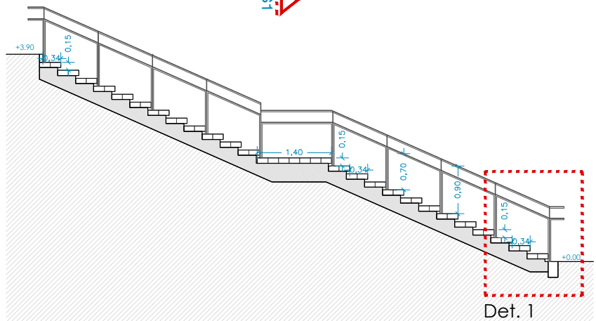
S1_SECCIÓ LONGITUDINAL
