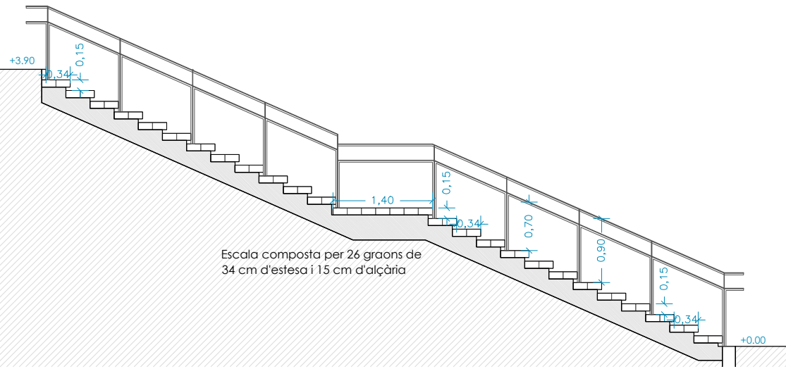
SECCIÓ LONGITUDINAL
