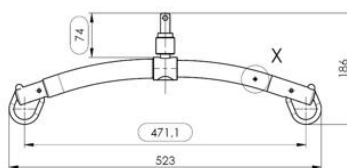
Mesures en mm de la Percha de 2 puntos / Ref: 015-02126
