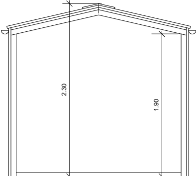
SECCIÓ A-B
