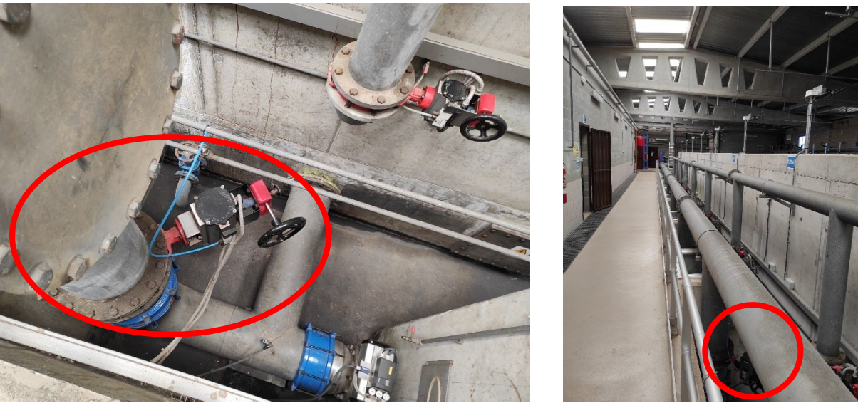
Figura 3. Vàlvula entrada aigua rentat
