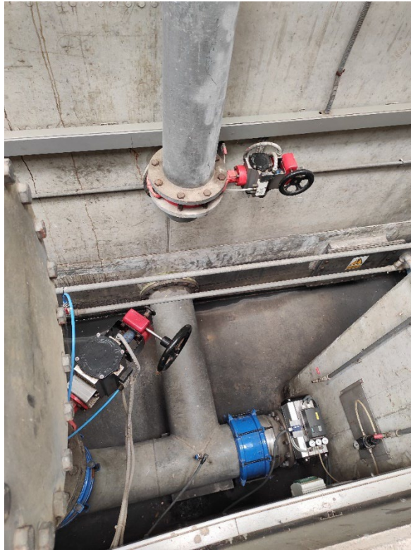
Fotografia 4. Vàlvules entrada aigua rentat i entrada aire rentat dels filtres
