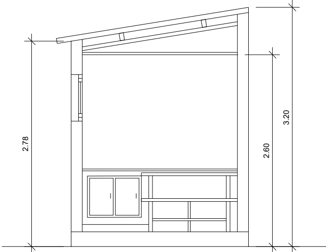
SECCIÓ A-B
