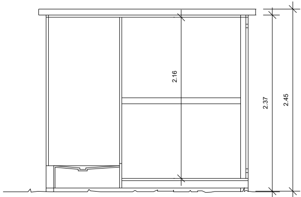
SECCIÓ A-B
