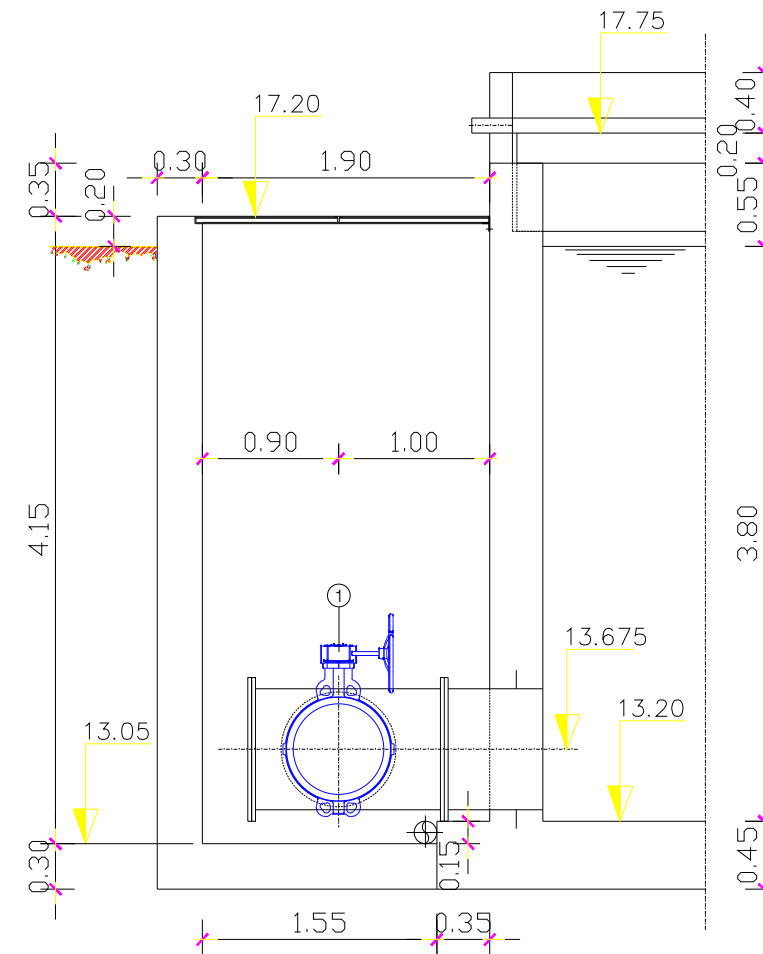
SECCIÓ B-B
