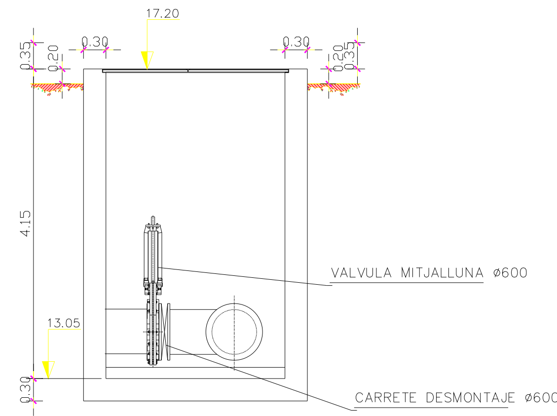
SECCIÓ A-A
