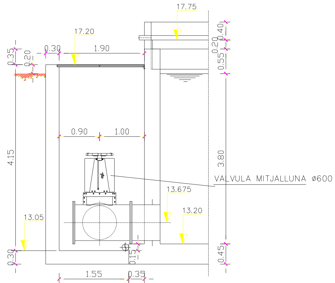
SECCIÓ B-B
