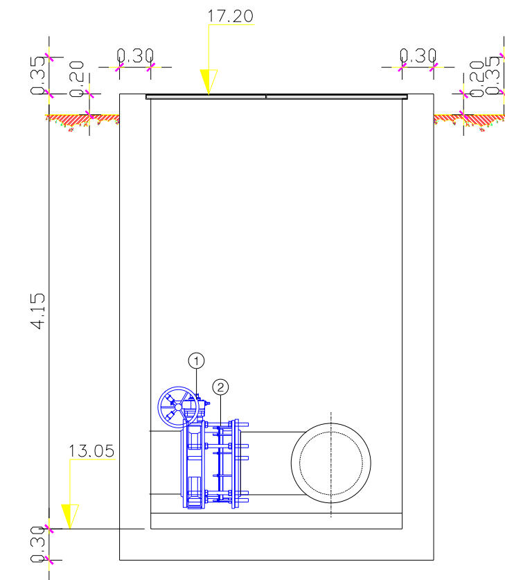
SECCIÓ A-A
