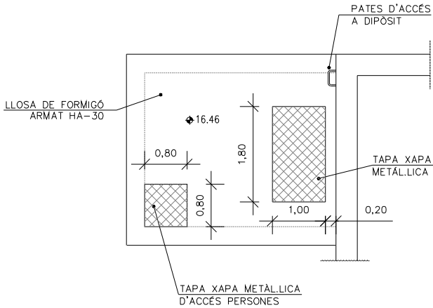
PLANTA COBERTA CASETA CLAUS SORTIDA ESCALA 1:100
