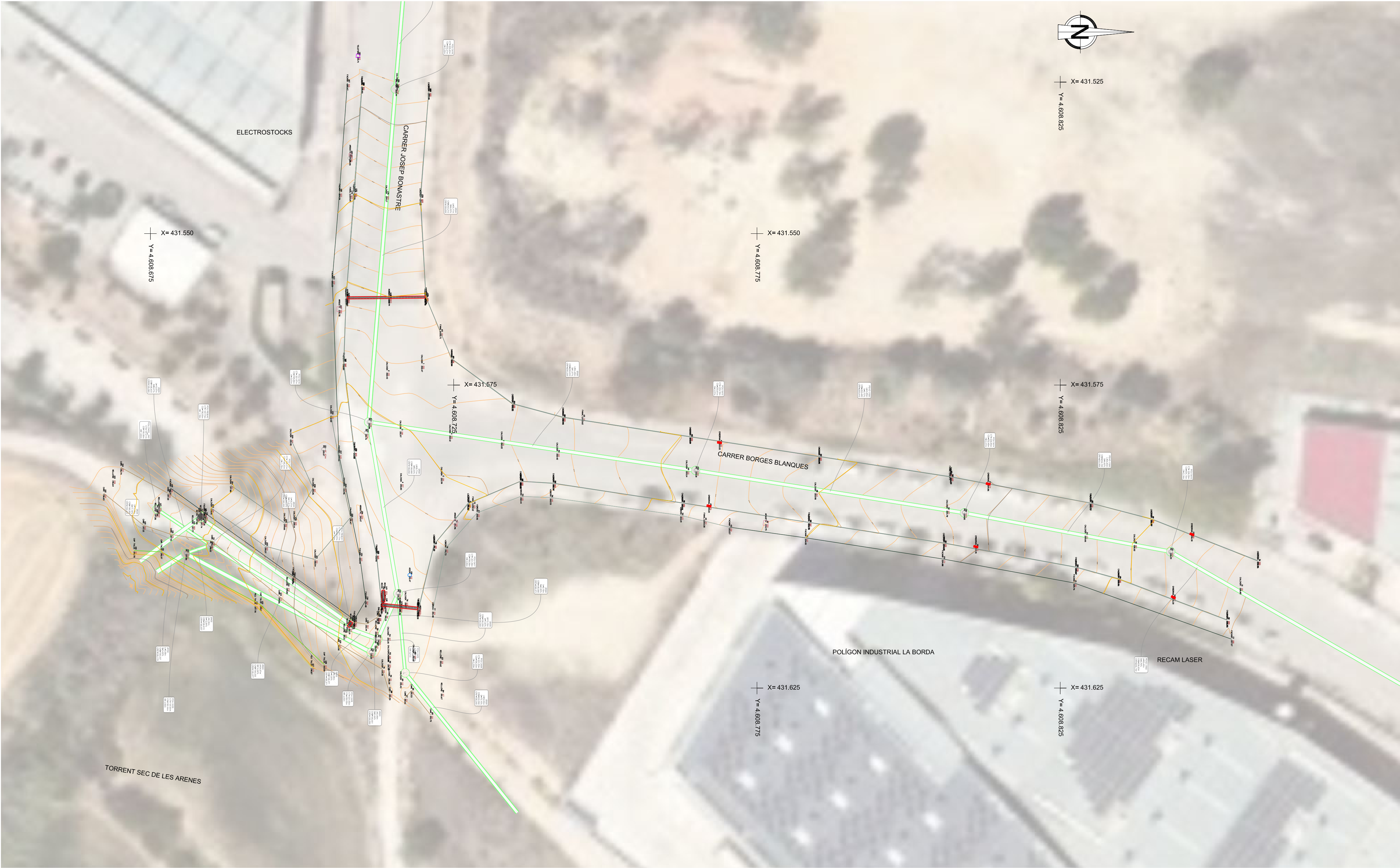
CLAVEGUERAM ESTAT ACTUAL PLANTA GENERAL escala 1:400
