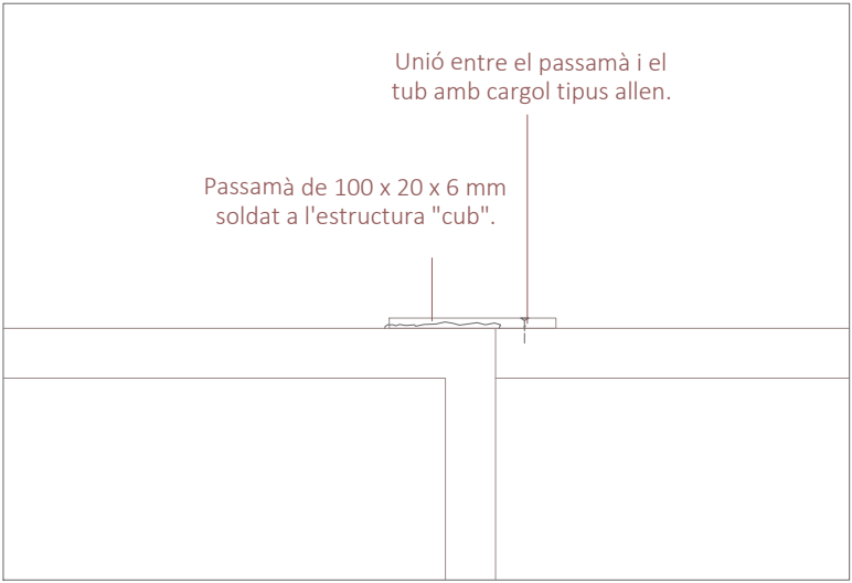
UNIONS ENTRE ESTRUCTURA CÚBICA I TUBS A3 1:5
