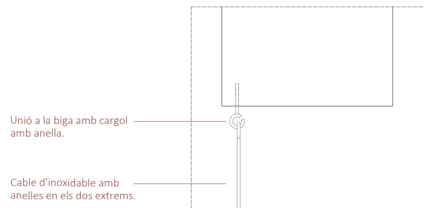
UNIÓ CABLE - BIGA 1:5
