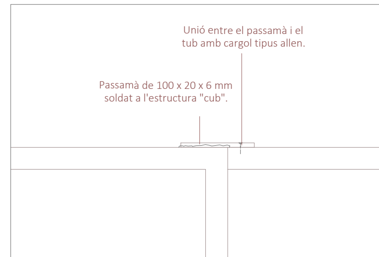
UNIONS ENTRE ESTRUCTURA CÚBICA I TUBS A3 1:5
