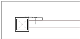
UNIONS PLAFÓ DE MDF I ESTRUCTURA TUBULAR A3 1:5
