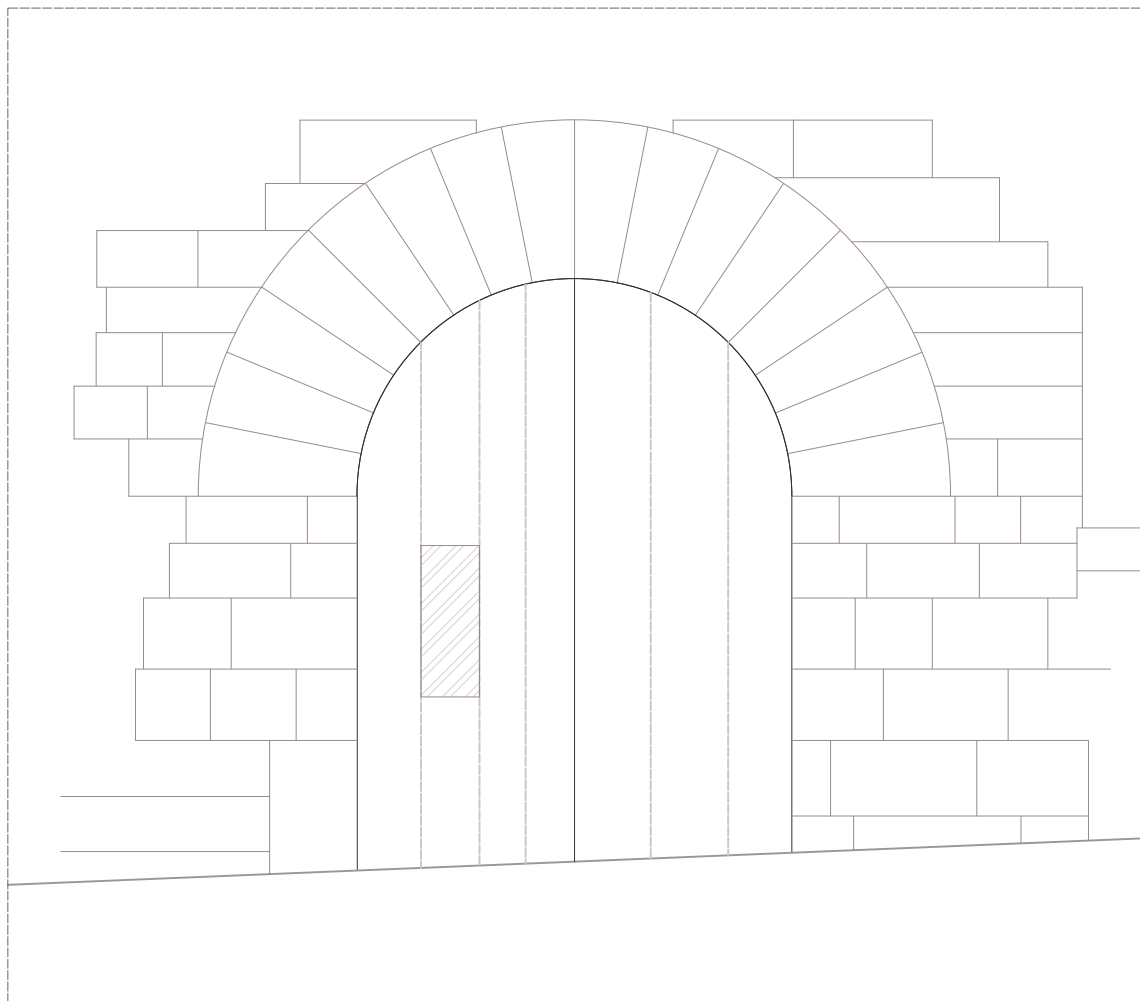
PORTA D'ENTRADA A3 1:20
