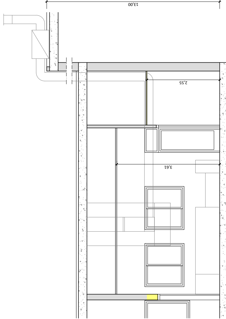
Secció esc. 1/50
