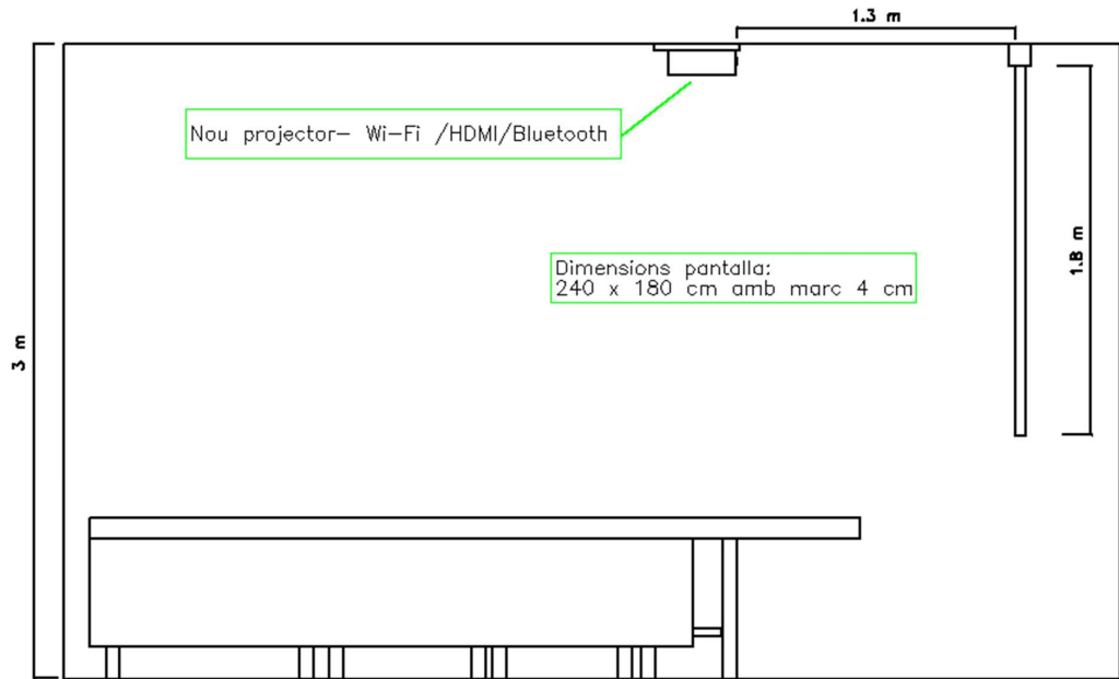
Il·lustració 18 Instal·lació del projectors
