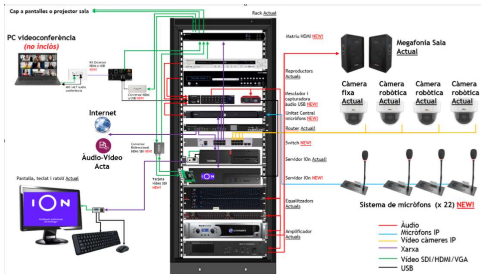
Il·lustració 13 Esquema de la solució a implementar
