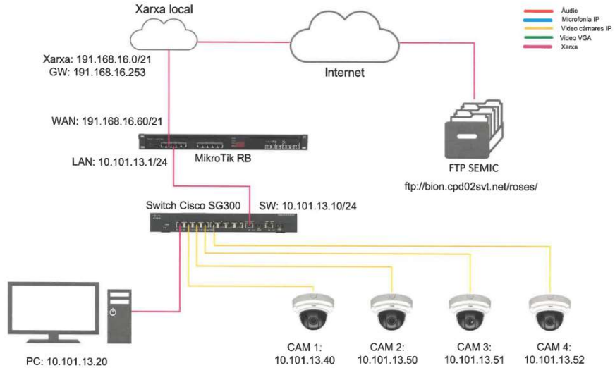
II-lustració 3 Esquema de xarxa
