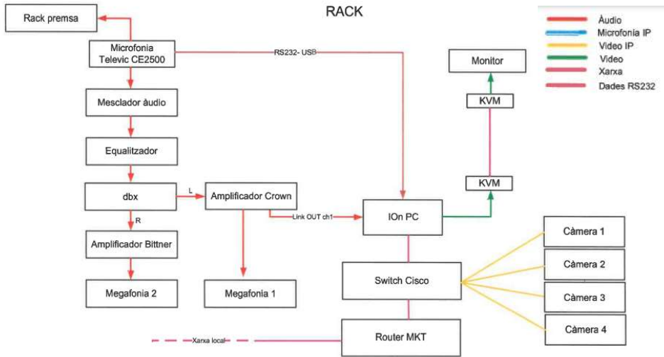
II-lustració 4 Esquema lògic
