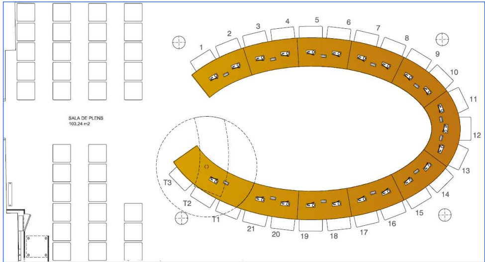
Il·lustració 10 Actualització de la numeració dels seients
