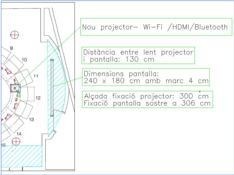
Il·lustració 12 Ubicació projector
