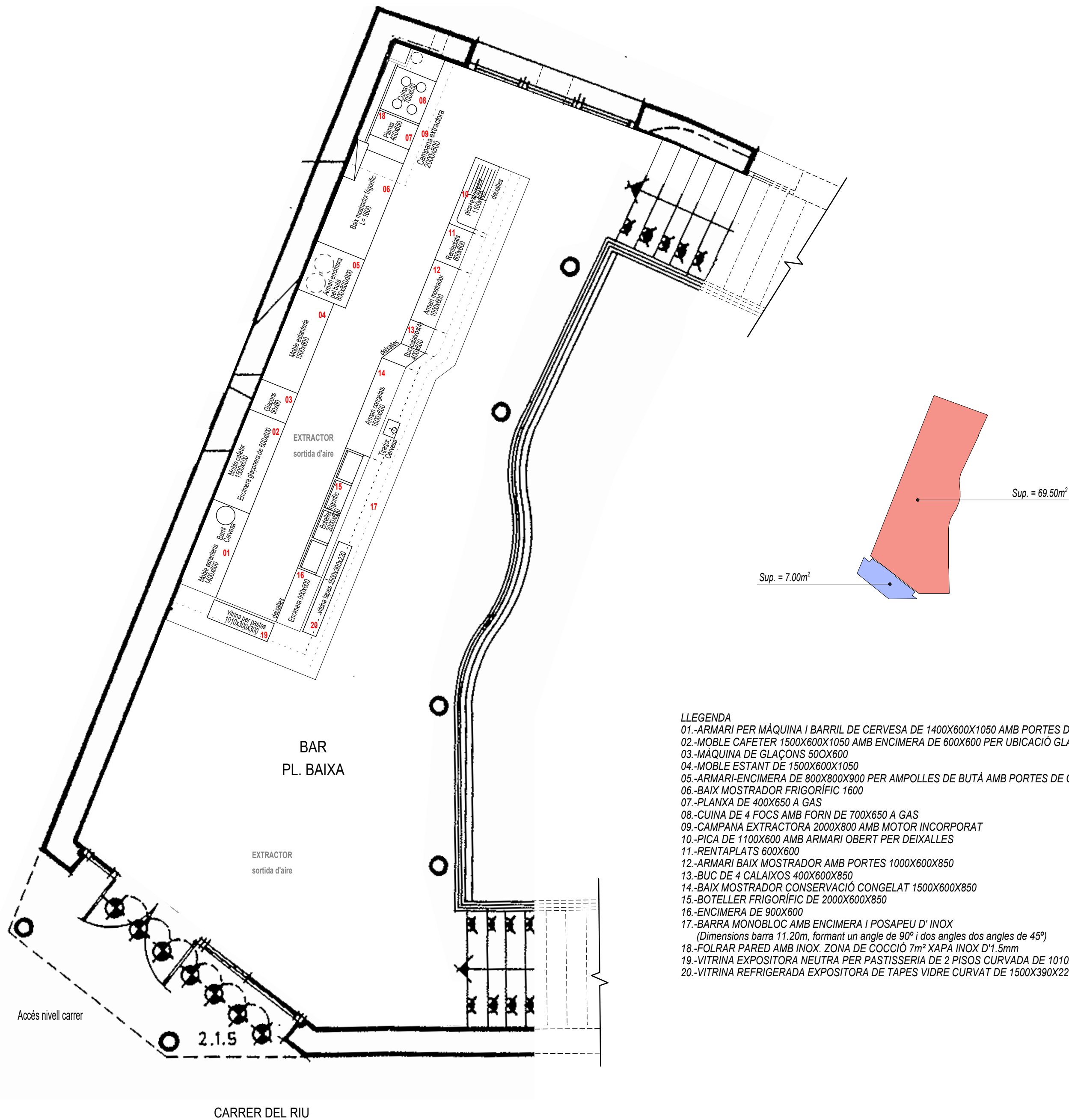
PLANTA BAIXA Esc.: 1:50 Sup. Bar 73m² (69.50m² + (50% * 7.00m²terrasa))
