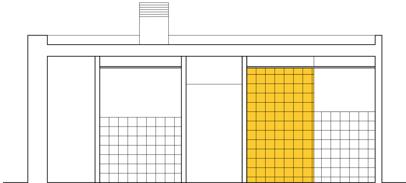
secció b-b'
