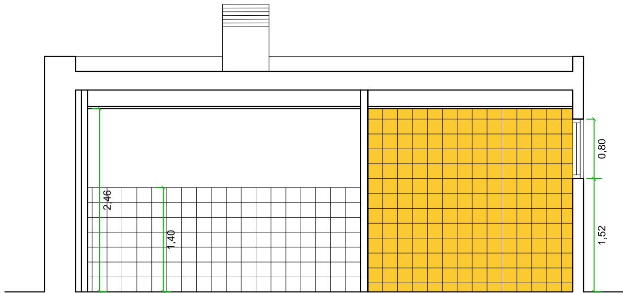
secció a-a'
