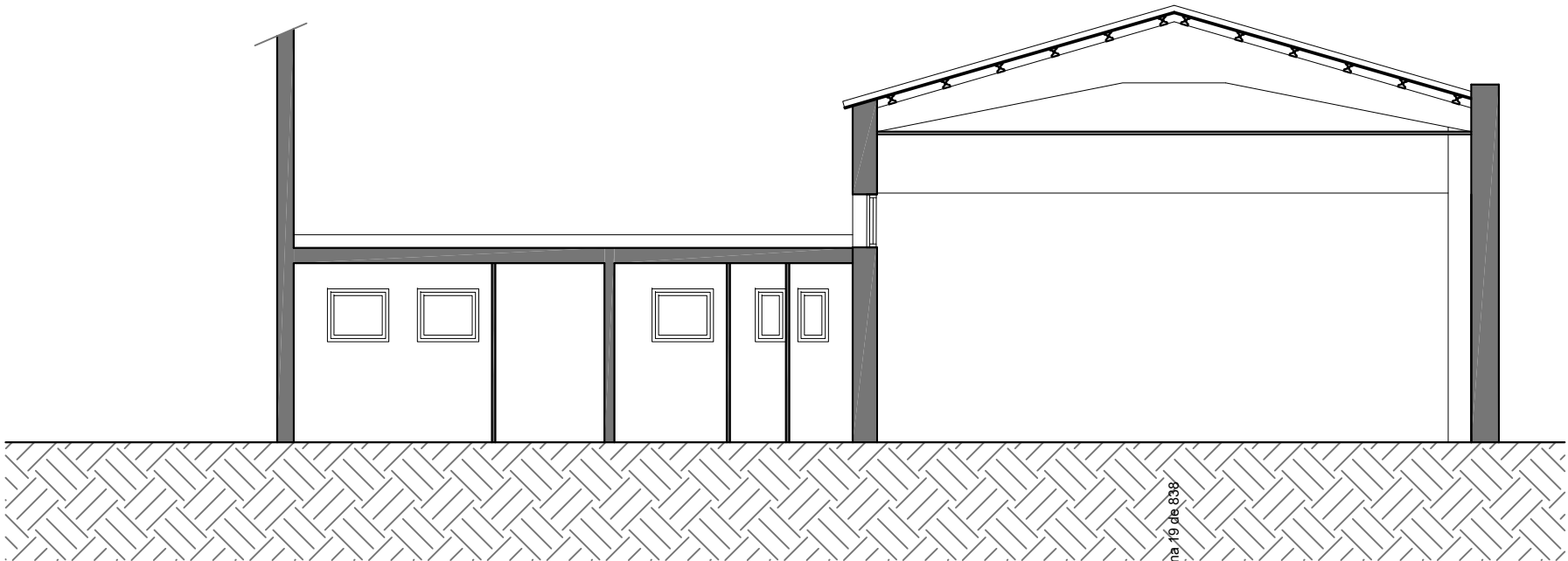
estat actual secció transversal, e 1/100
