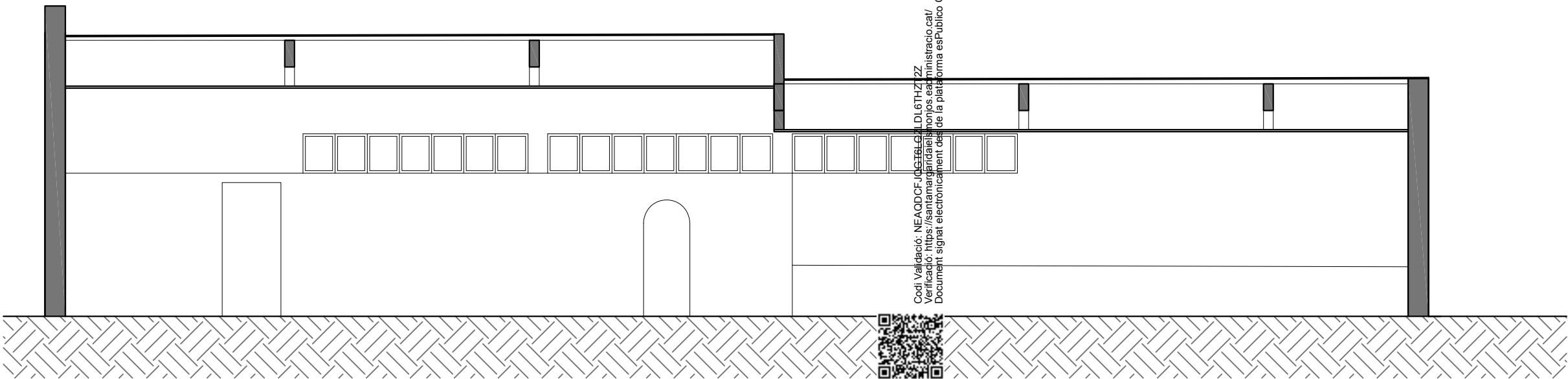
estat actual secció longitudinal, e 1/100
