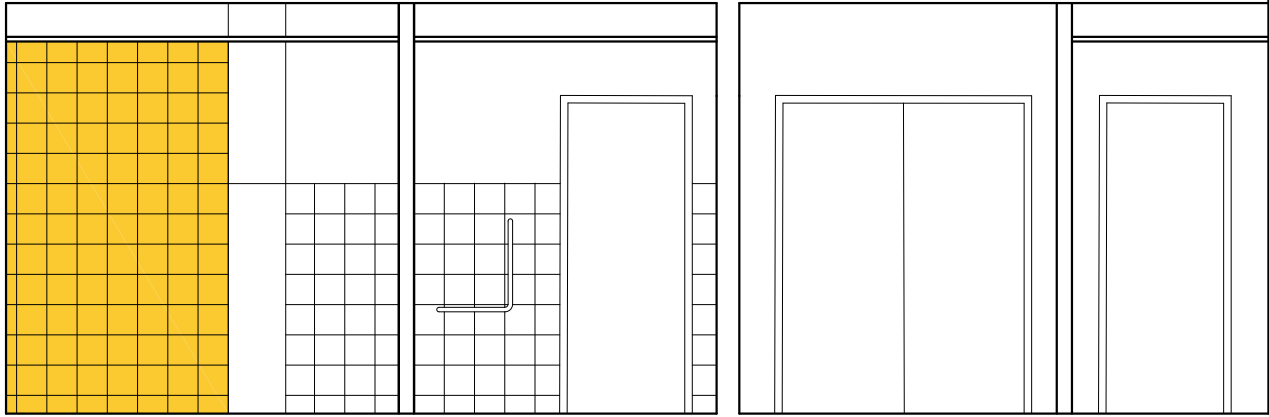
secció h-h'
