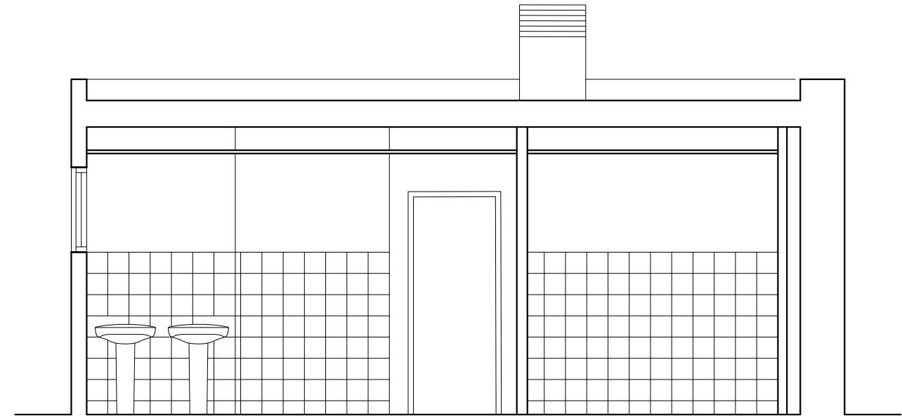
secció e-e'
