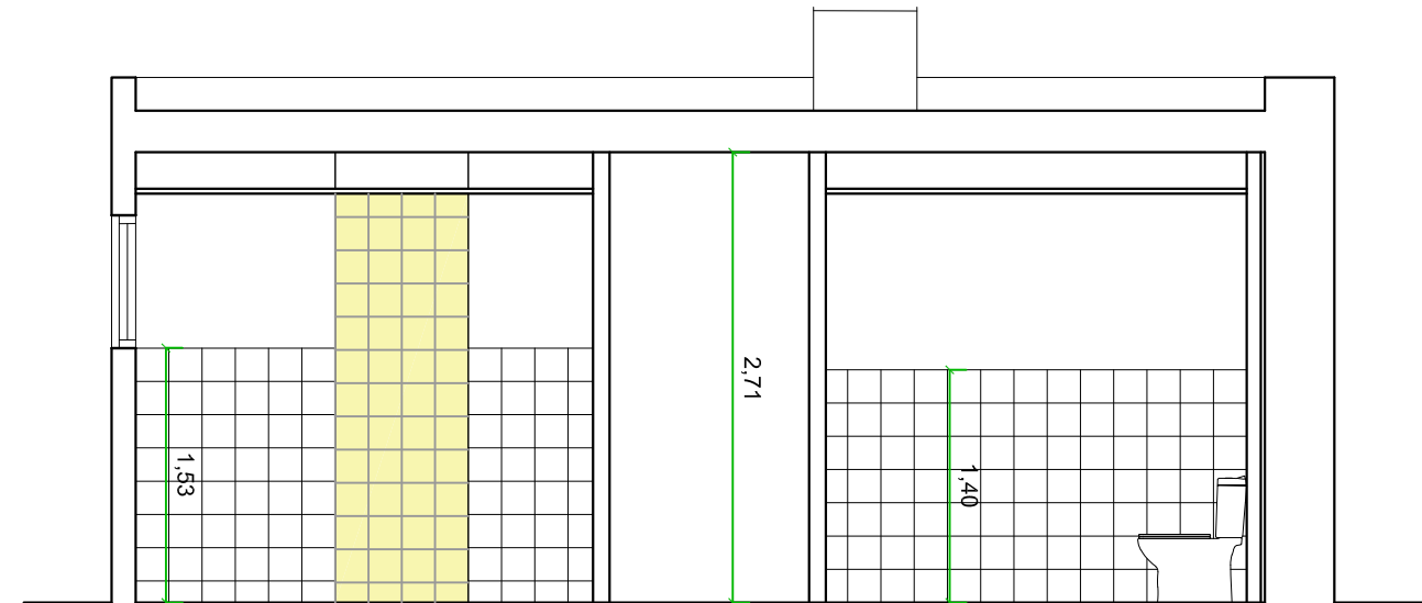
secció f-f''
