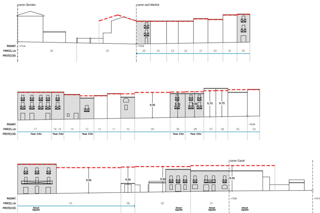
Plànol O.28 Alçat Illa 06332
