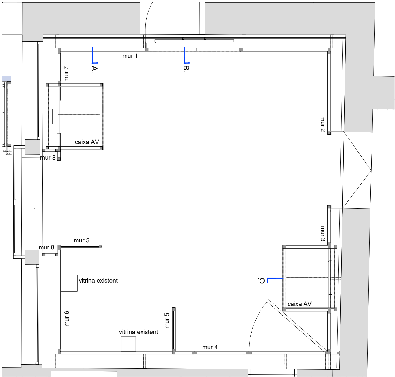
PLANTA SALA PETITA
