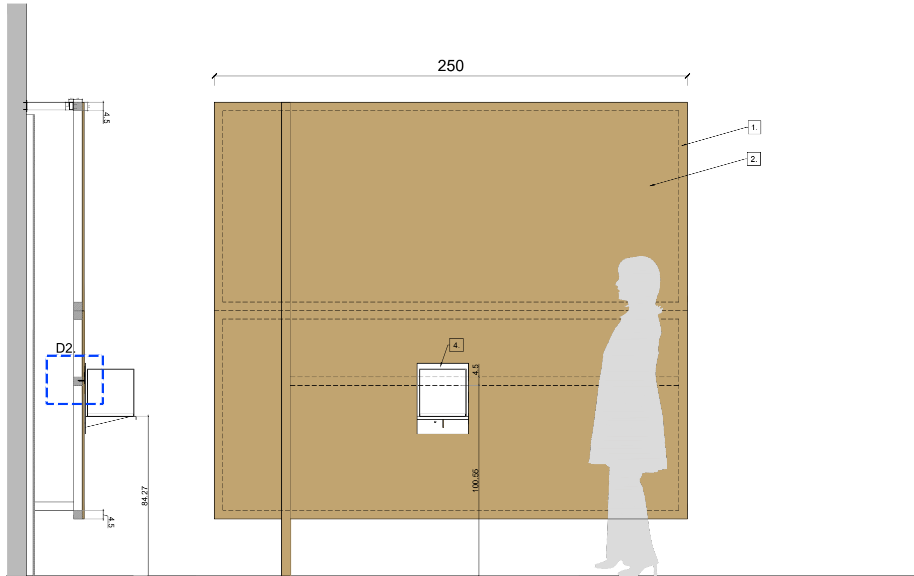
ALÇAT. E. 1/20
