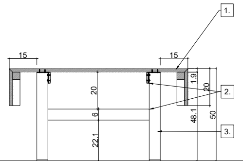
SECCIÓ A. E.1/20
