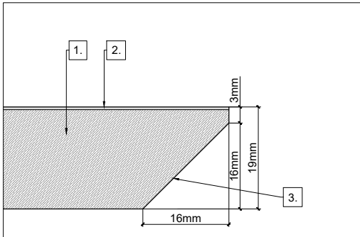
DETALL BISELL TIPUS A.
