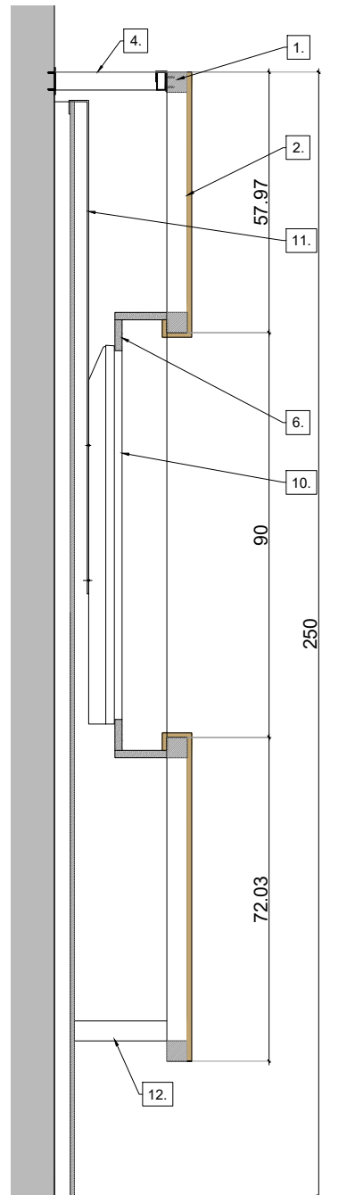
SECCIÓ B. E.1/15
