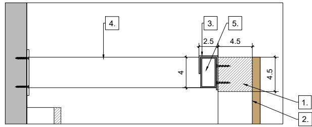
DETALL 1. E.1/5
