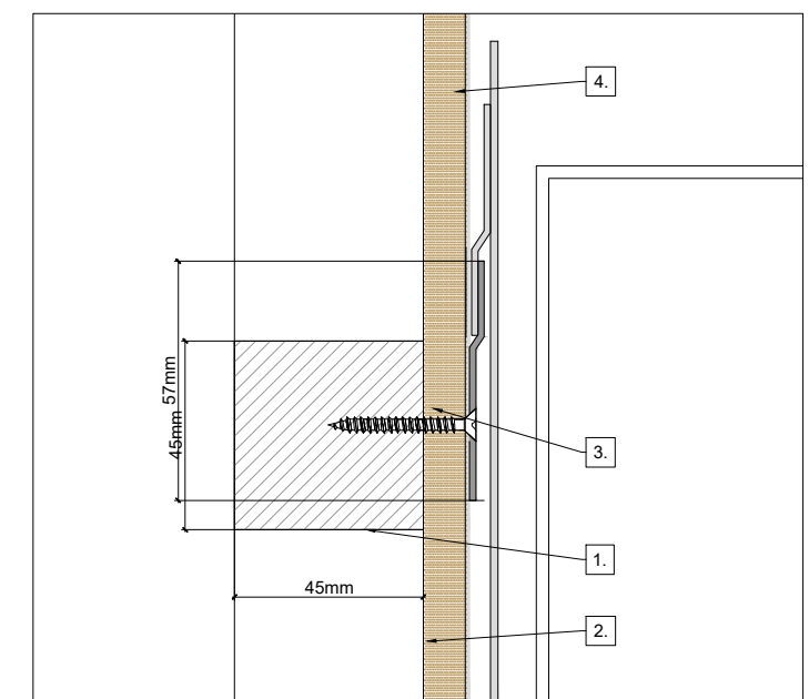
DETALL 2. E. 1/2
