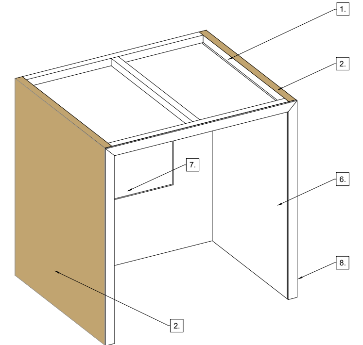
AXO CAIXES AV
