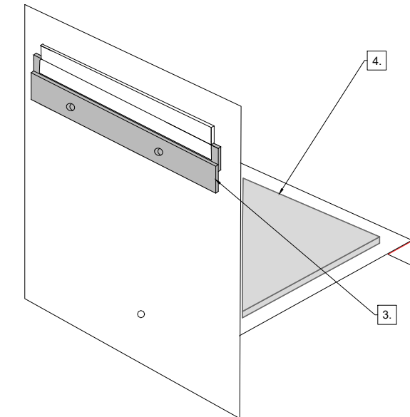
AXONOMETRIA SUBJECCIÓ VITRINA
