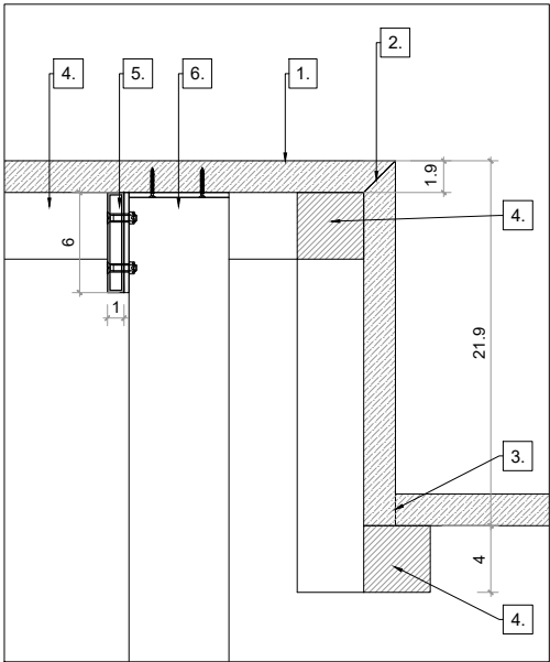
DETALL B. UNIÓ 90°. E. 1/5
