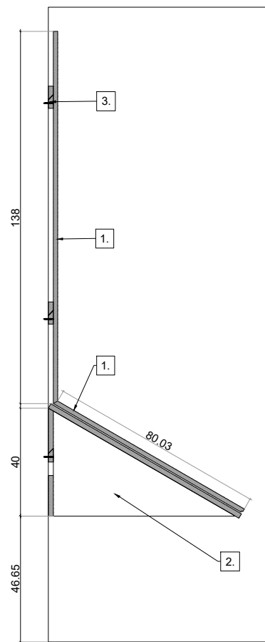
SECCIÓ 1.
