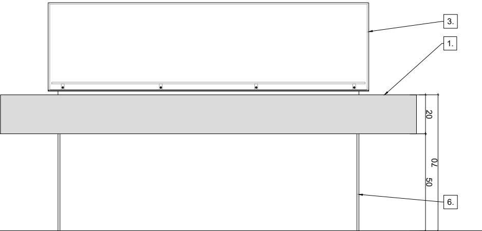
ALÇAT. E.1/20
