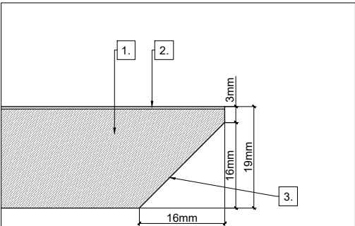
DETALL BISELL TIPUS A. E. 1/1
