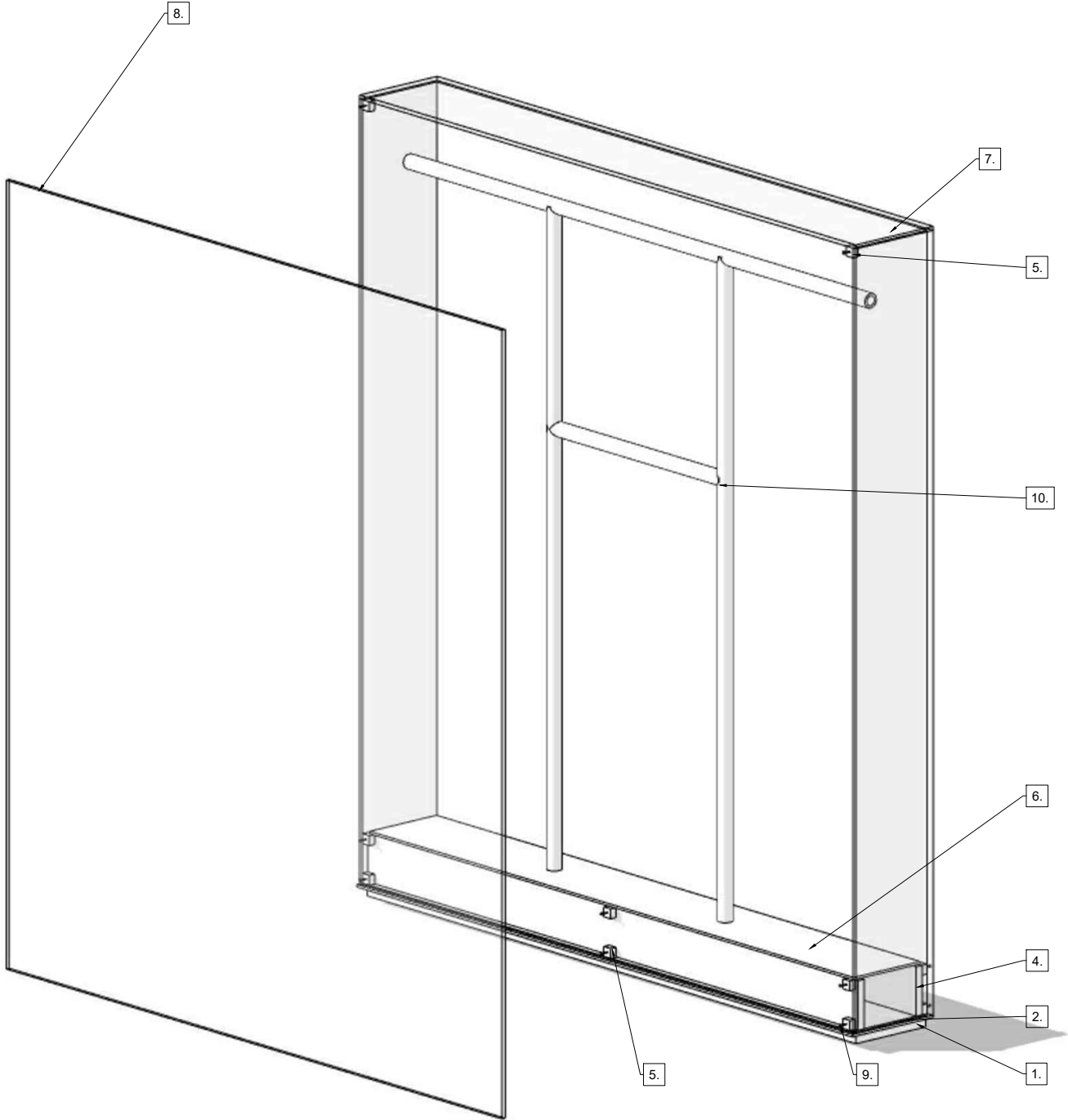
AXONOMETRIA VITRINA VESTITS. S/E
