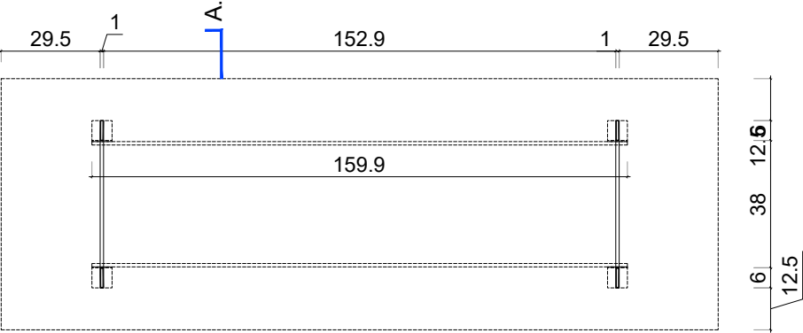
PLANTA ESTRUCTURA POTES. E.1/30
