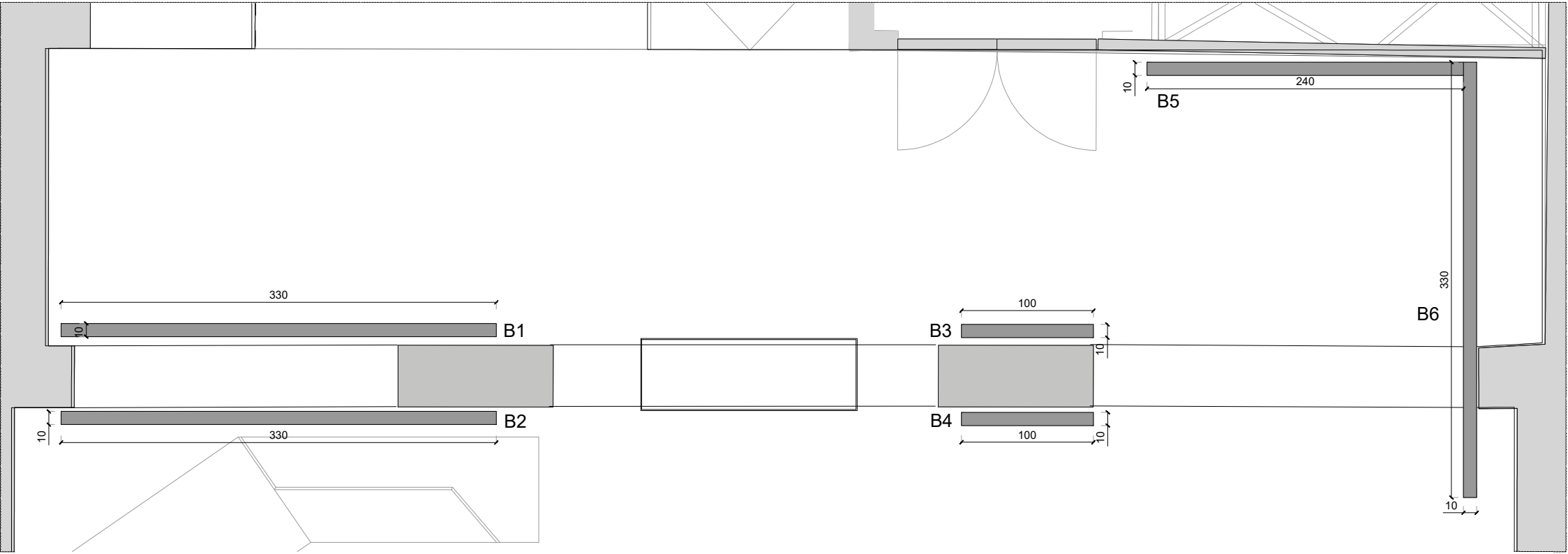
PLANTA. E. 1/40
