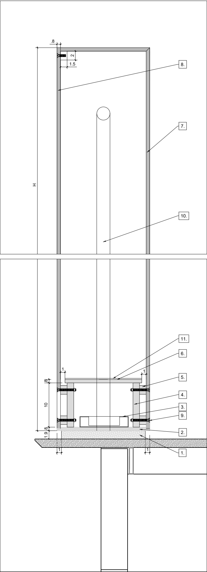
SECCIÓ 1
