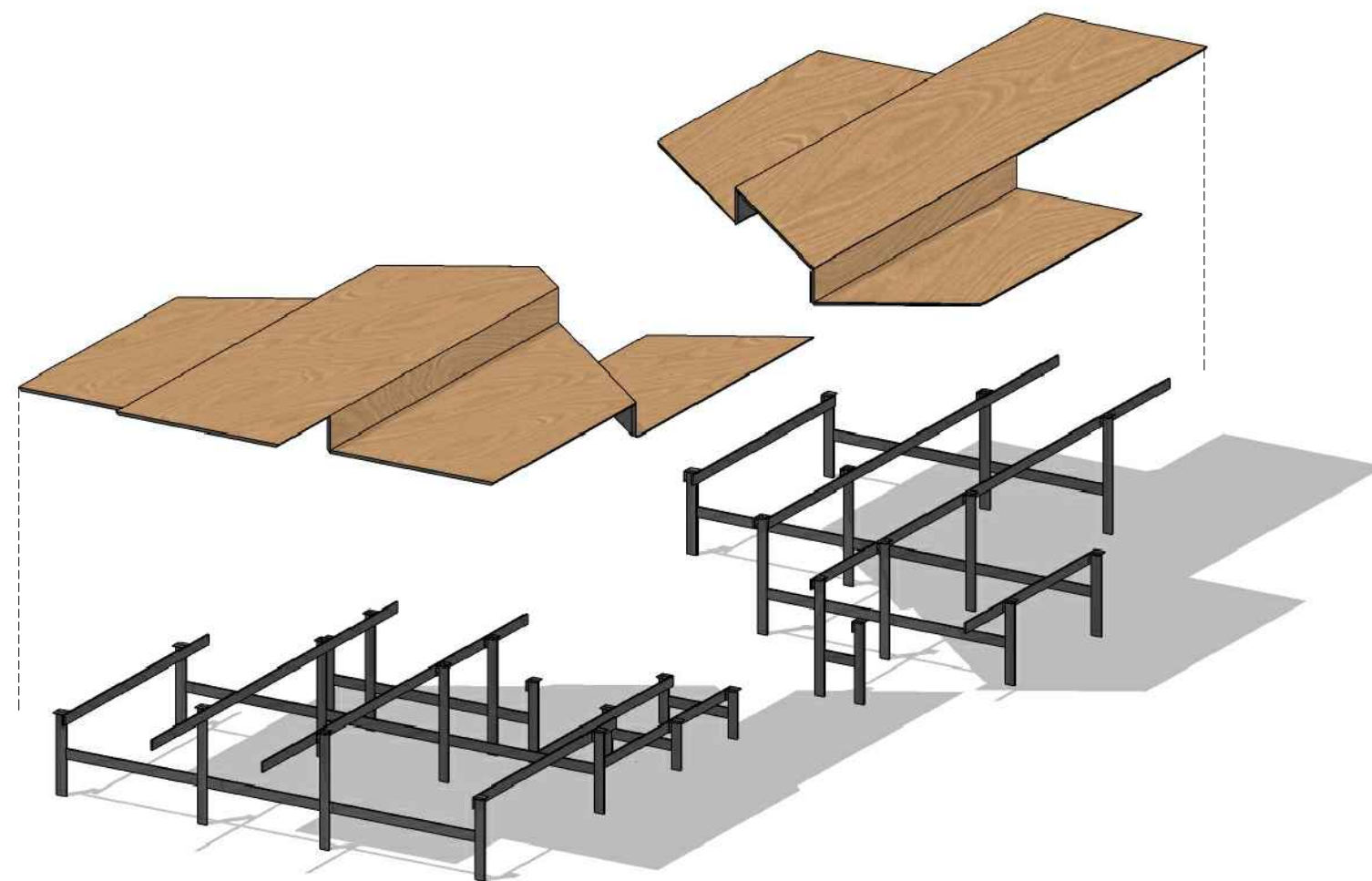
AXONOMETRIA POTES METÀL·LQUES + TAULA DE FUSTA
