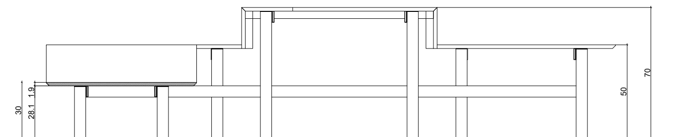
SECCIÓ B.
