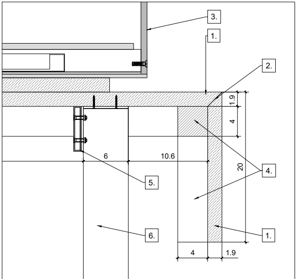
DETALL UNIÓ A 90°
