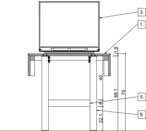
SECCIÓ A. E.1/20
