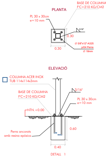
Pergola fonament 1 : 50
