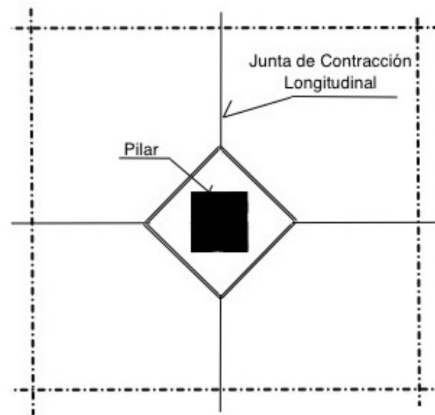
Esquema junts de pilar en soleres
