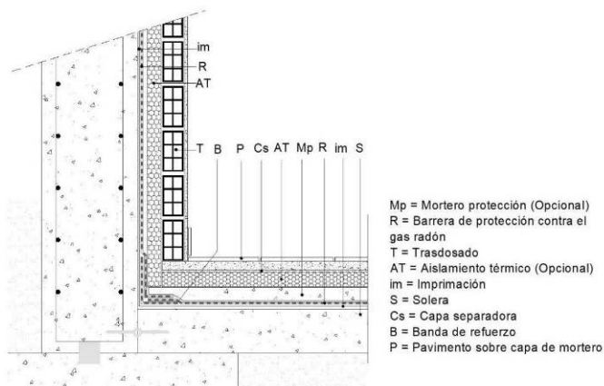
Fig. 7. Solera con sistema de despresurización lineal Easi-Sump y barrera de protección contra el radón.
