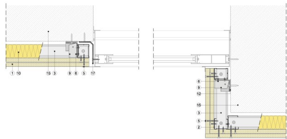
Sección horizontal
