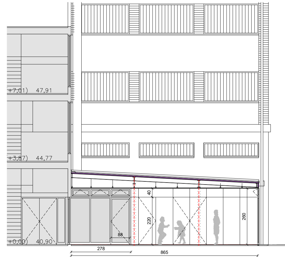
SECCIÓ LONGITUDINAL 2
