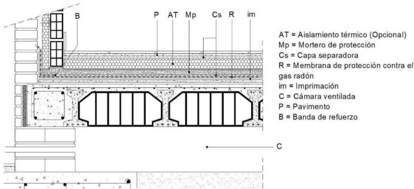
Fig. 5. Suelo elevado: forjado ventilado y barrera de protección contra el radón. Sistema monocapa adherido.
