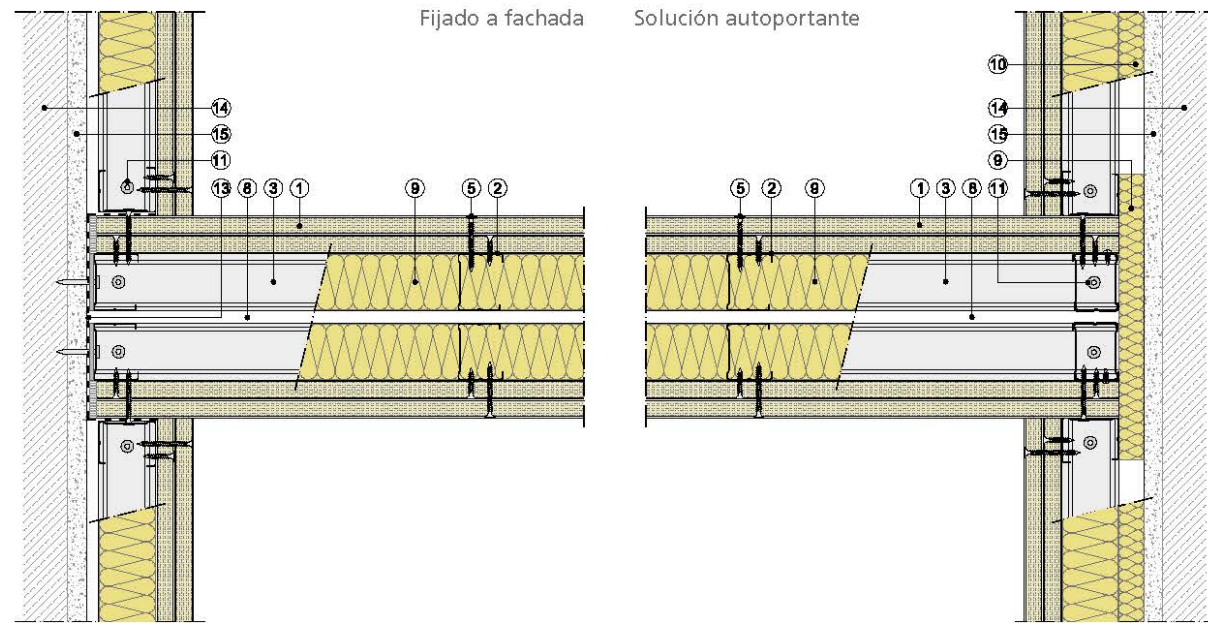
Sección horizontal
