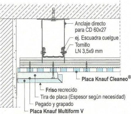
D127.es-SO6 Friso recrecido con junta en sombra adicional
