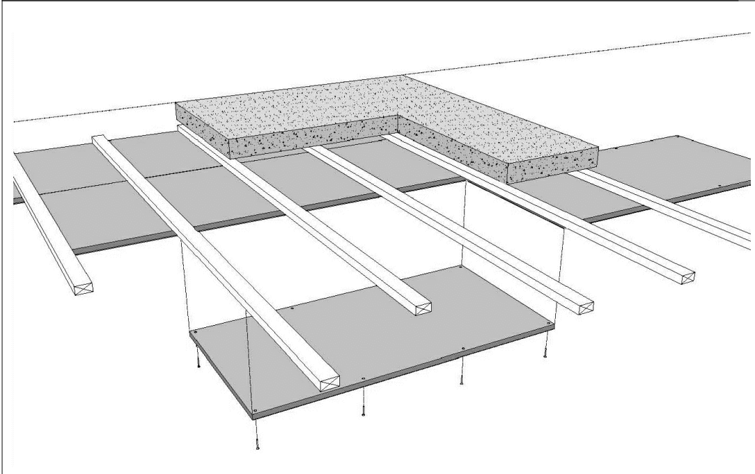
D3. DETALL CELRAS FONOABSORBENT. SISTEMA
