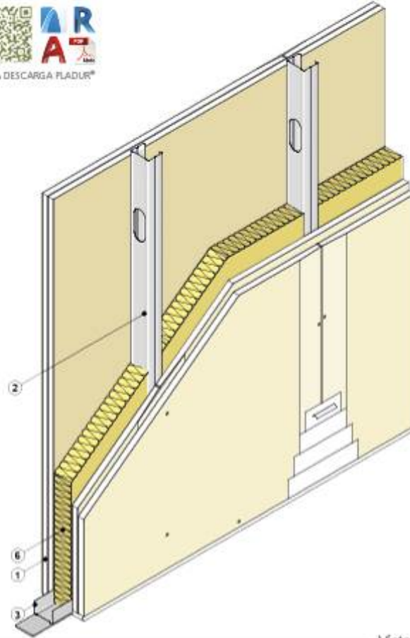
Vista isométrica
