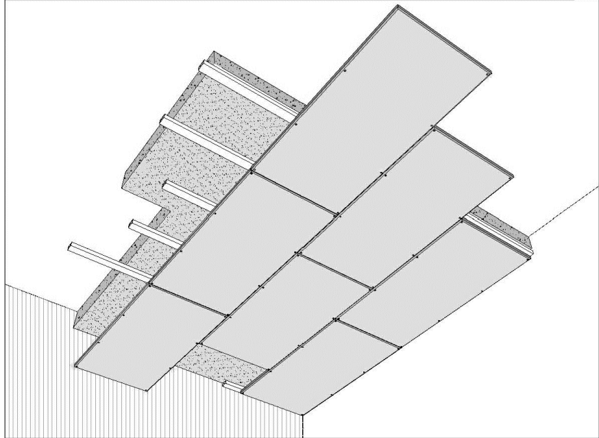
D1. DETALL CELRAS FONOABSORBENT. SISTEMA
