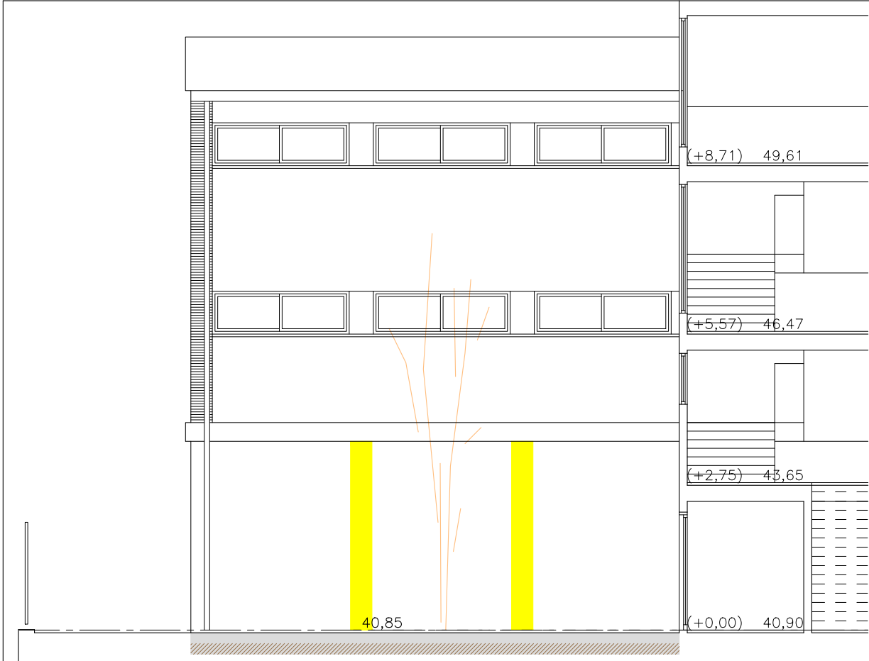
SECCIÓ L1
