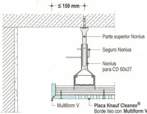
D127.es-SO7 Techo foseado
