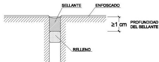
Figura 2.6 Ejemplo de junta de dilatación
