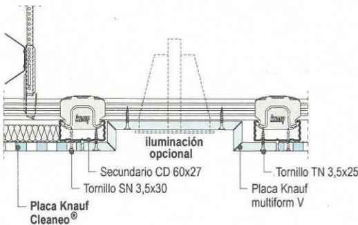
D127.es-SO4 Foseado. Iluminación integrada
