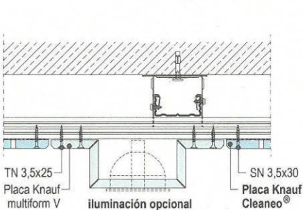
D127.es-SO5 Cajón. Iluminación integrada
