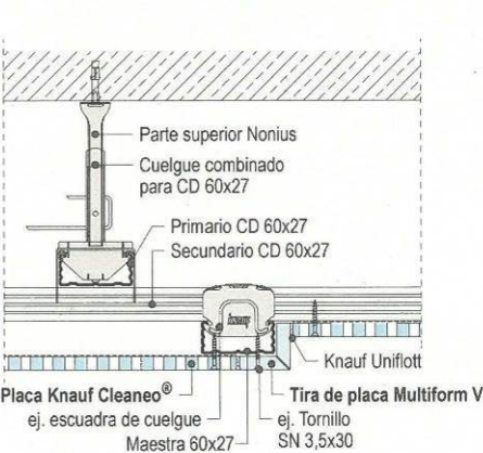
D127.es-SO3 Cambio de nivel de techo
