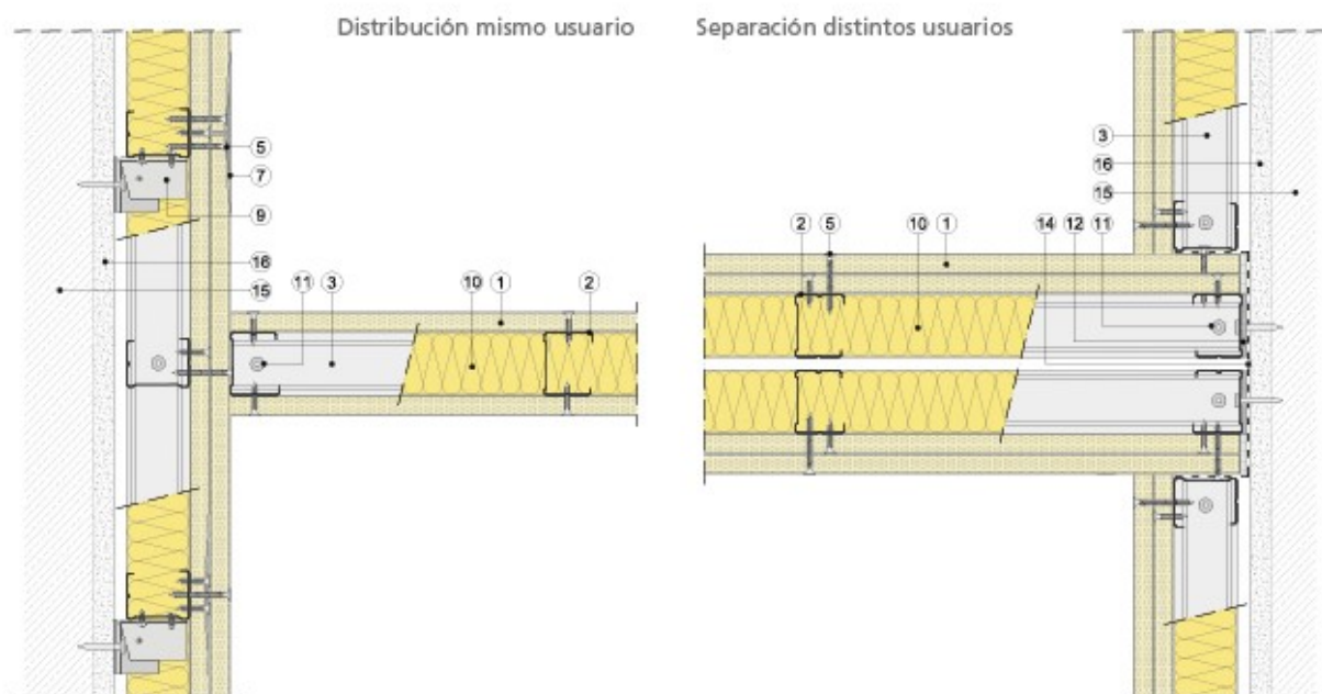
Sección horizontal
