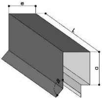
Coronación de albardilla CT
