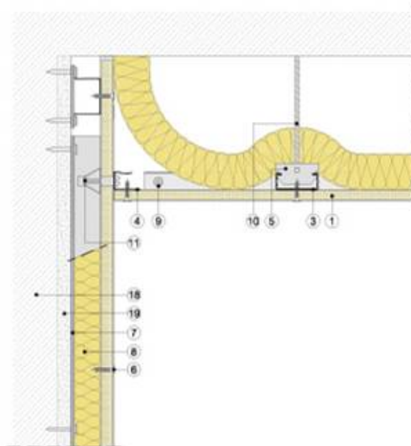
Sección vertical
