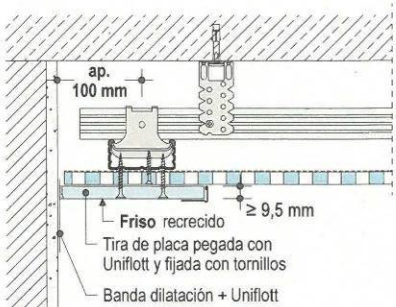
D127.es-D1 Friso - recrecido
