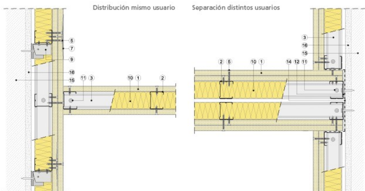
Sección horizontal
