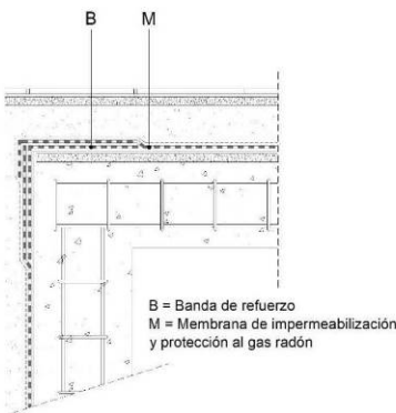
Fig. 8. Encuentro del muro con cubierta enterrada.
