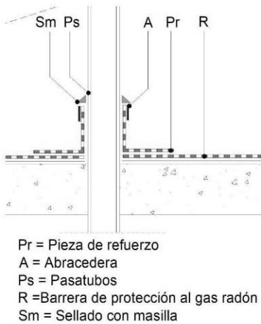
Fig. 11. Paso de conducto sin manguito (suelos). Protección de gas radón.
