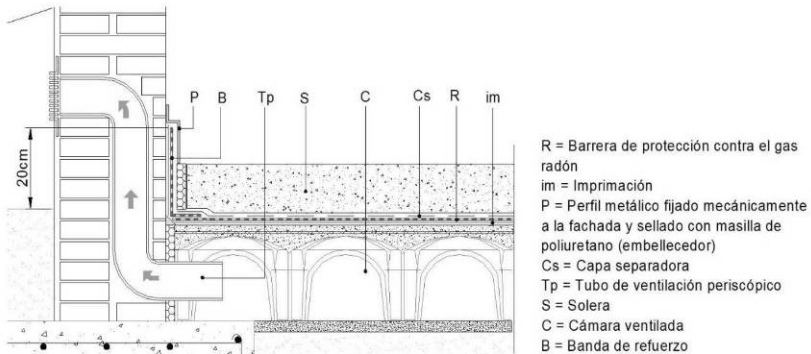
Fig. 6. Solera y muro con barrera de protección contra el radón por el interior. Sistema monocapa adherido. Caso de rehabilitación.
