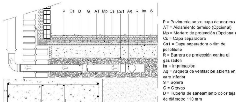
Fig. 7. Solera con sistema de despresurización lineal Easi-Sump y barrera de protección contra el radón.
