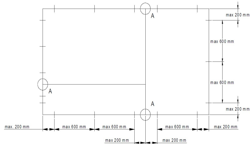
Figura 6. Posicionamiento de las fijaciones
