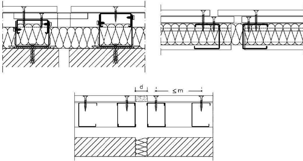
Figura 185 – Juntas de dilatación con perfilaría auxiliar
