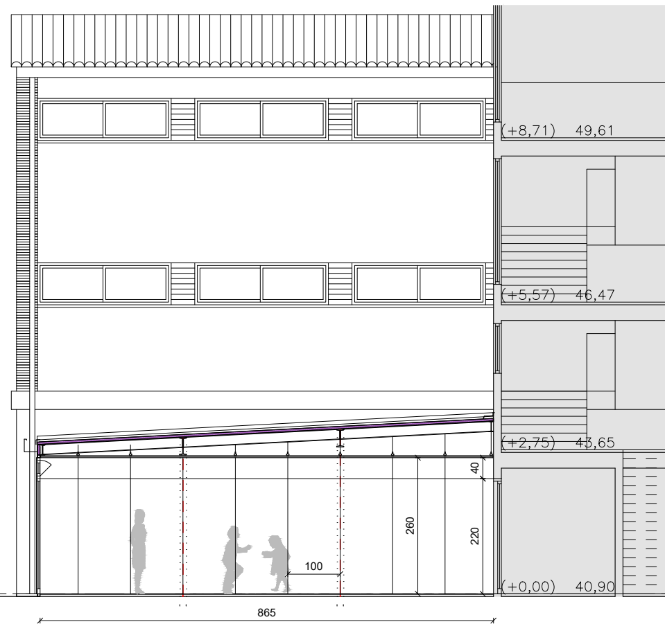
SECCIÓ LONGITUDINAL 1
