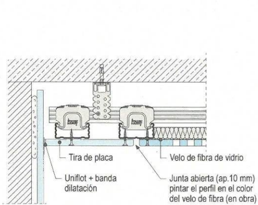
D127.es-D5 Friso con junta abierta
