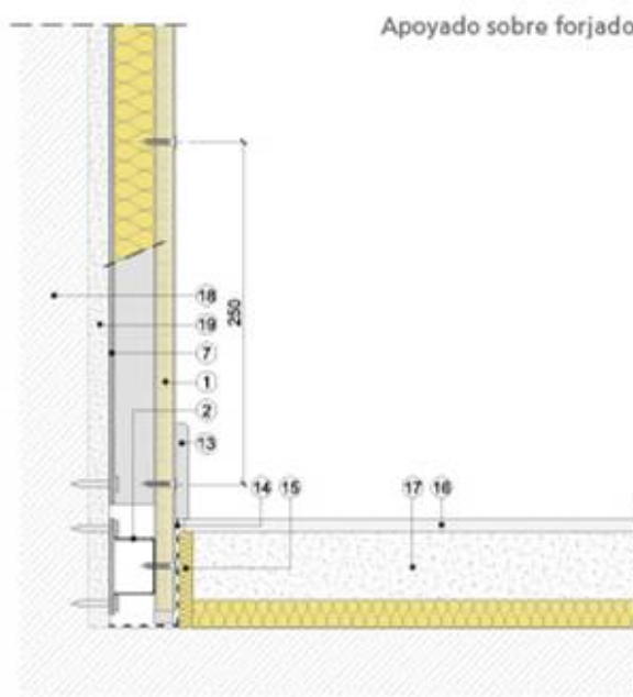
Sección vertical
