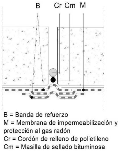
Fig. 12. Juntas de dilatación de muro vertical.
