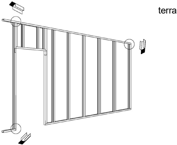
Figura 70 – Instal·lació de la banda estanca
