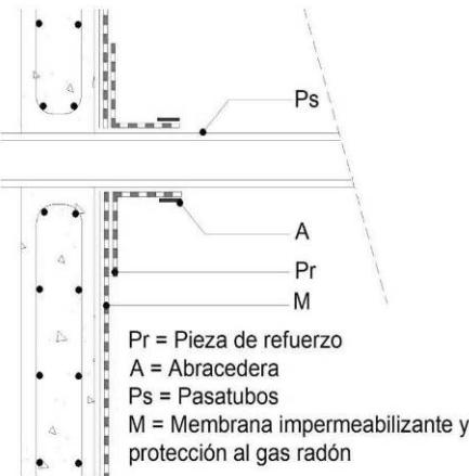
Fig. 10. Paso de conducto sin manguito (muros). Protección de gas radón.
