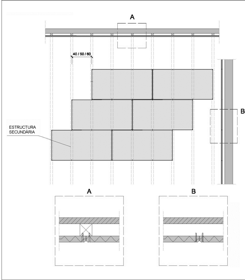
D2. DETALL CELRAS FONOABSORBENT. ESPECEJAMENT I ESTRUCTURA DE SUBJECCIÓ
