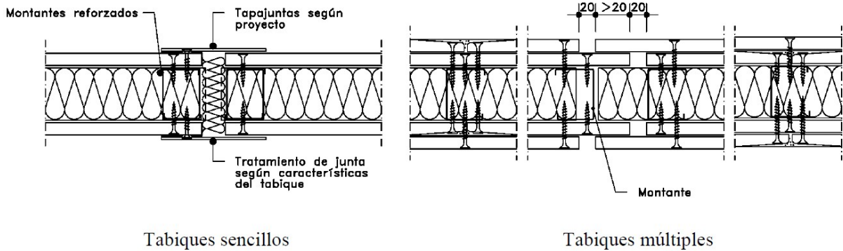
Figura 106 – Junta de dilatación
