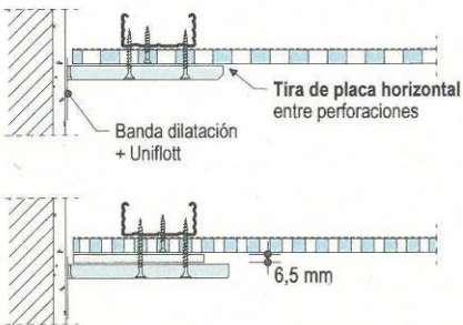
D127.es-SO7 Techo foseado
