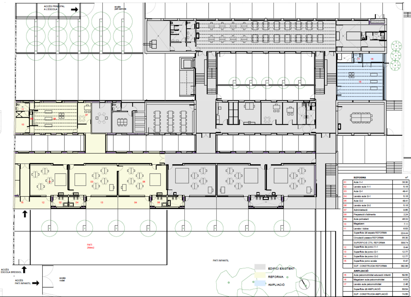
Planta Baixa
