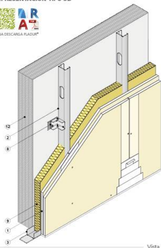
Vista isométrica
