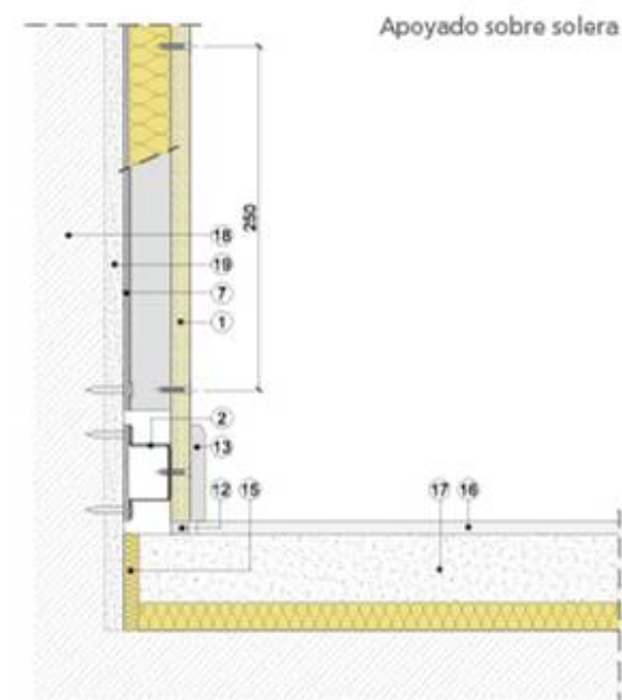
Sección vertical
