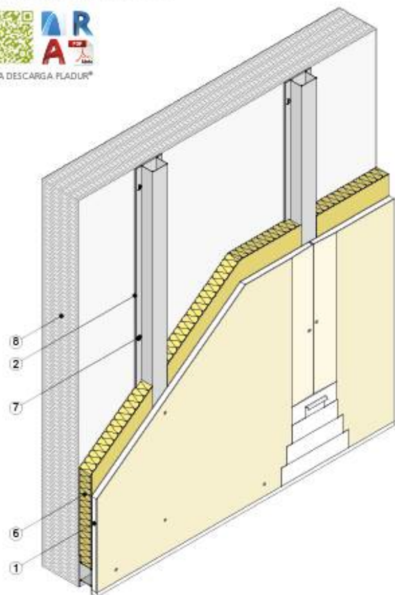
Vista isométrica
