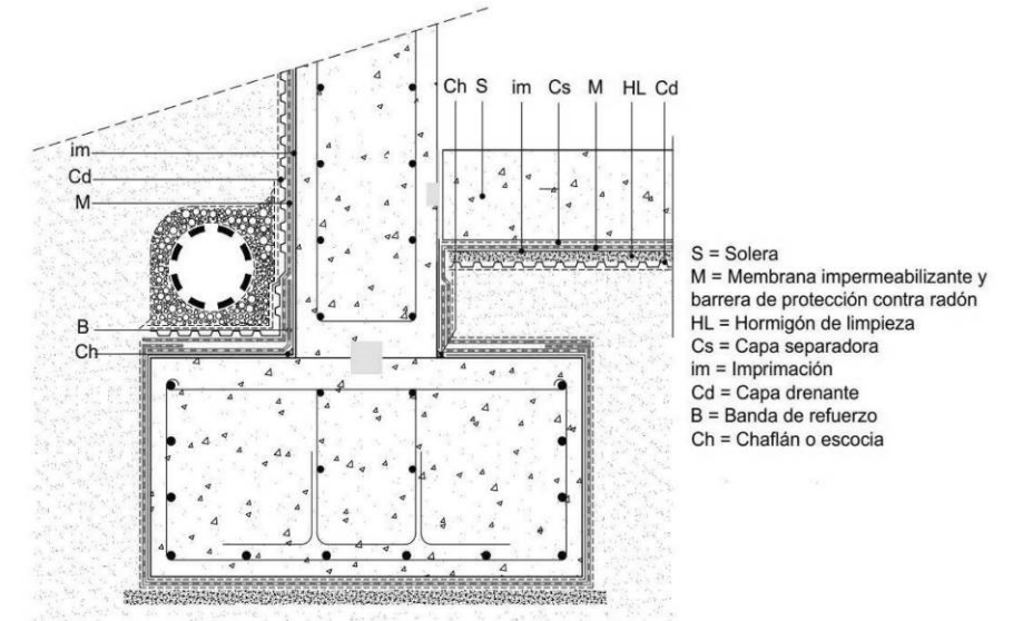
Fig. 2. Placa y muro con barrera de protección contra el radón e impermeabilización por el exterior. Sistema bicapa no adherido en placa y sistema monocapa adherido en muro
