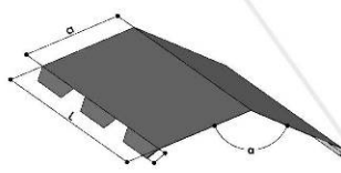
Cumbrera troquelada CT
