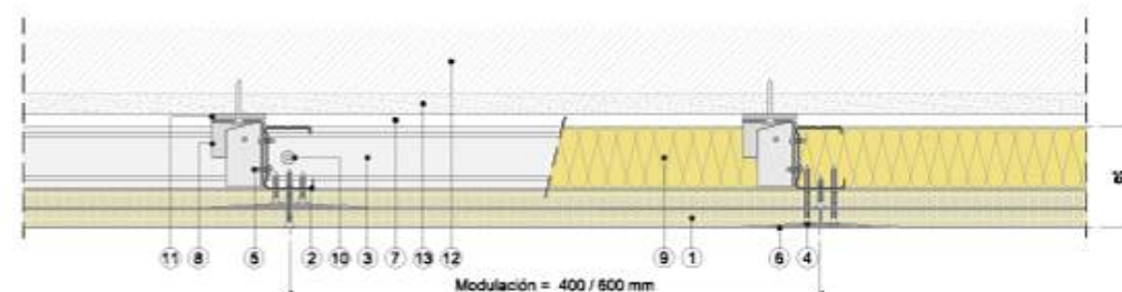
Sección horizontal
