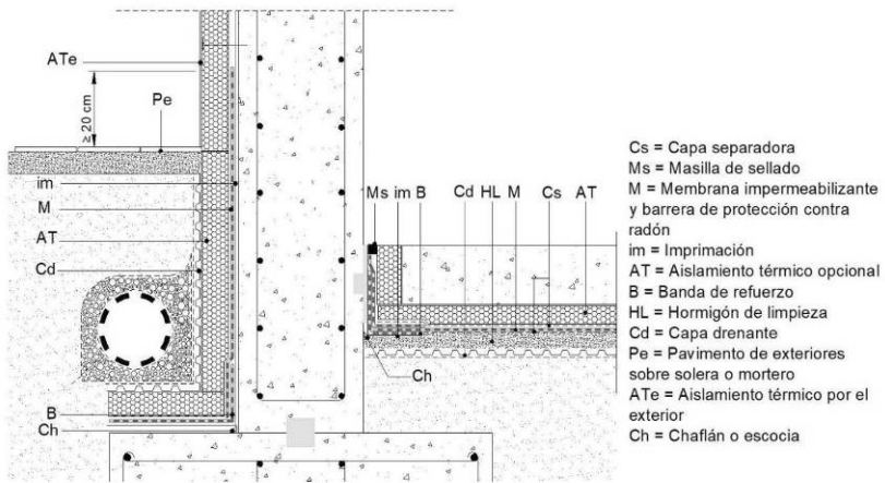
Fig. 4. Suelo elevado: forjado sanitario ventilado y barrera de protección contra el radón. Sistema monocapa adherido.
