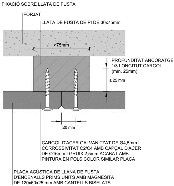
D4 DETALL FIXACIÓ
