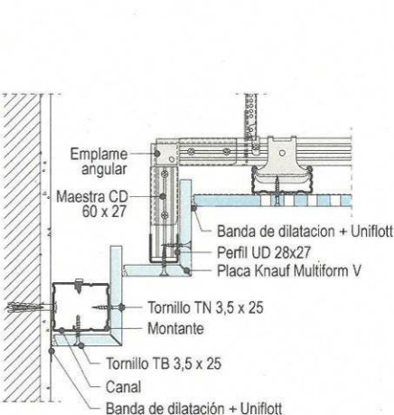
D127.es-SO2 Friso escalonado
