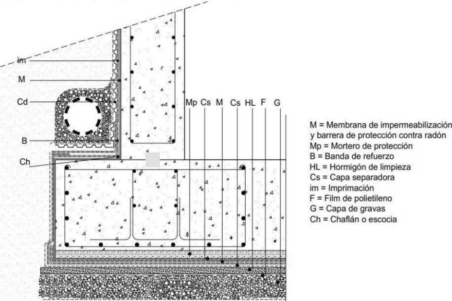
Fig. 2. Placa y muro con barrera de protección contra el radón e impermeabilización por el exterior. Sistema bicapa no adherido en placa y sistema monocapa adherido en muro
