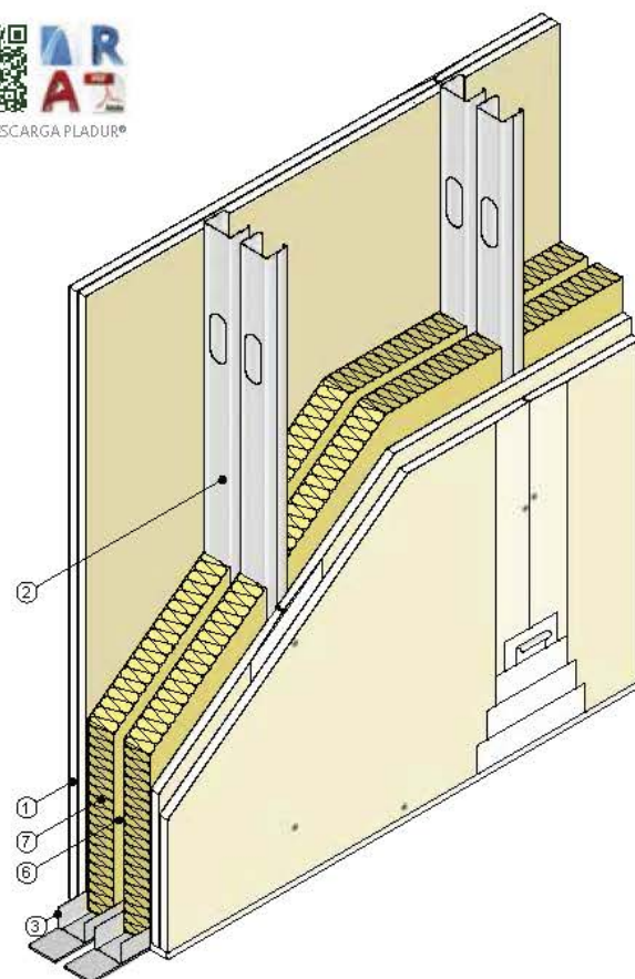
Vista isométrica
