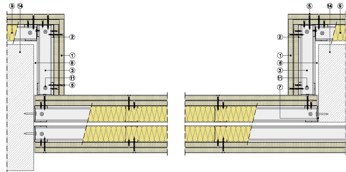
Sección horizontal
