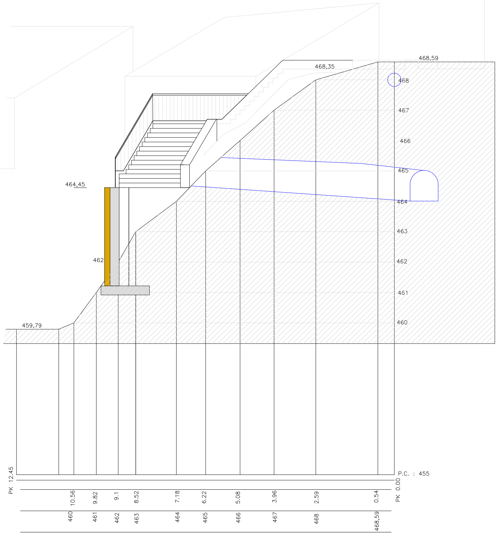
PERFIL LONGITUDINAL TERRENO ESCALA H=1:1000 V=1:1000
