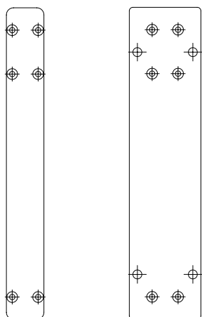
Tapa lateral i suport de paret. Alumini anoditzat, gruix 2mm.
