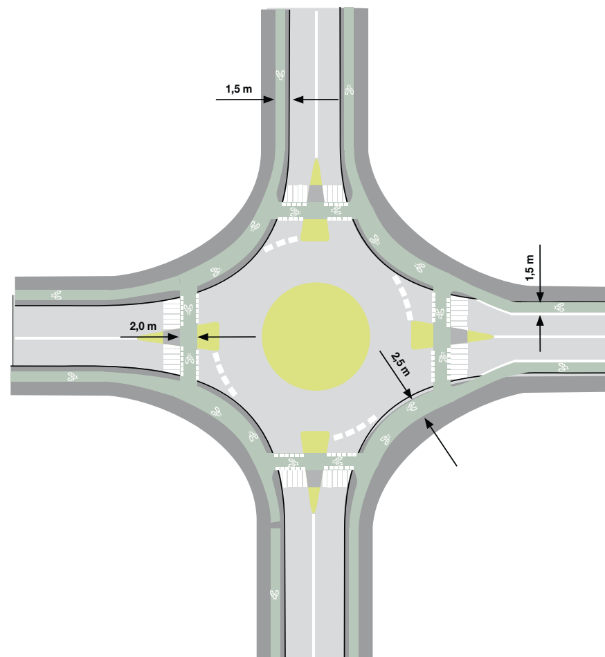
Figura 23.- Intersecció giratòria
