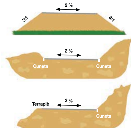
Figura 19.- Drenatge de vies ciclistes
