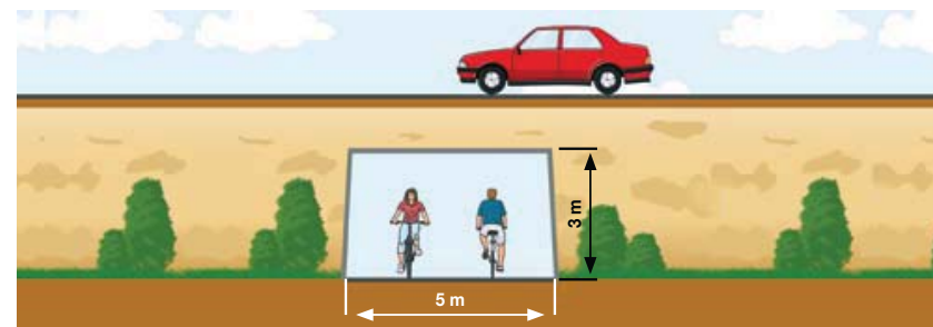
Figura 13.- Secció mínima en túnels de vies ciclistes
