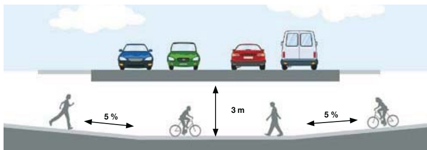
Figura 14.-Pas soterrat ciclistes/vianants
