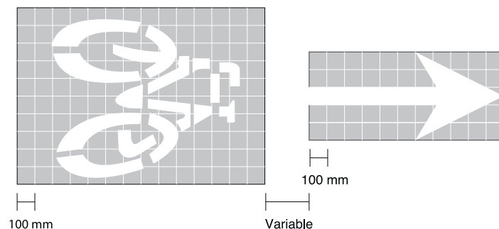
Figura 28.- Marca viària de les vies ciclistes
