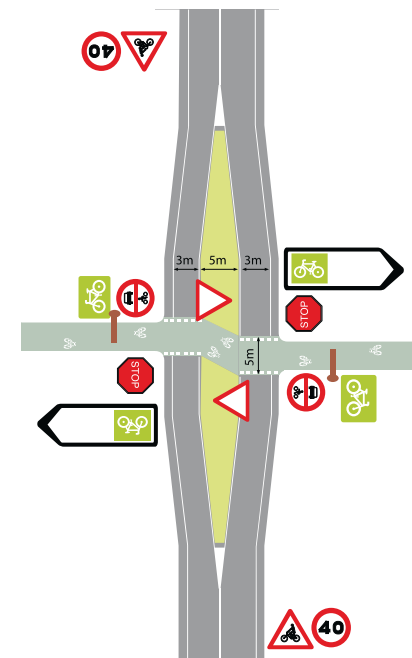
Figura 22.- Intersecció amb via convencional amb trànsit intens
