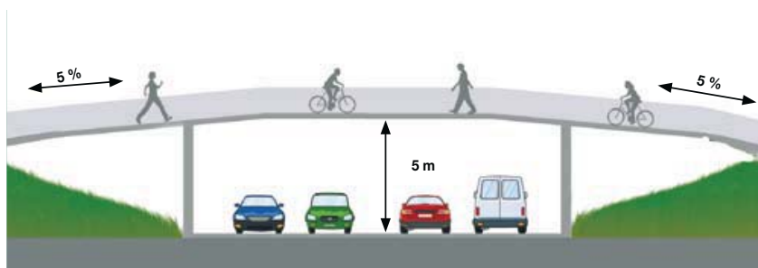
Figura 12.- Pas elevat ciclistes / vianants
