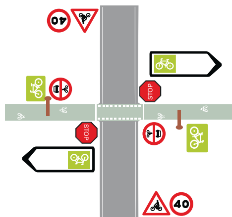
Figura 21.- Intersecció amb via convencional amb trànsit feble
