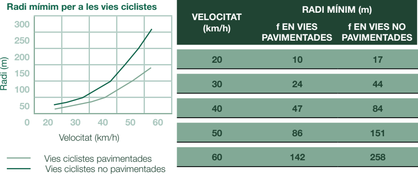
Quadre 5. Radi mínim en vies ciclistes
