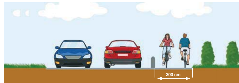
Figura 4.- Carril bici protegit bidireccional en zona interurbana
