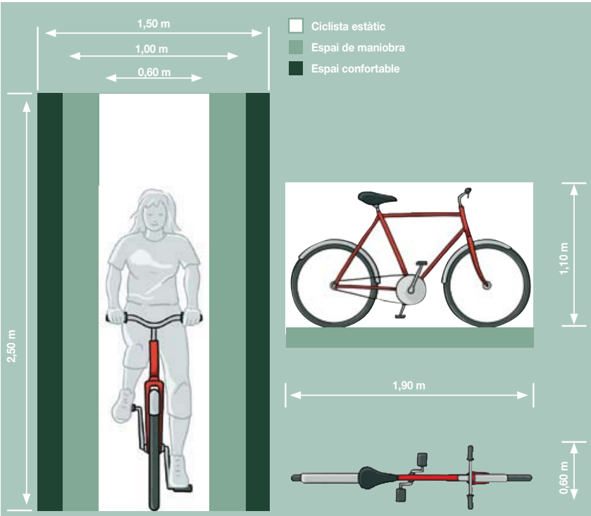
Figura 11.- Espai útil d'un o una ciclista
