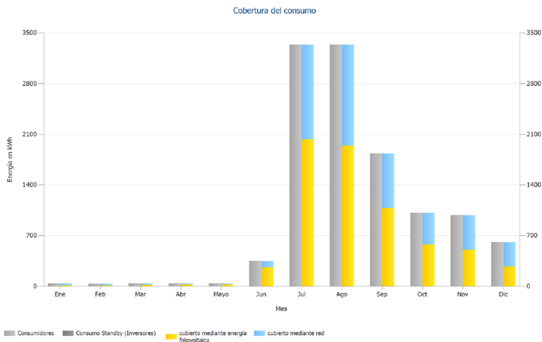
Figura 7: Cobertura solar sobre el consum.
