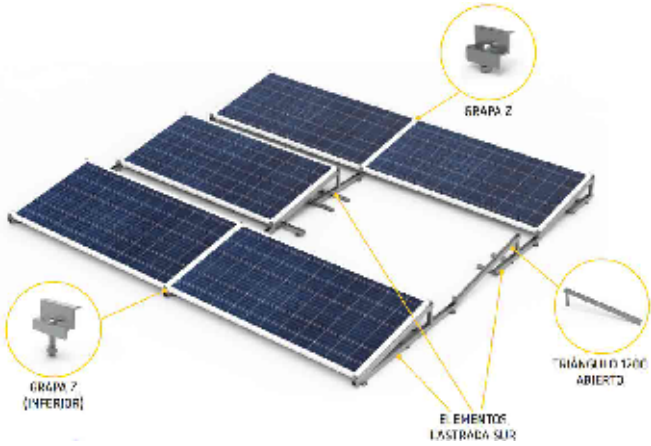
Detall estructura fotovoltaica coberta
