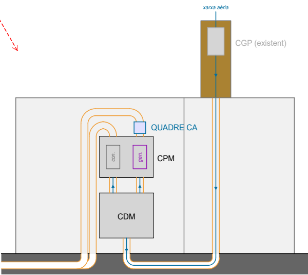
Detall CGP + CDM + CPM doble
