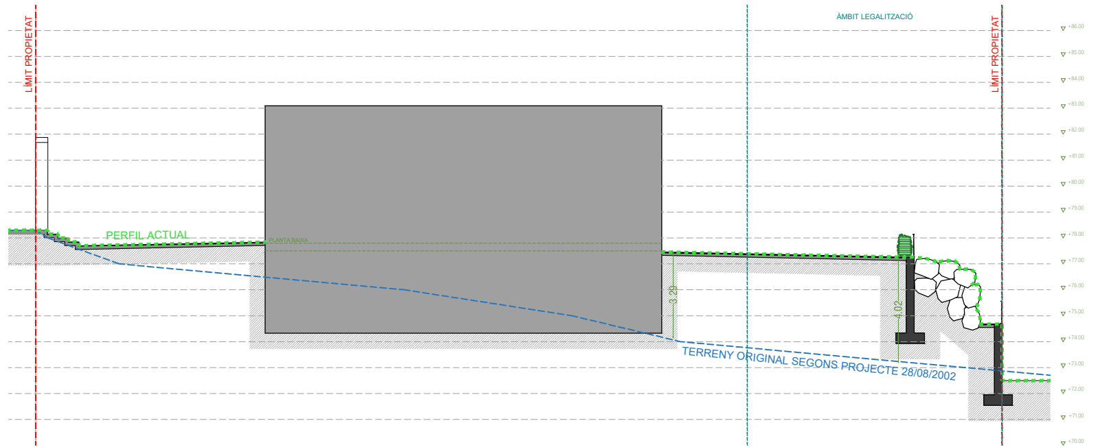
SECCIÓ 2
