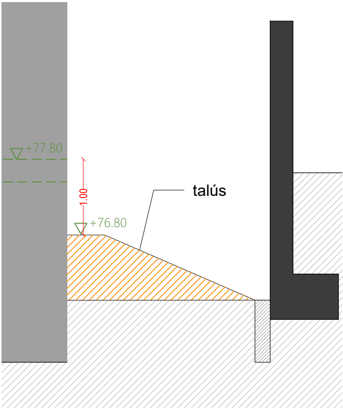
SC3. PROPOSTA
