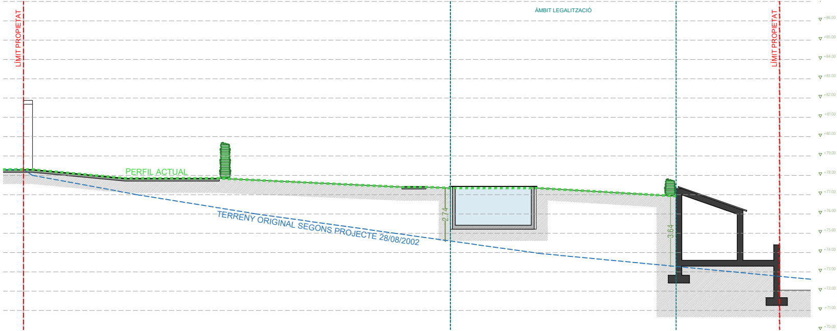
SECCIÓ 4
