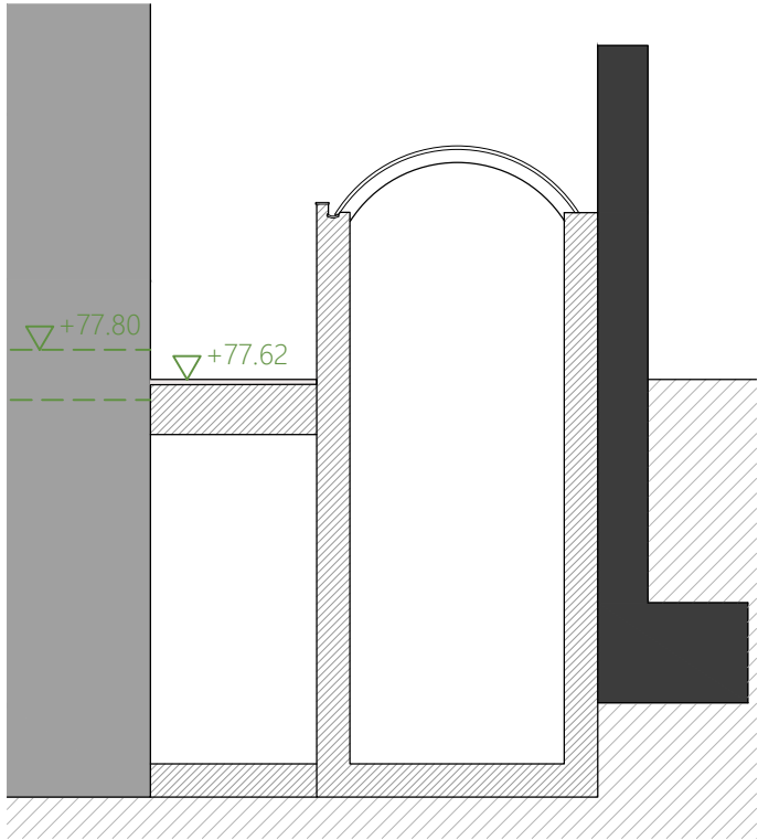
SC1. ESTAT ACTUAL
