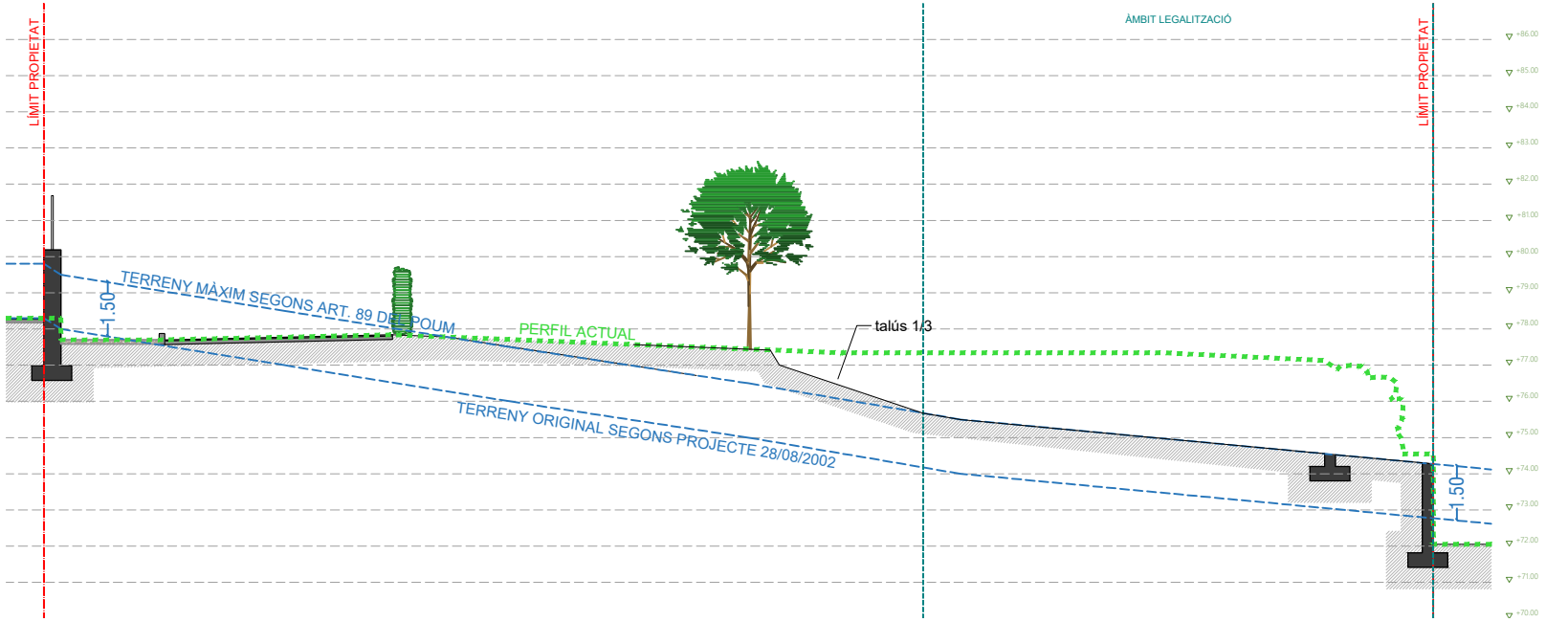
SECCIÓ 3
