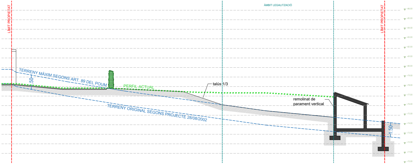
SECCIÓ 4
