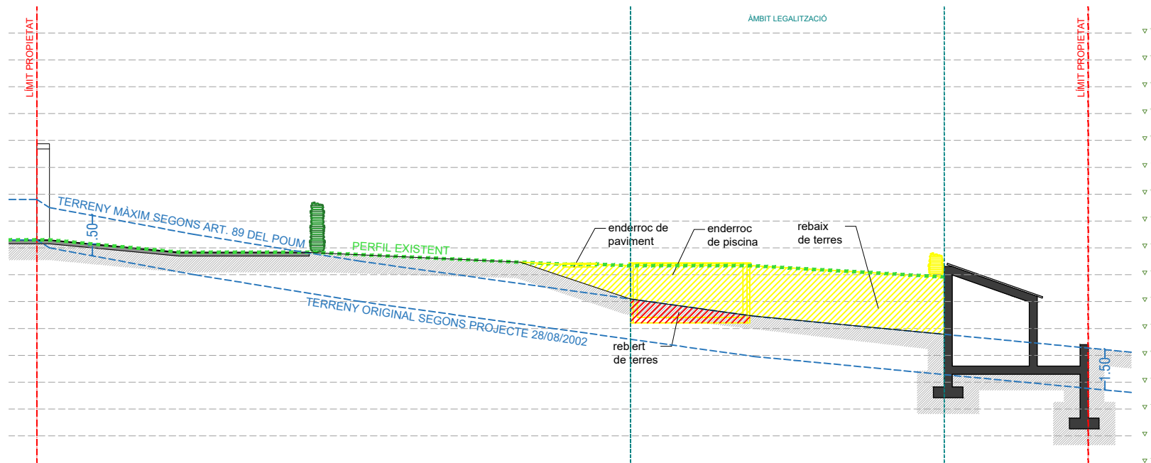
SECCIÓ 4
