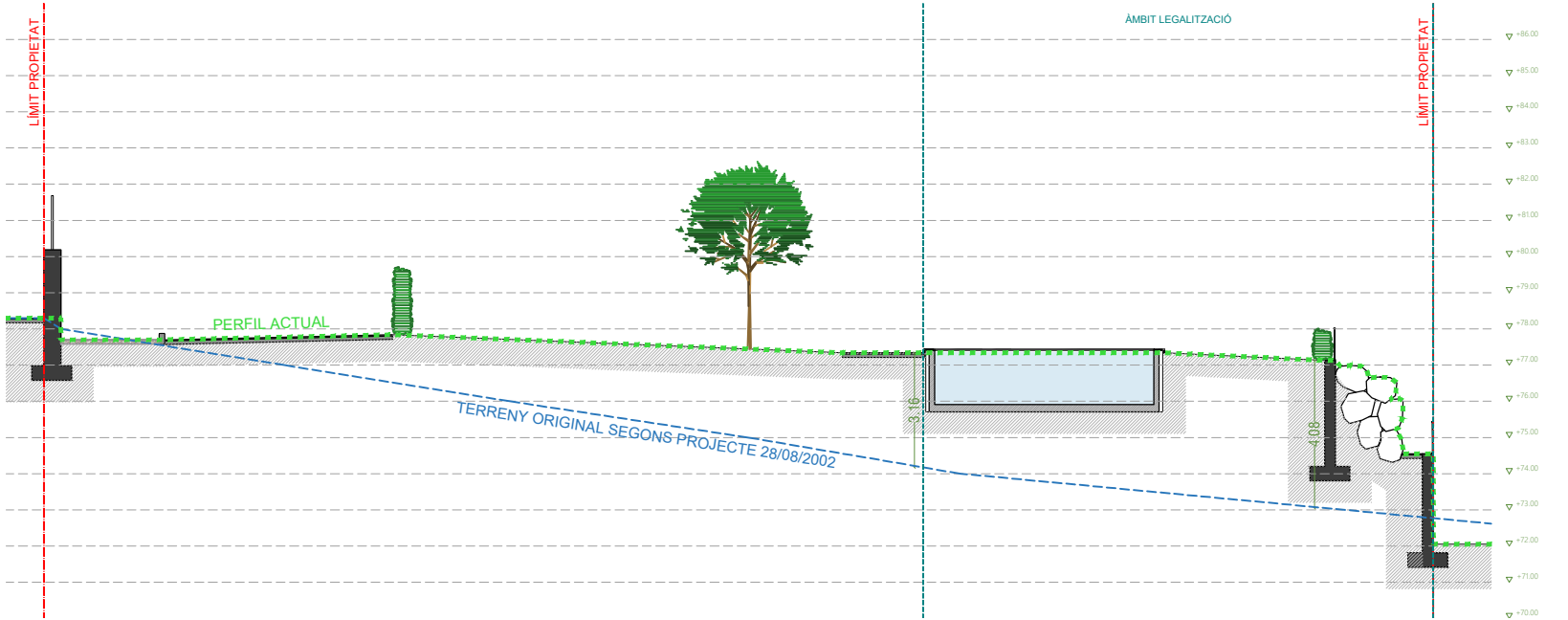
SECCIÓ 3
