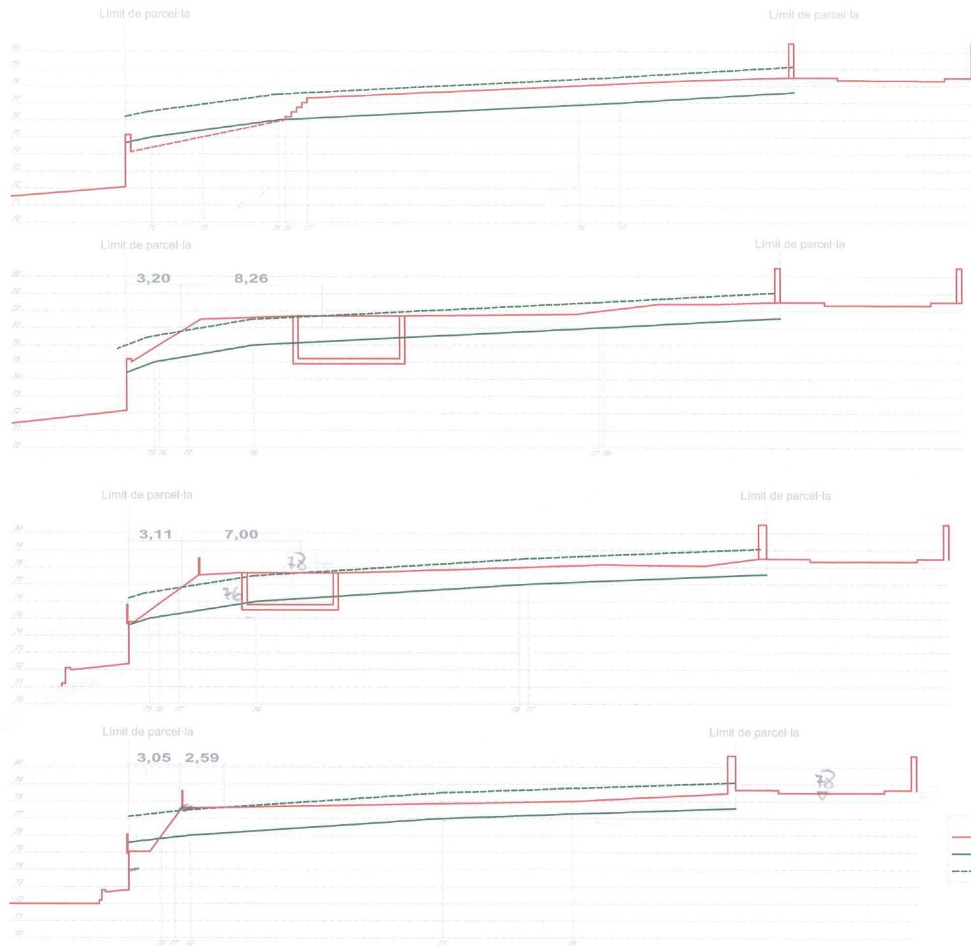
SECCIÓ AA'
