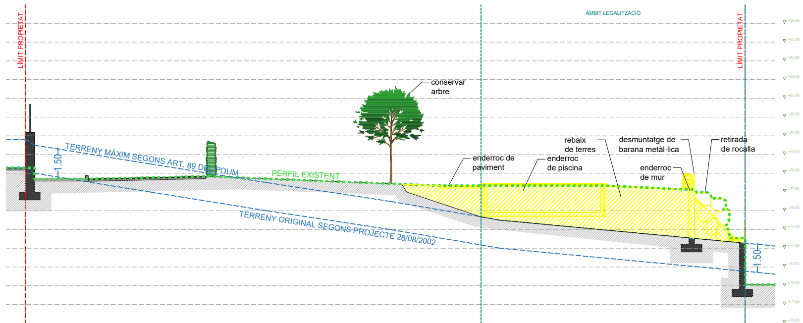
SECCIÓ 3
