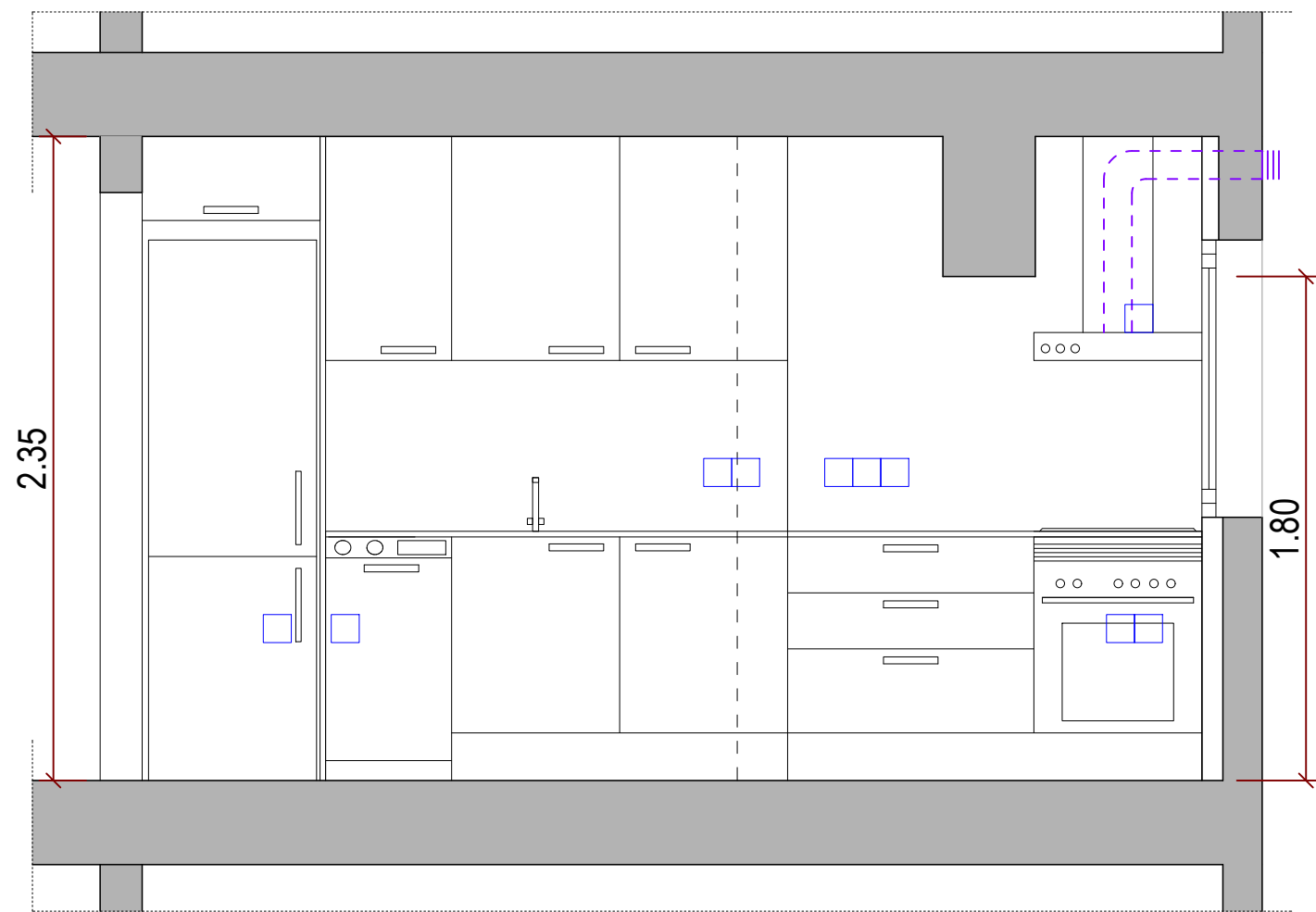
ALÇAT A
