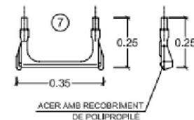
DETALL GRAÓ
