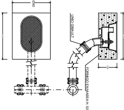
DETALL BOCA DE REC E: 1/100
