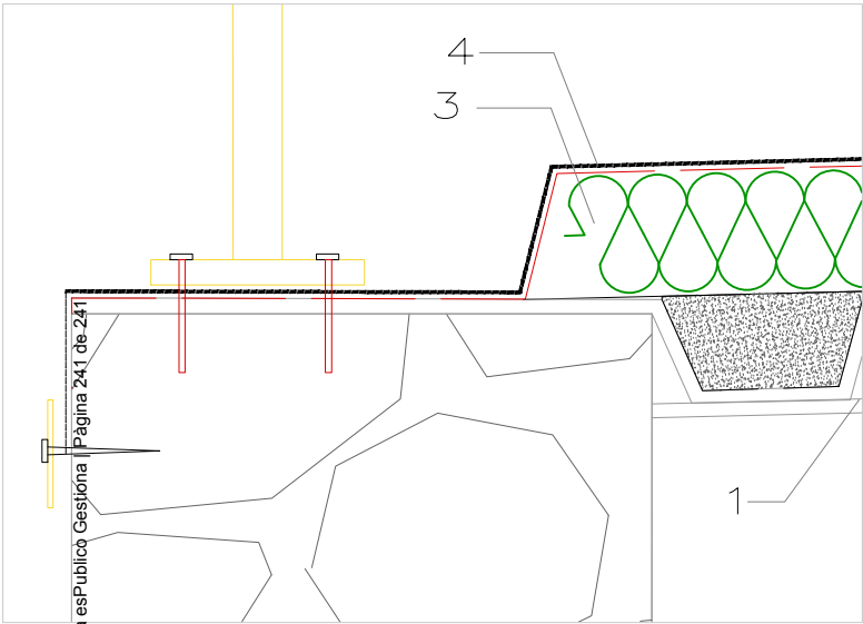
DETALL A
