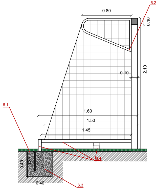
DETALL MUNTATGE ESCAIRE
