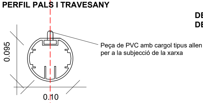
DETALL PERFIL PALS I TRAVESANY
