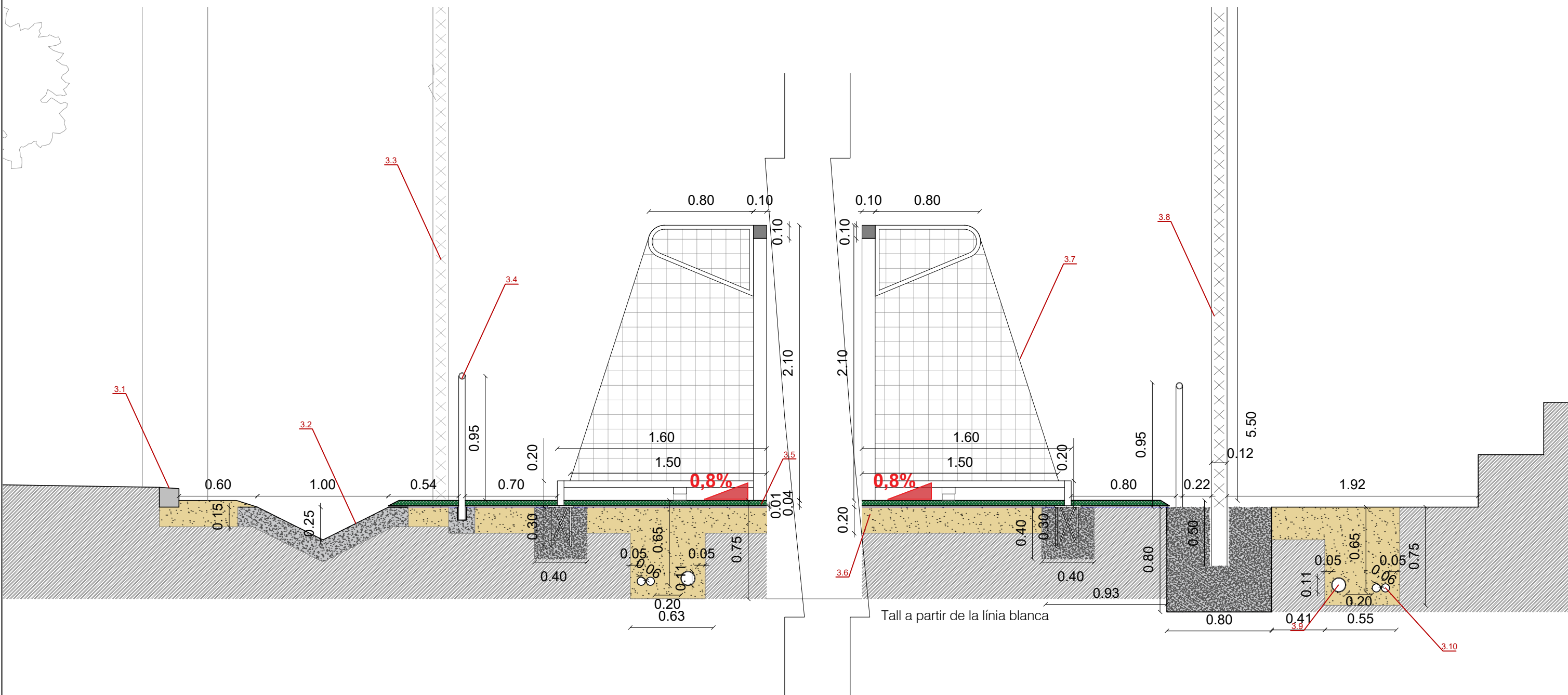
SECCIÓ TRANSVERSAL CONSTRUCTIVA
