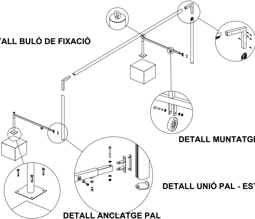
DETALL ANCLATGE PAL
