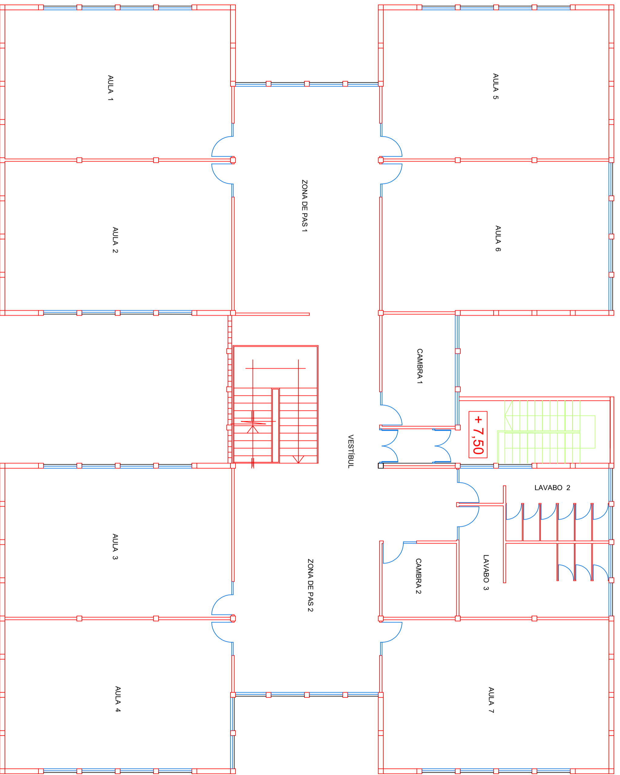
PLANTA SEGONA Sup. Const. 627,00 m 2
