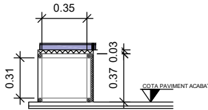
SECCIÓ A -A' 1 : 20
