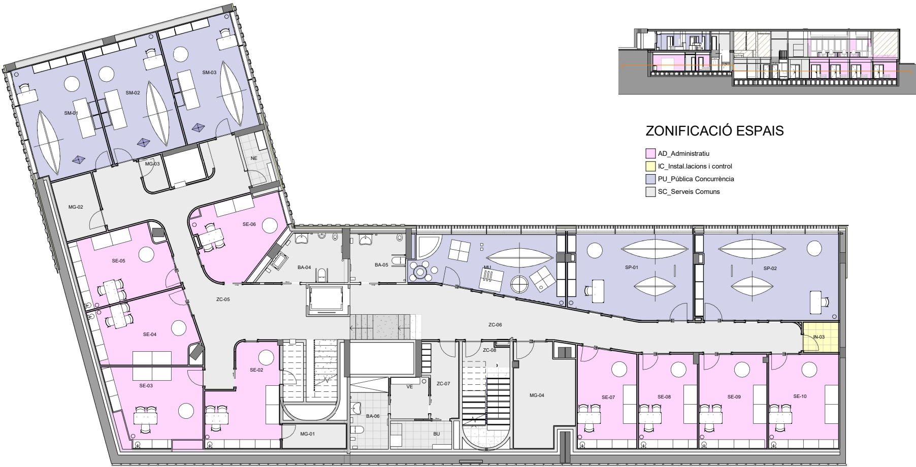
08E0102101-S01 Estat Reformat Funcional 1 : 100
