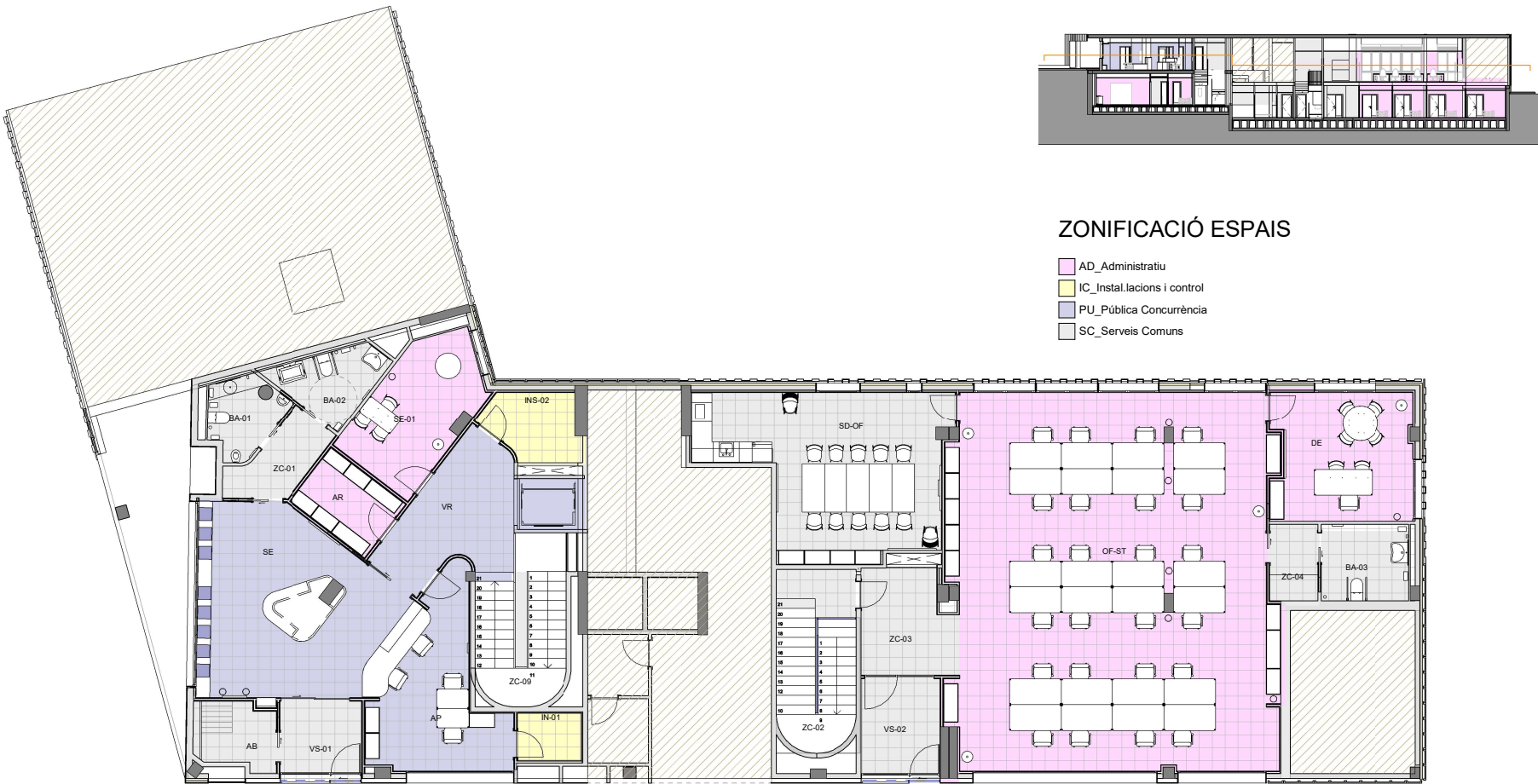
08E0102101-P00 Estat reformat Funcional 1 : 100
