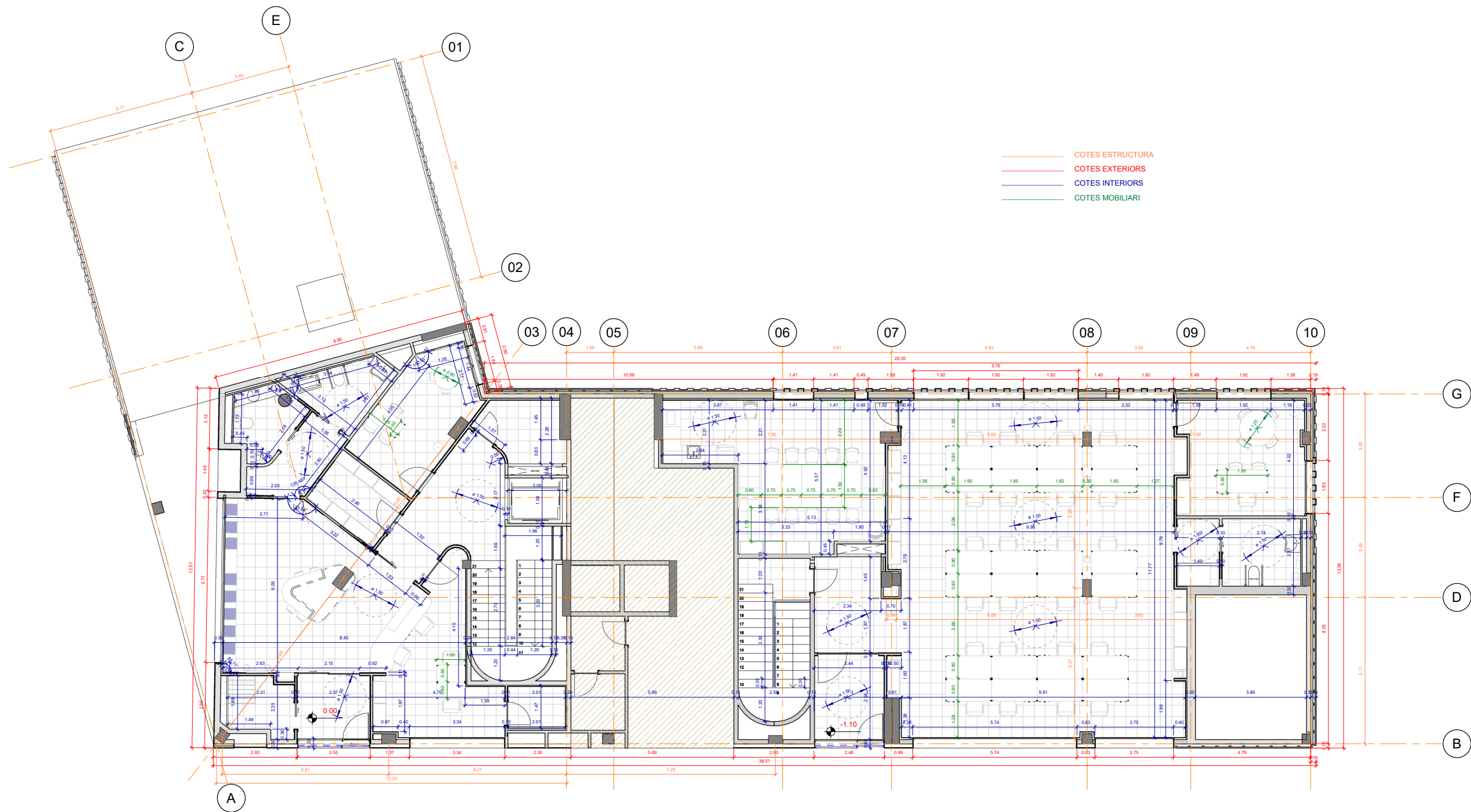
08E0102101-P00 Estat reformat COTES 1:75
