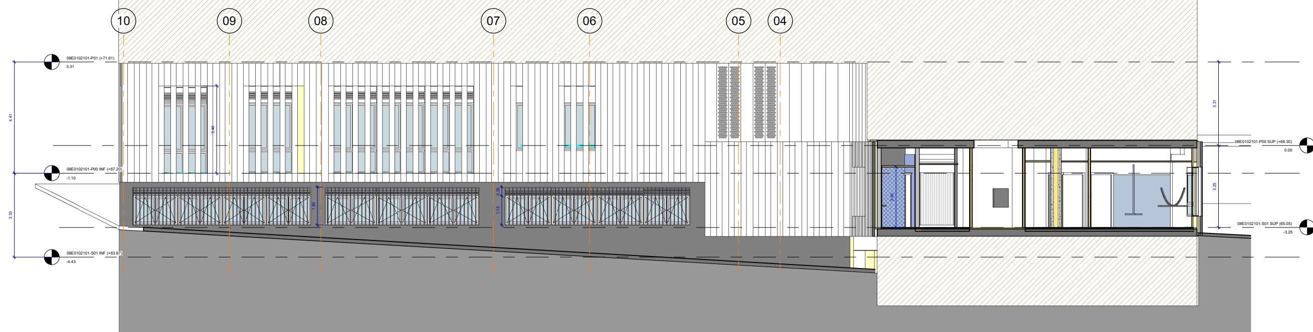
A04 FAÇANA PLAÇA DE LA TERRA 1 : 75
