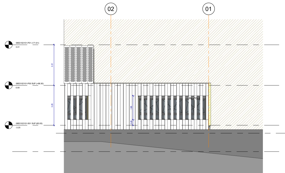
A01 FAÇANA PLAÇA DE LA TERRA 2 1 : 75
