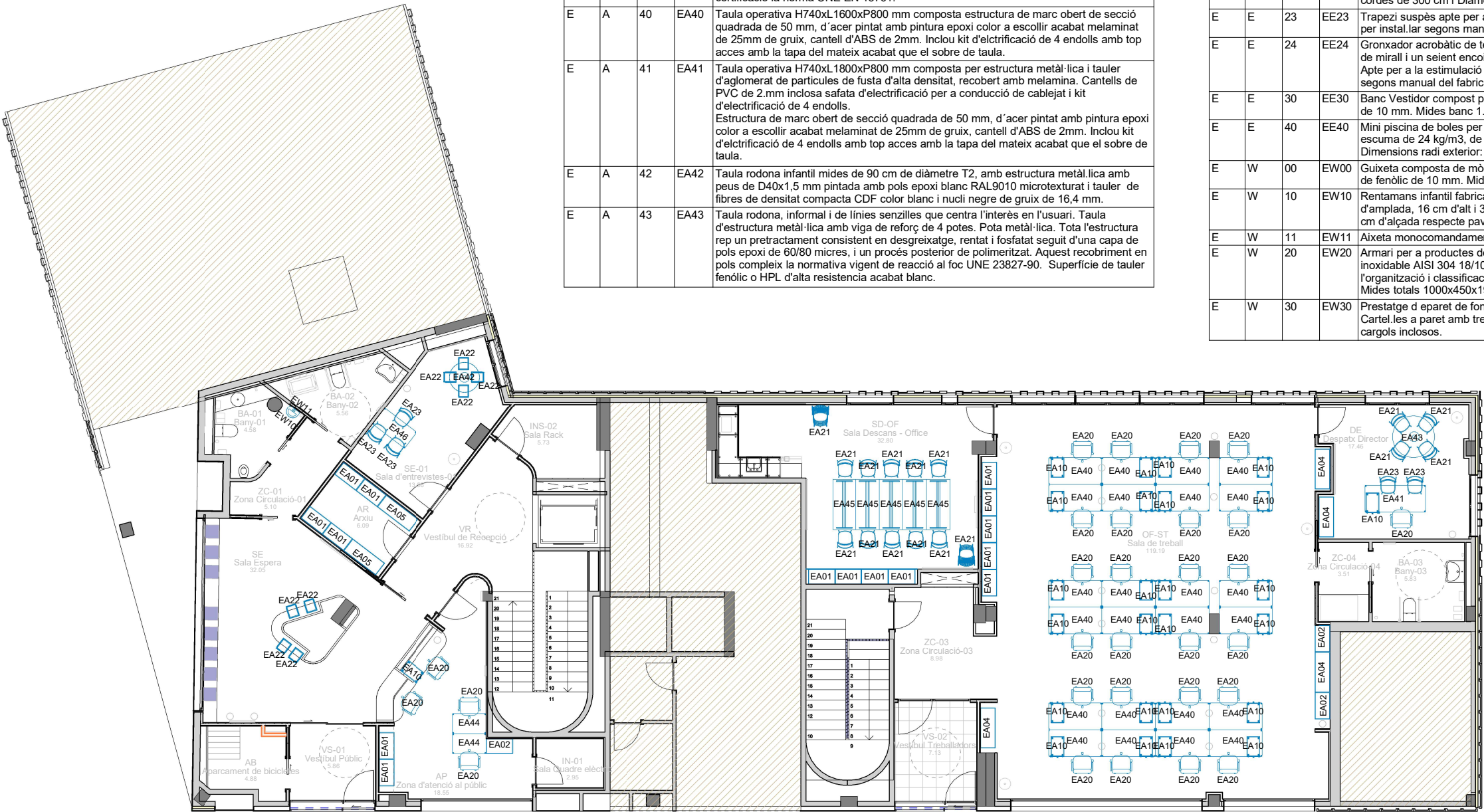
08E0102101-P00 MOBILIARI E 1 : 75
