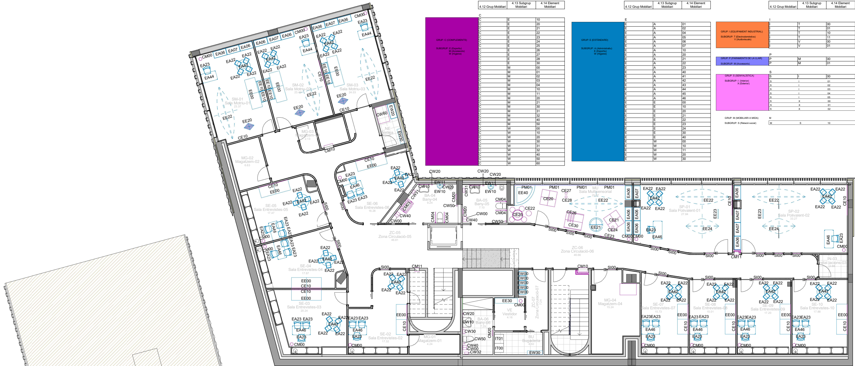
08E0102101-S01 MOBILIARI 1:75
