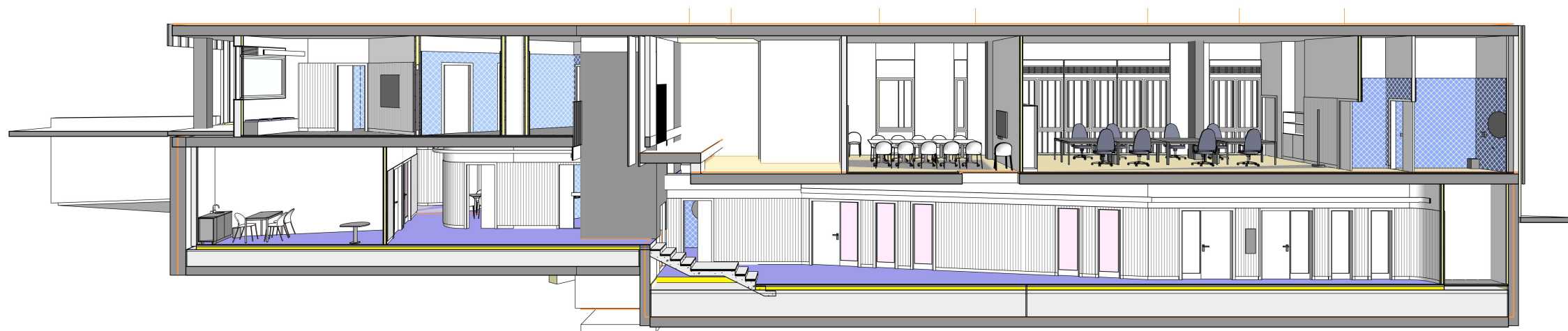
3D SECCIÓ FUGADA
