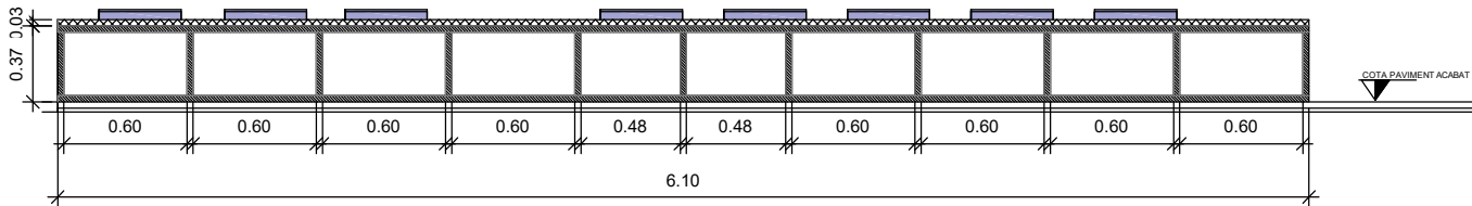
ALÇAT BANC 1 : 20
