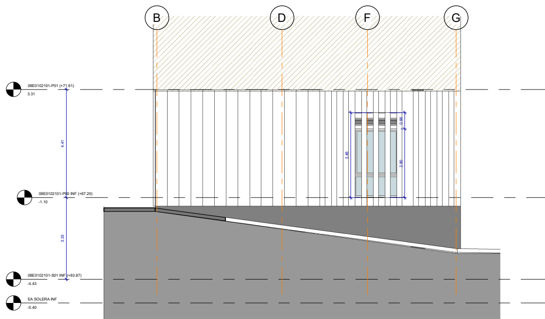
A02 FAÇANA LATERAL 1 : 75
