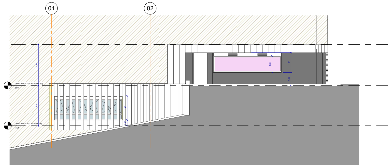
A05 FAÇANA PLAÇA DE L'AIRE 1 : 75
