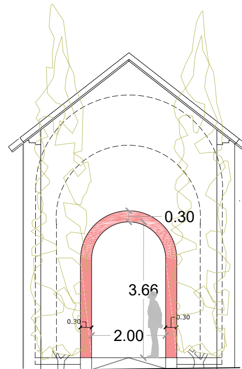
FAÇANA POSTERIOR PROPOSTA OBERTURA
