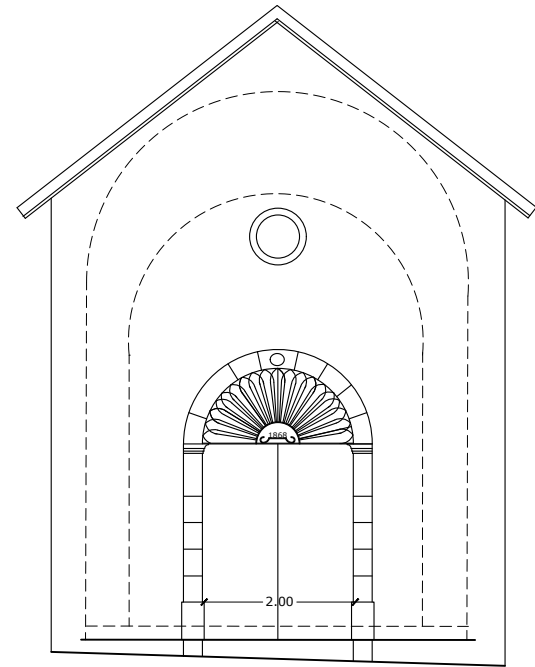
FAÇANA PRINCIPAL ESTAT ACTUAL
