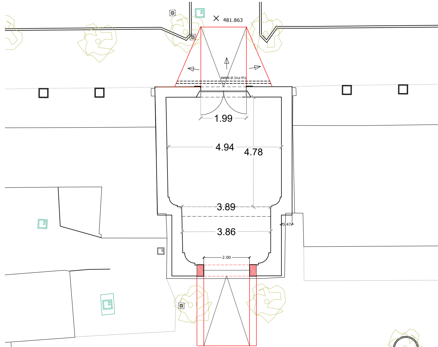
PLANTA PROPOSTA
