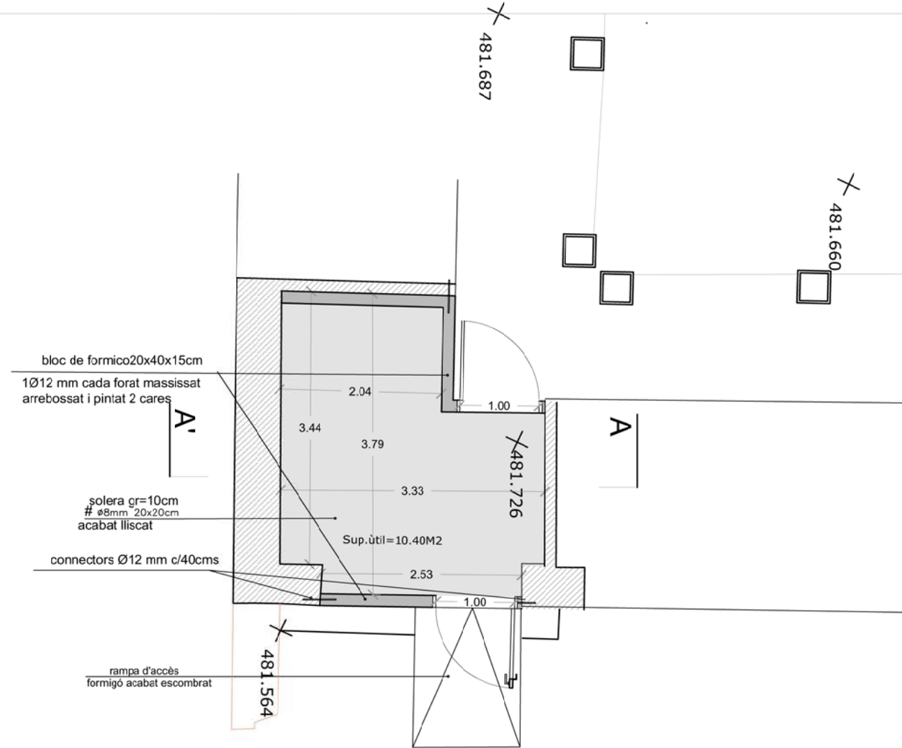
SECCIÓ A-A'
