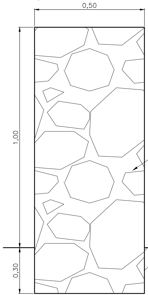
DETALL MUR PEDRA SECA ESCALA=1/10
