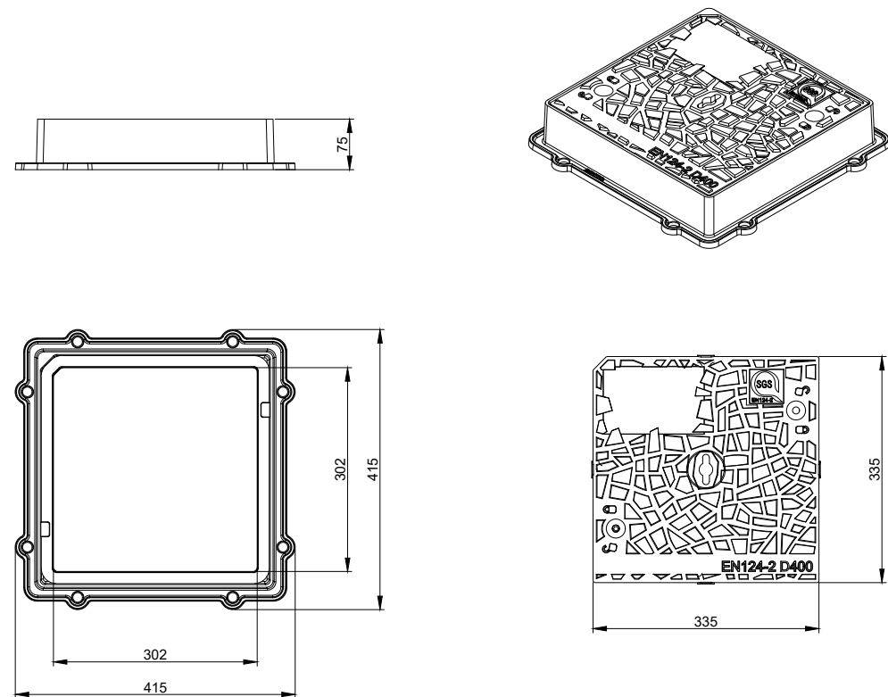
MARC I TAPA D-400
