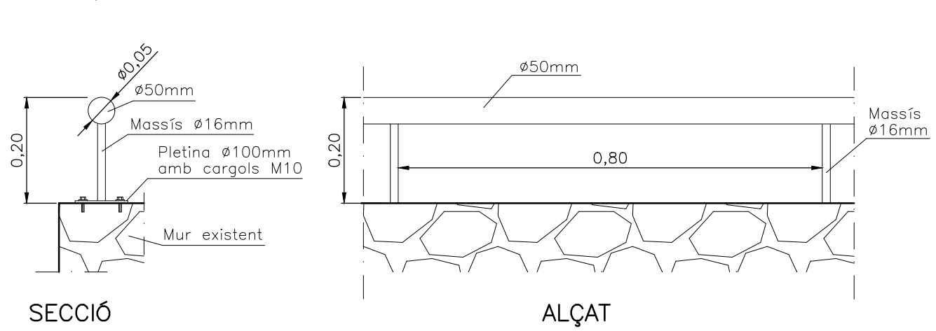
DETALL BARANA SOBRE MUR EXISTENT ESCALA=1/10
