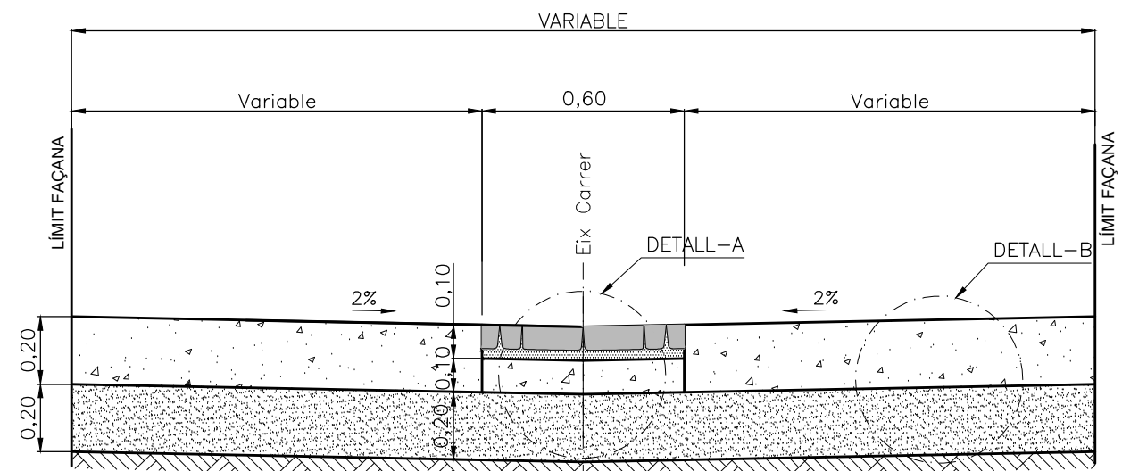
SECCIÓ TIPUS ESCALA=1/20
