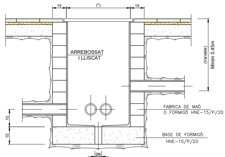
DETALL TRONETA TIPUS SENSE ESCALA
