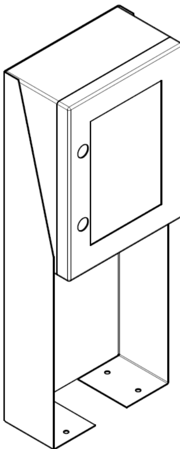
Dibuix general armari més suport
