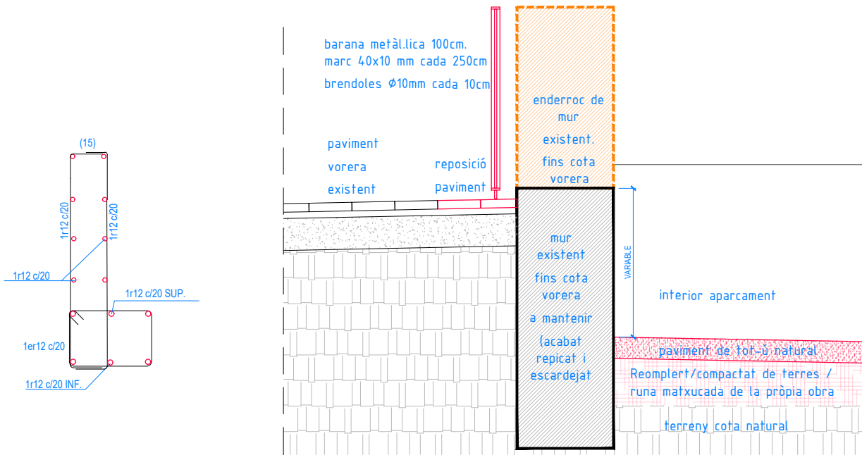
DETALL MUR TIPUS 3 EA3: 1/25
