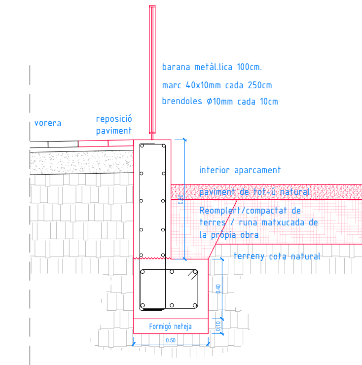
DETALL MUR TIPUS 2 EA3: 1/25
