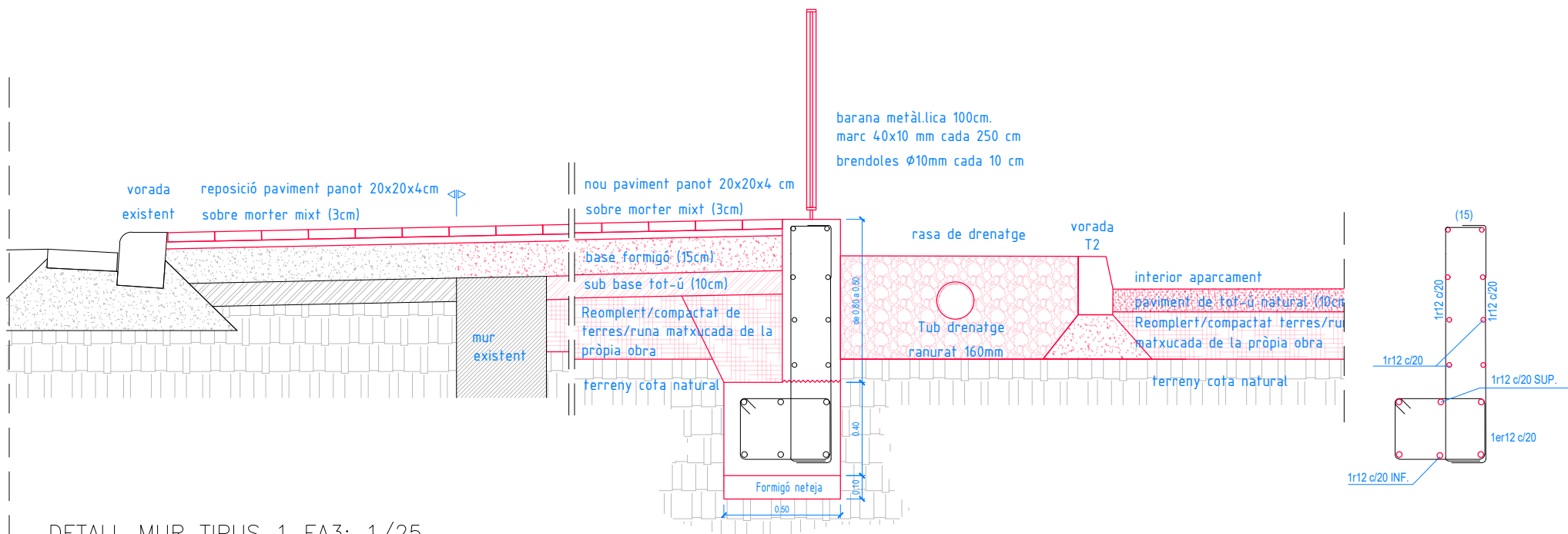
DETALL MUR TIPUS 1 EA3: 1/25
