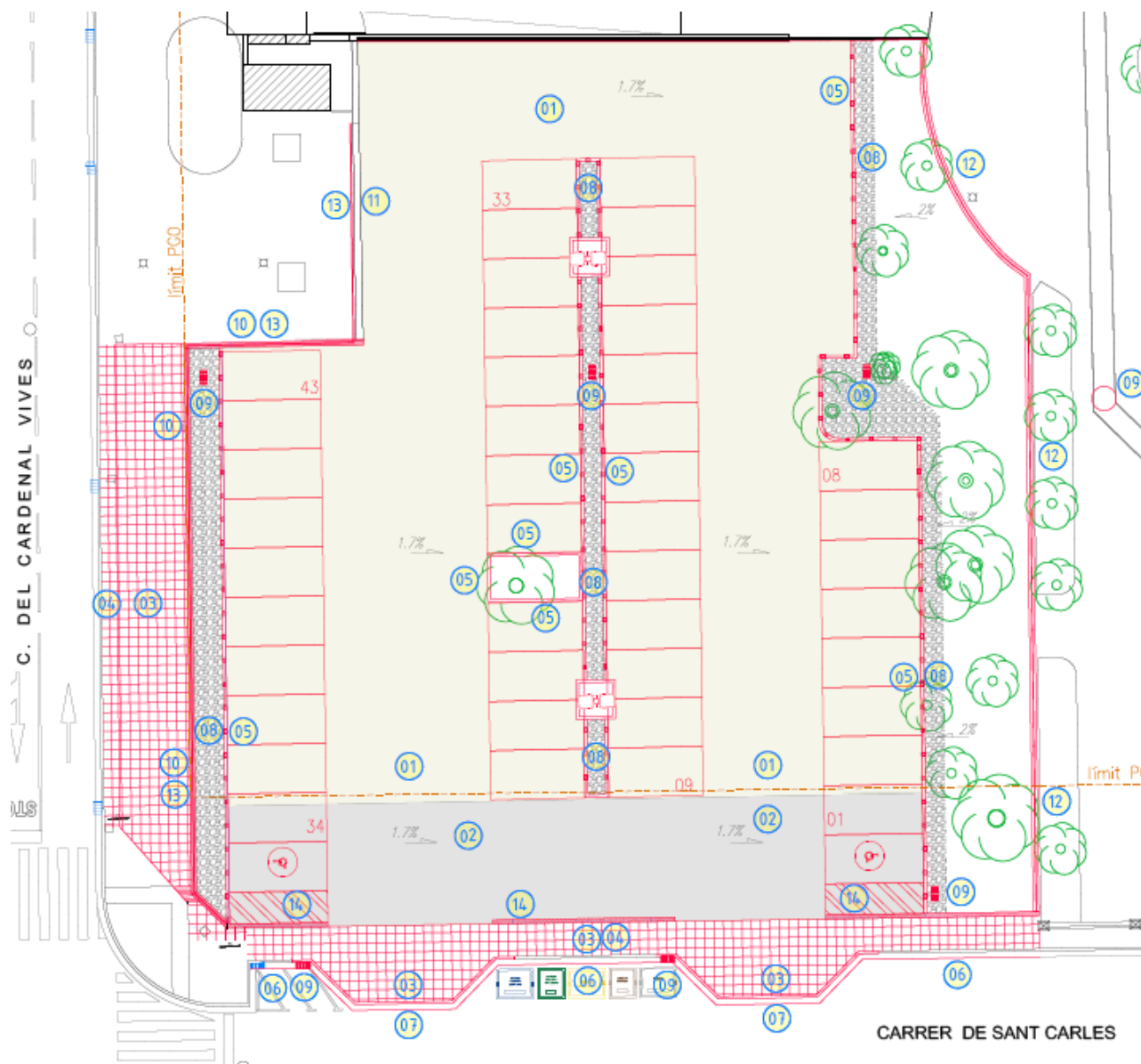
PLANTA ESTAT ACTUAL
