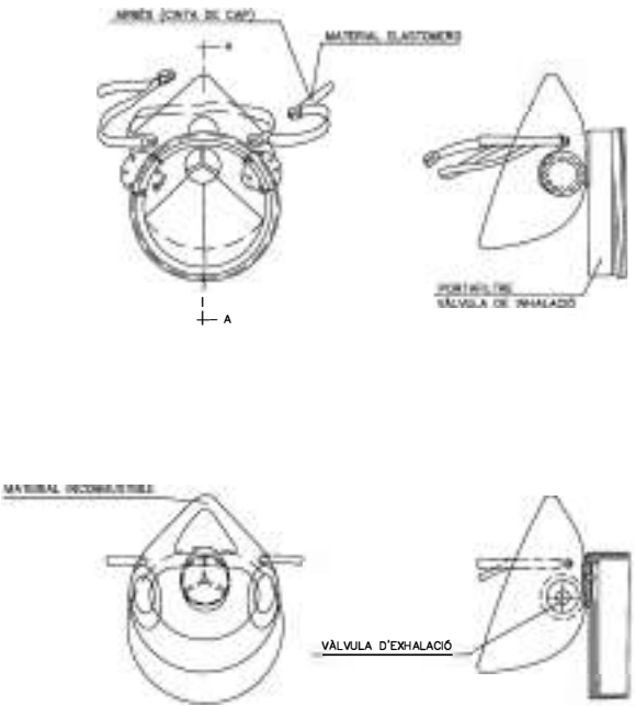
SECCIÓ A-A
