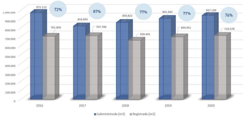
Gràfica aigua subministrada i registrada i rendiments
