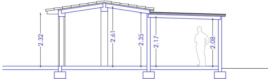
SECCIÓ A
