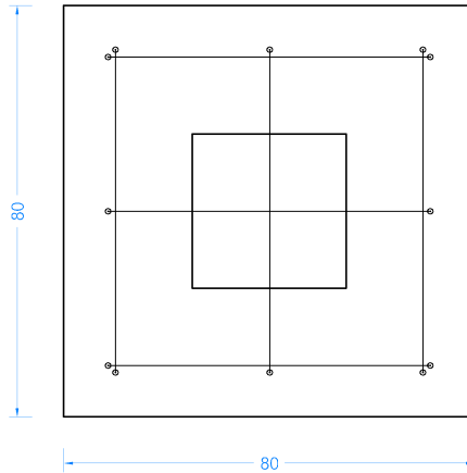
PILARS D'OBRA 30x30
