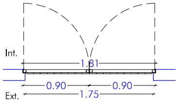
PORTA TIPUS S-2 1 unitat
