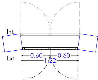
PORTA TIPUS S-1 5 unitats
