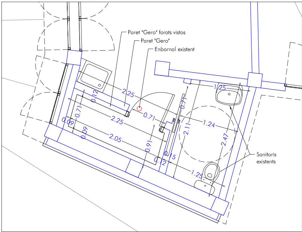
DETALL BANY I ZONA COMPRESSOR
