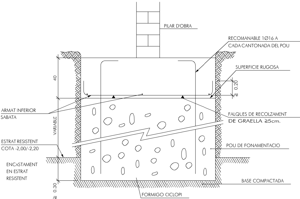
Sabata Sobre Pou de Fonamentacio
