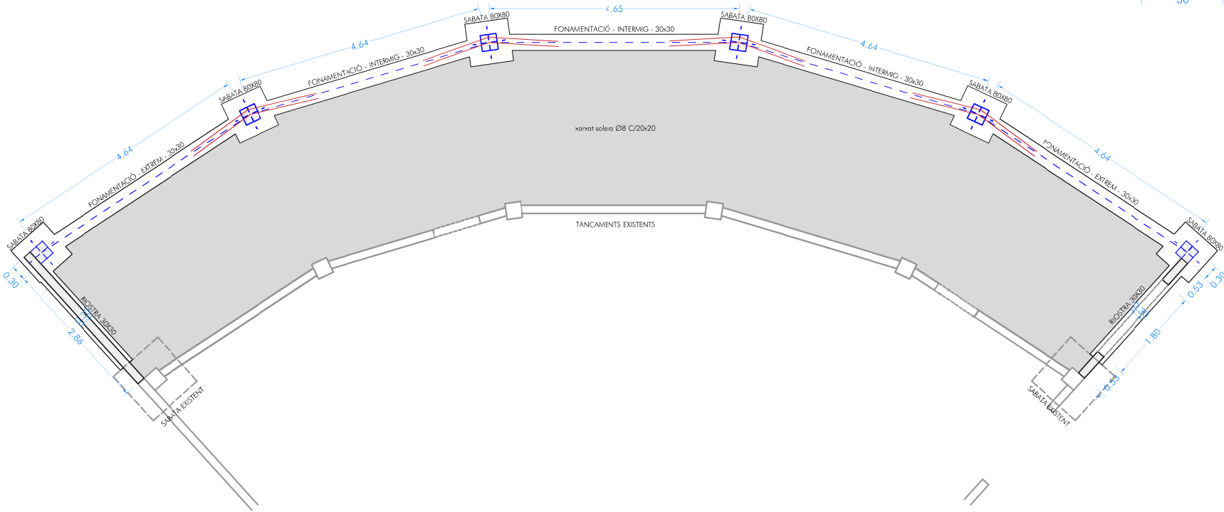
PLANTA FONAMENTS
