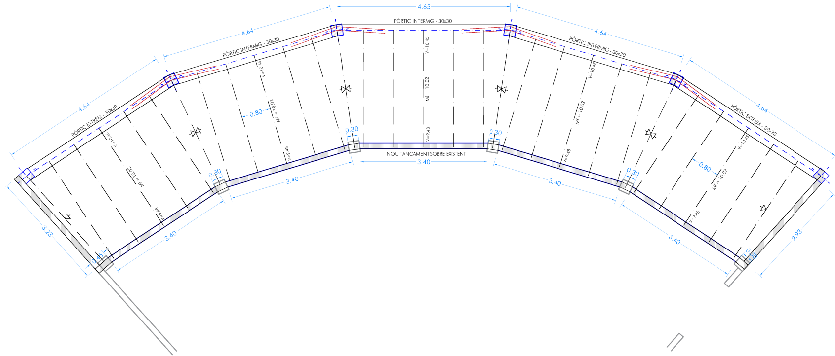
SOSTRE PLANTA BAIXA
