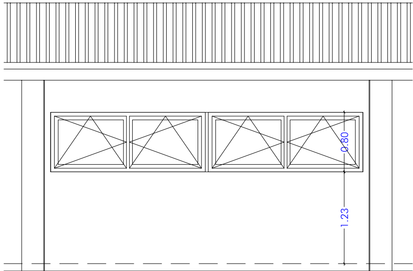
ALÇAT FUSTERIES
