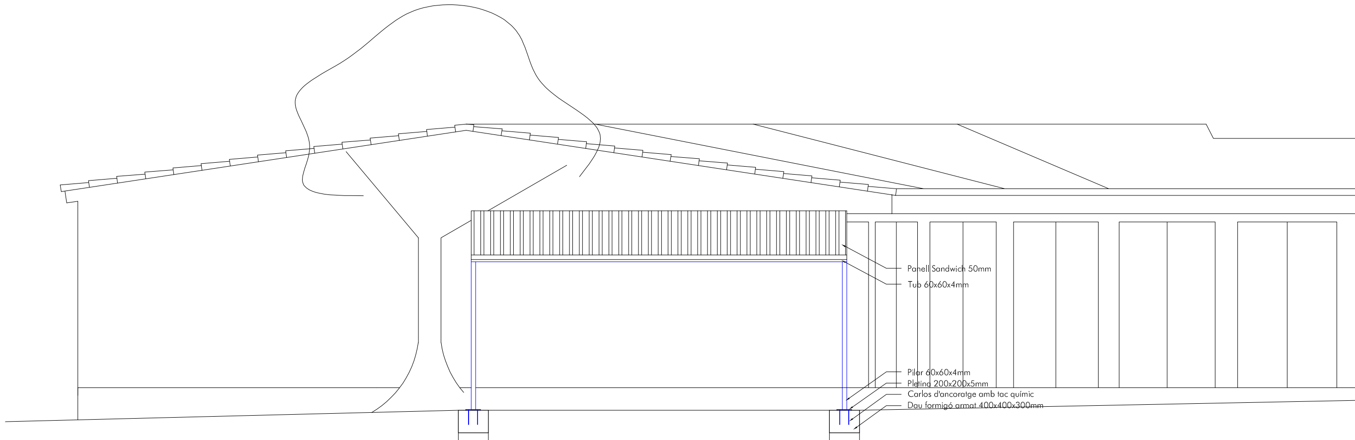
ALÇAT ZONA FOSSAT e.1/50
