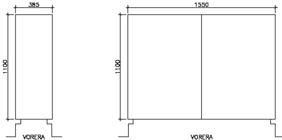
Armari d'intempèrie TIPUS 2
