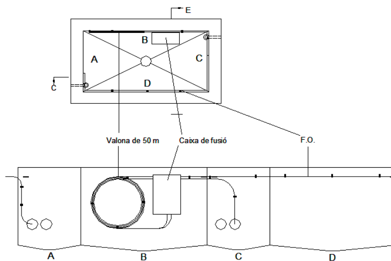
Croquis instal·lació caixes empiulament
