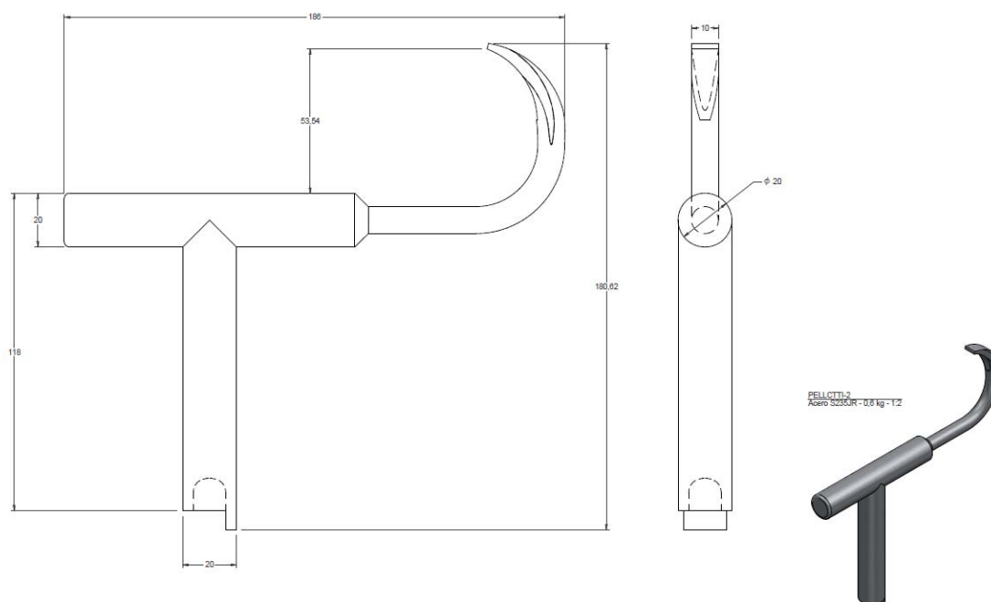
Exemple ganxo/clau tanca de seguretat
