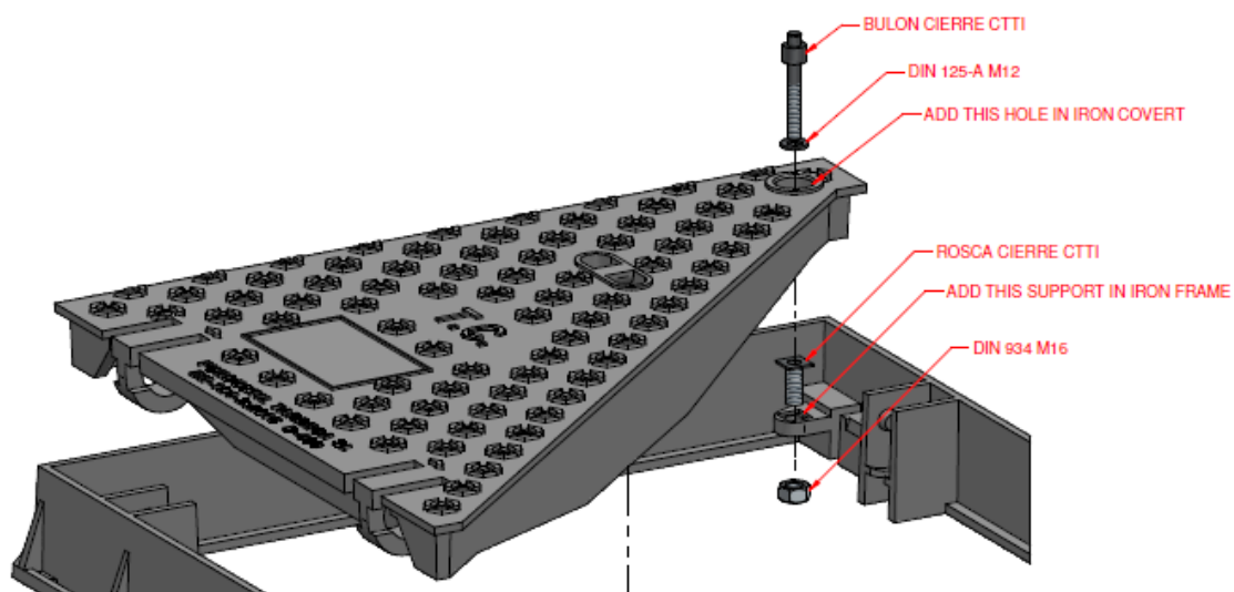
Exemple tanca de seguretat pericó tipus B2/C2
