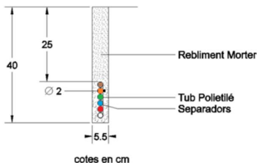
Exemple microrasa en calçada amb configuració Base 1
