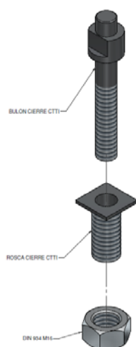
Exemple tanca de seguretat pericó tipus B2/C2
