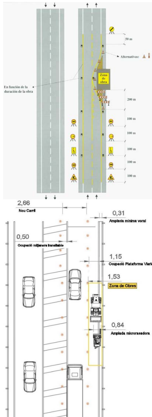
Senyalització de reducció de carril segons 8.3 I.C de Carretres
