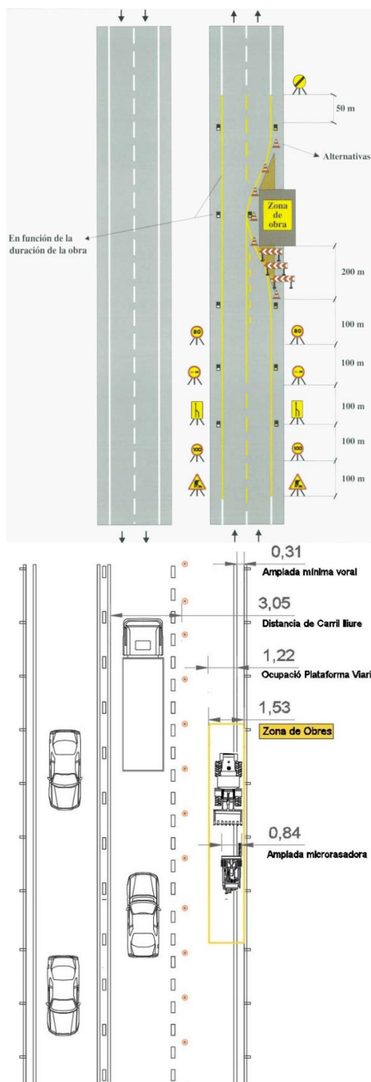
Senyalització per a tall de carril segons 8.3 IC de Carreteres
