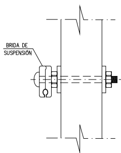
Brida de suspensió d'acer galvanitzat per cable autosuportat
