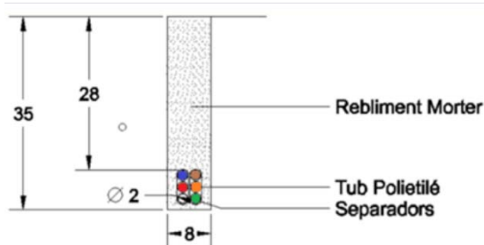
Exemple microrasa en calçada amb configuració Base 2
