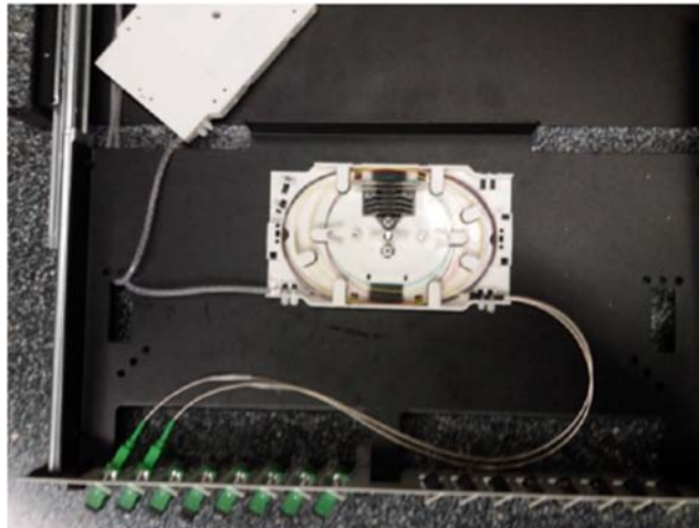
Reparditor 16 posicions SC/APC
