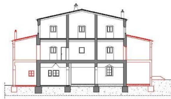
Secció AB de Can Giberga o Can Maragall, amb les galeries afegides posteriorment en vermell.
