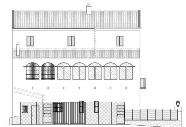
Alçat façana oest
