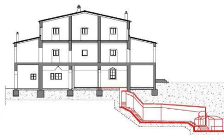
Secció AB de Can Maragall, amb l'hipogeu en vermell construït en una data indeterminada.
