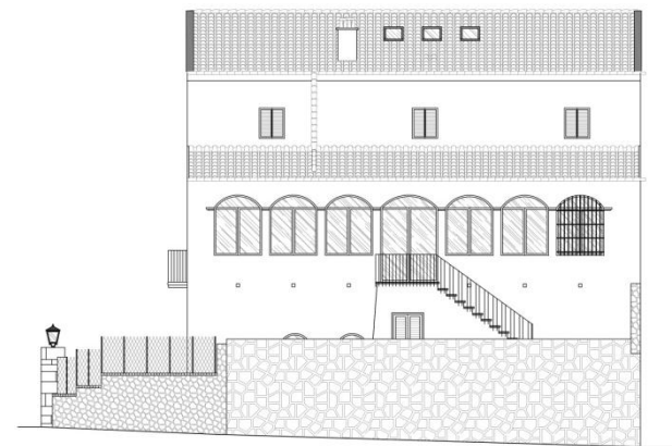
Alçat façana est
