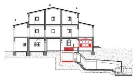
Secció AB de Can Maragall, amb la porta per vehicles rodants, el canvi de cota, i les escales d'accés intern en vermell, reforma datada cap a mitjans del segle XX.
