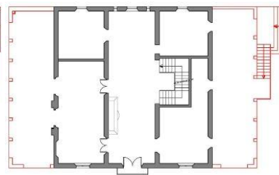
Plànol de la primera planta de Can Giberga o Can Maragall, amb les galeries afegides posteriorment en vermell.
