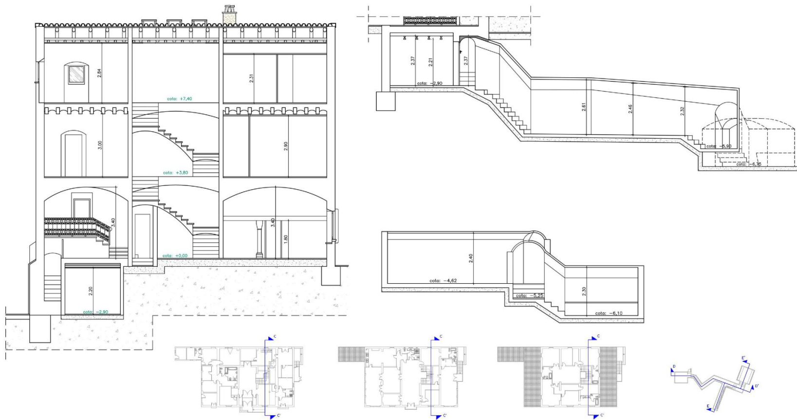
Secció transversal "C", "D" i "E"
