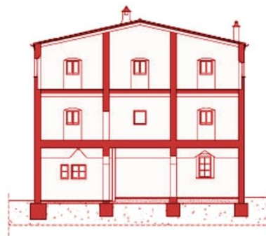
Secció AB de Can Giberga o Can Maragall, amb l'ampliació del segle XVIII en vermell.
