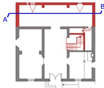
Plànol de la planta baixa de Can Giberga o Can Maragall, amb l'ampliació del segle XVIII en vermell i la línia de secció AB en blau.
