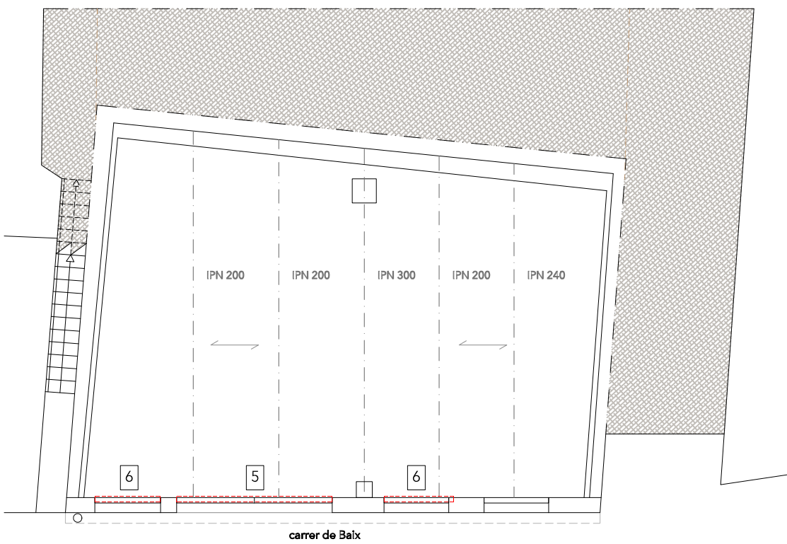
PLANTA BAIXA 2
