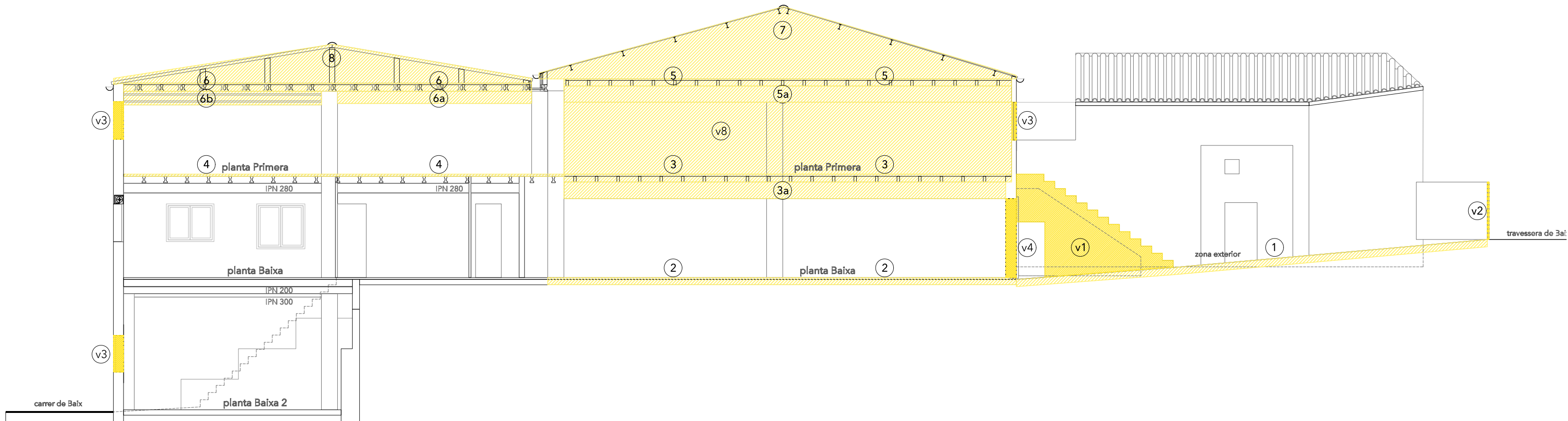
SECCIÓ LONGITUDINAL
