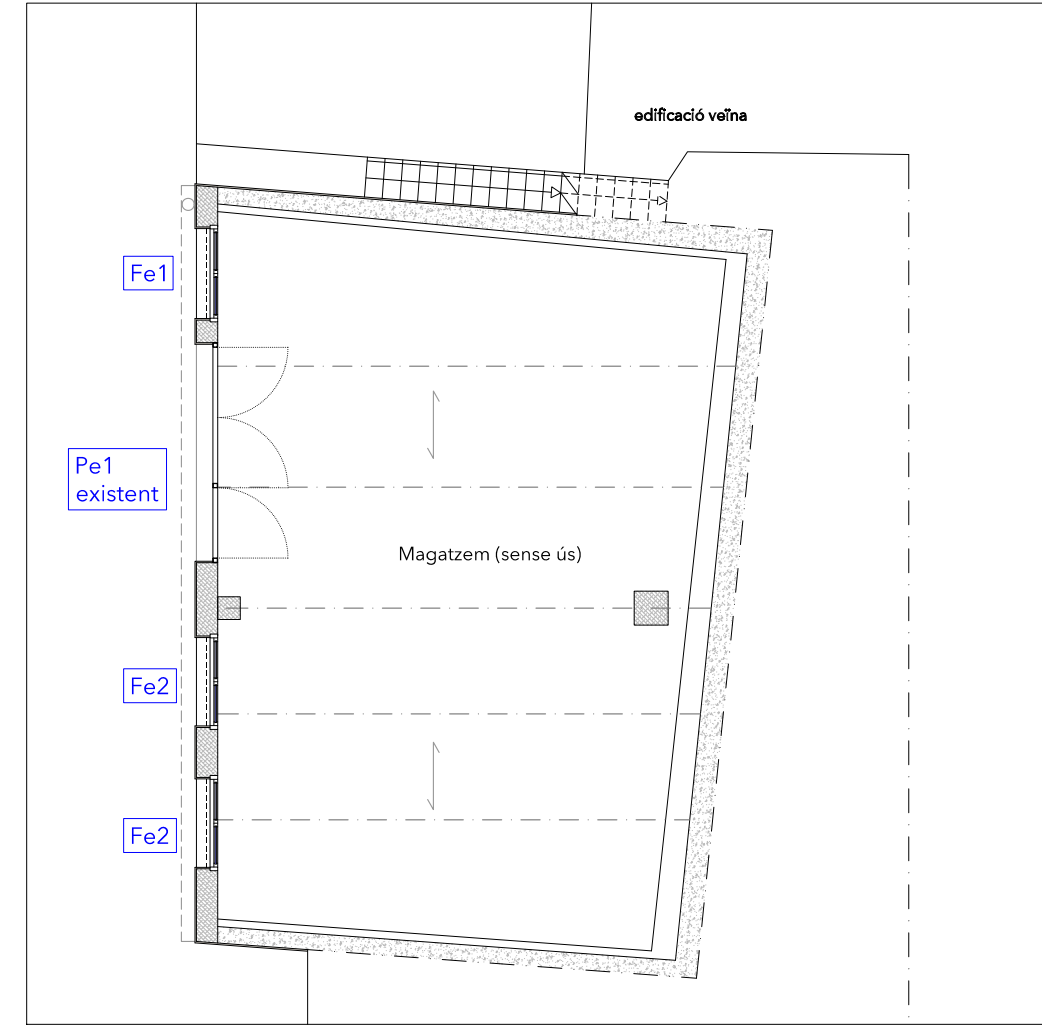
PLANTA BAIXA 2
