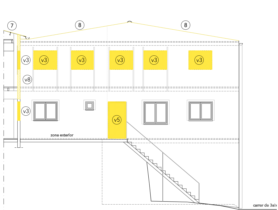
FAÇANA 2 - carrer de Baix
