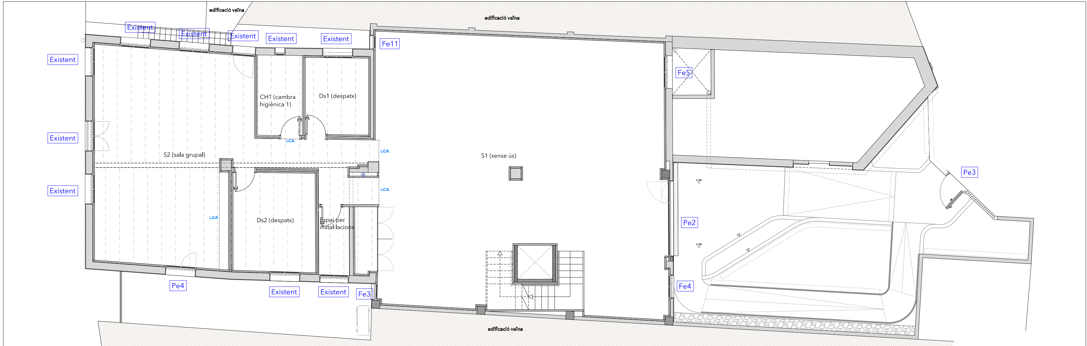
PLANTA BAIXA
