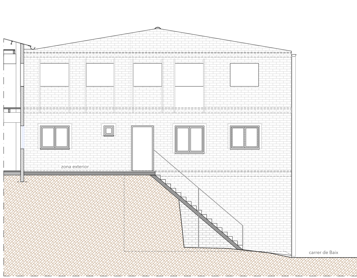
FAÇANA 3 - LATERAL OEST
