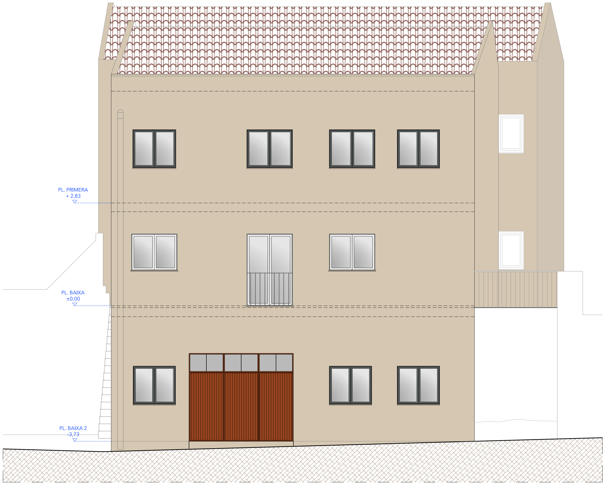
FAÇANA 3
