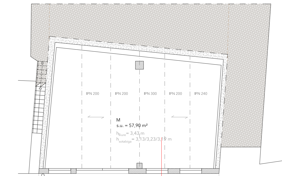
PLANTA BAIXA 2
