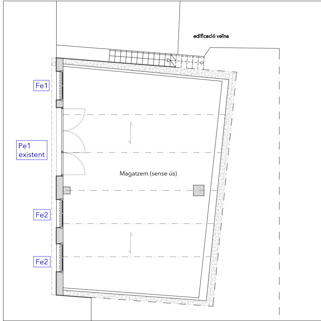
PLANTA BAIXA 2
