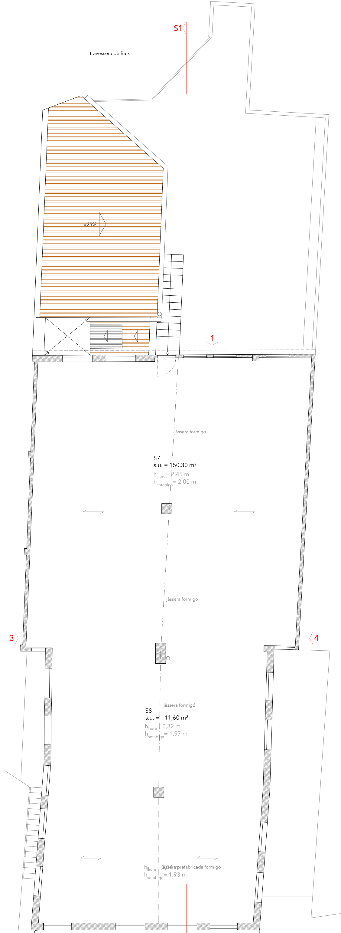
PLANTA PRIMERA
