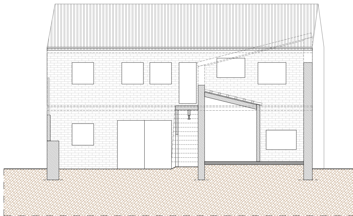
FAÇANA 1 - NORD (zona exterior)
