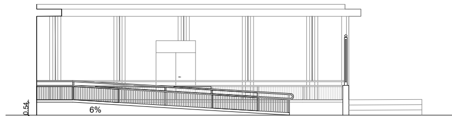
Secció a-a' E. 1 : 75 DIN A3
