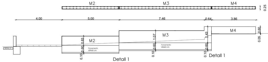
Detalls de murs M2, M3, M4
