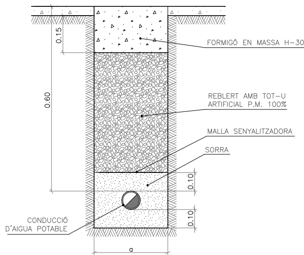
SECCIÓ TIPUS D RASA TIPUS EN VIAL FORMIGONAT ZONA URBANA
