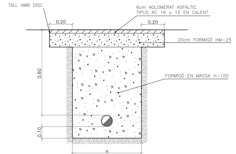
SECCIÓ TIPUS C RASA TIPUS EN VIAL ASFALTAT ZONA URBANA
