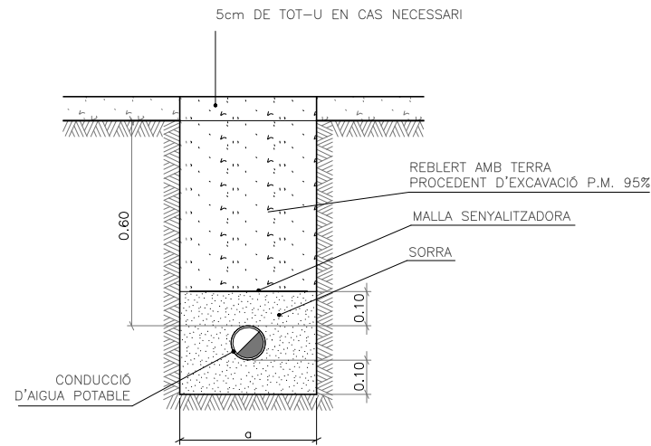
SECCIÓ TIPUS A RASA TIPUS EN TERRA
