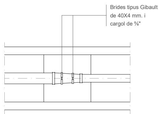
PLANTA CON DE REDUCCIÓ Peces especials
