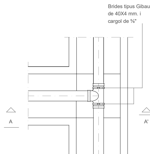
PLANTA DERIVACIÓ EN "T" Peces especials
