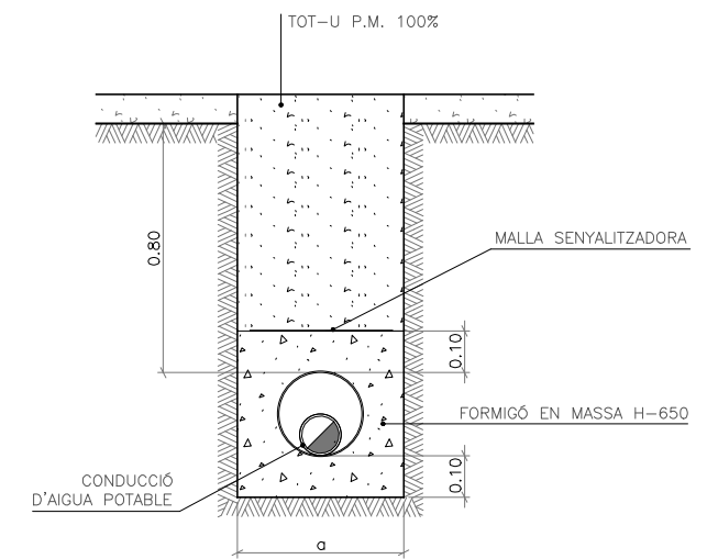
SECCIÓ TIPUS F CREUAMENT PERPENDICULAR VIAL EN ZONA SENSE PAVIMENTAR
