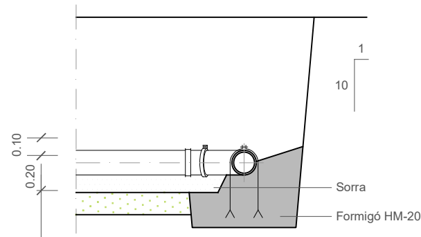
ANCORATGE Peces especials
