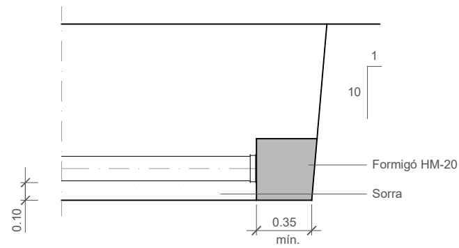
ALÇAT Peces especials
