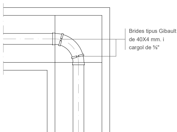
PLANTA DERIVACIÓ A 90° (COLZE) Peces especials
