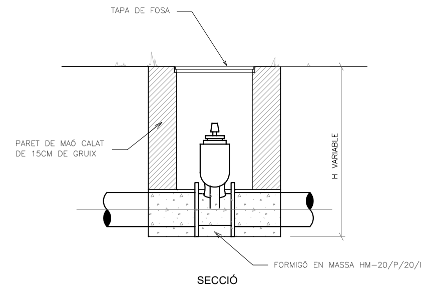
DETALL TIPUS A ARQUETA AMB VÀLVULA
