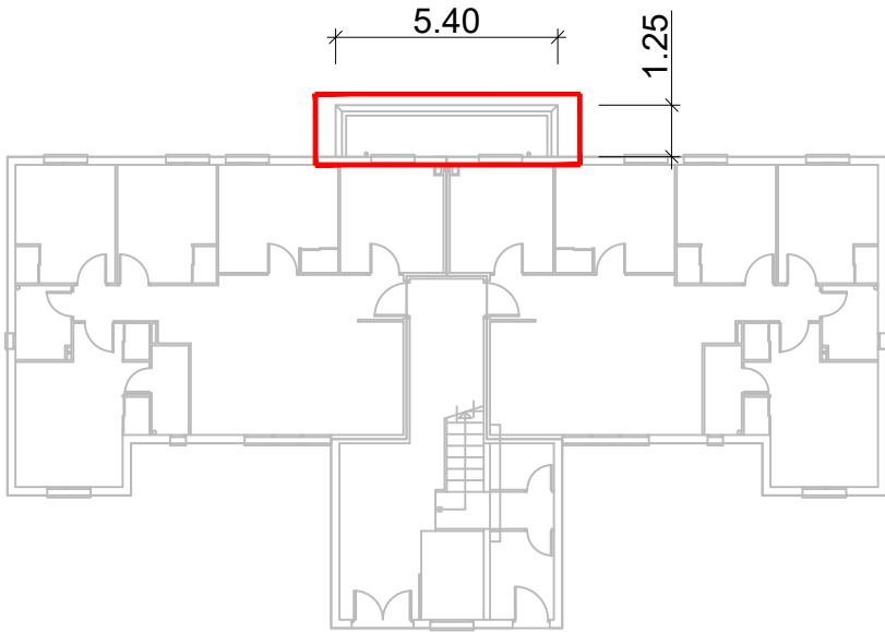
PLANTA TIPUS E 1/200
