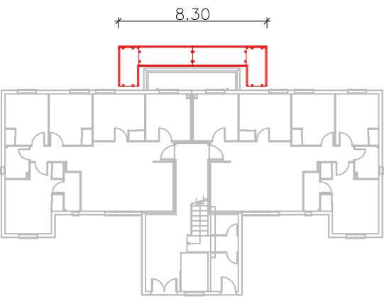
PLANTA E 1/300
