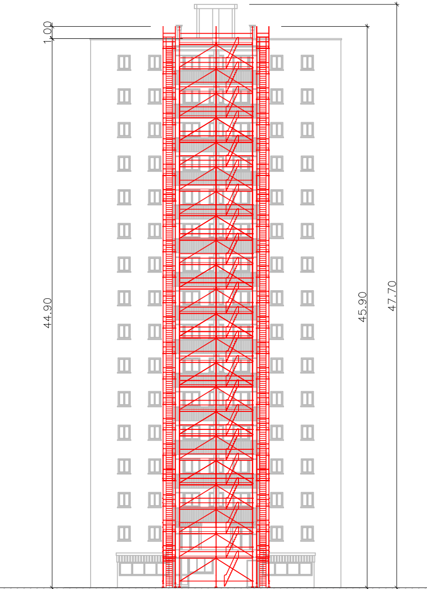
ALÇAT E 1/300
