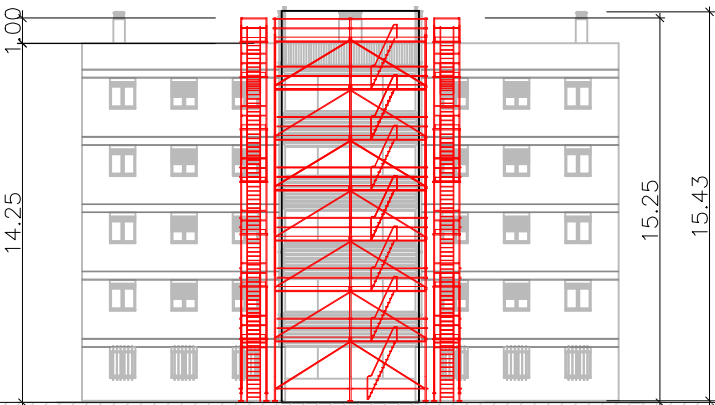
ALÇAT E 1/300
