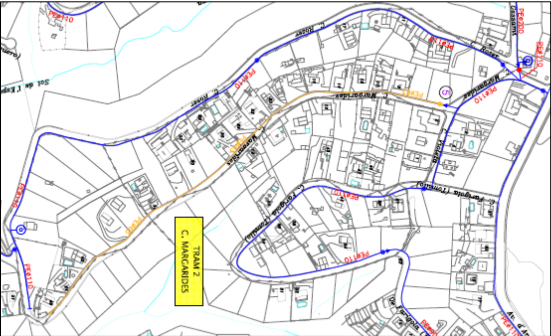
Figura 2. Plànol objecte de l'actuació
