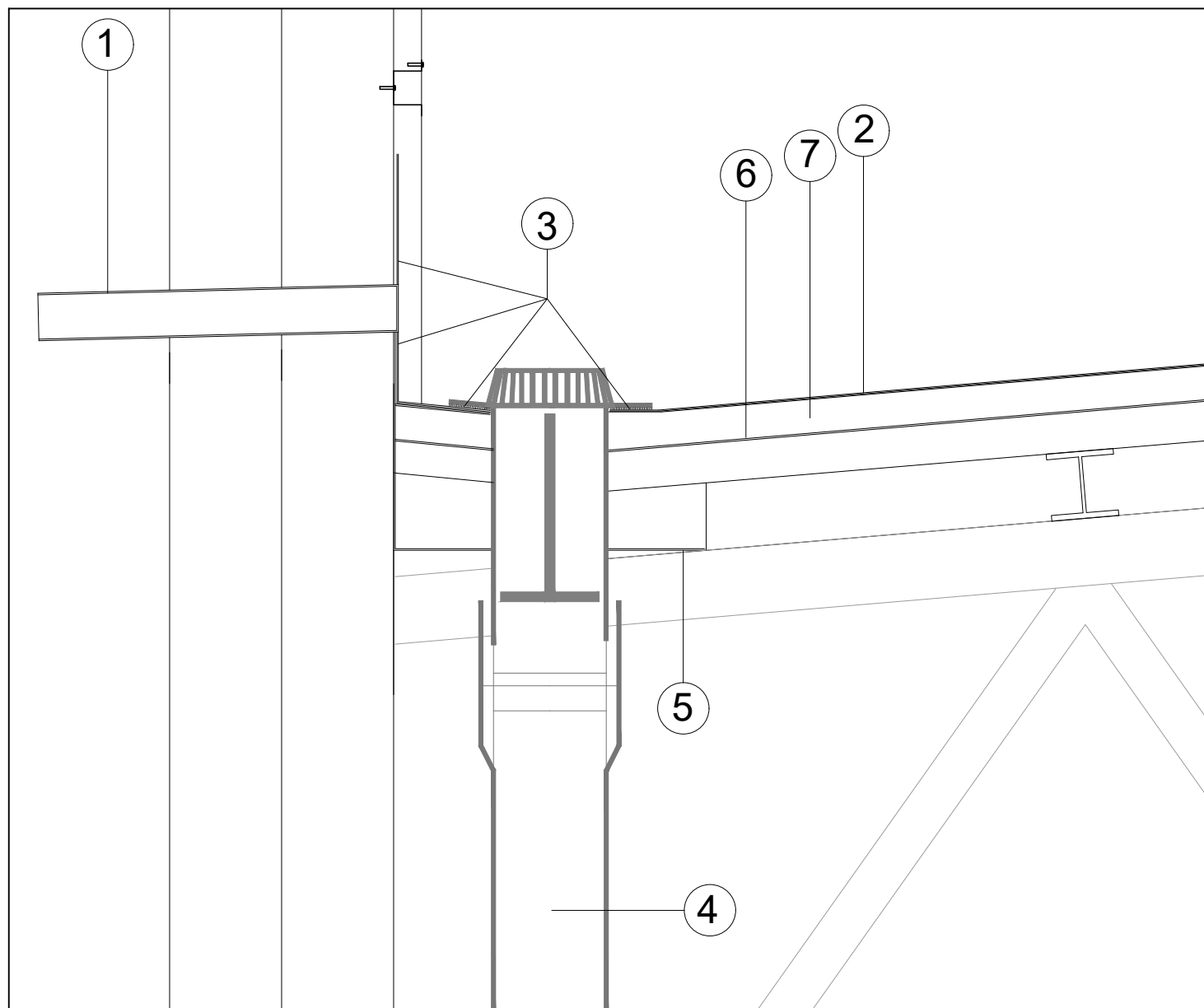
D1- Gargola seguridad sumidero y canalón
