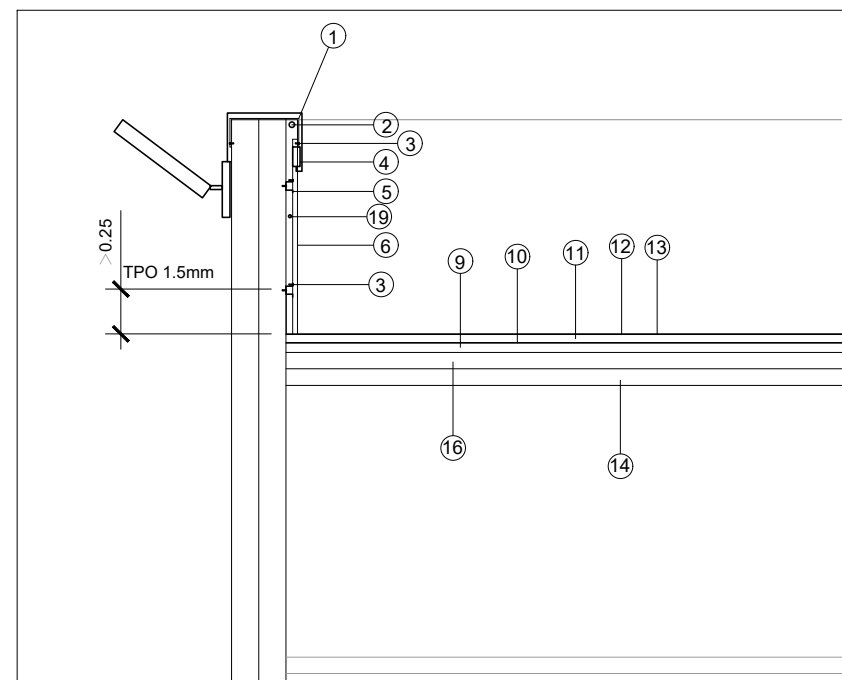
D1-ENCUENTRO CUBIERTA-CANLÓN-MURO
