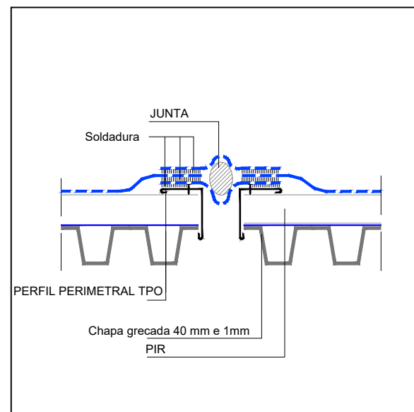
D4- DETALLE JUNTA DE DILATACIÓN
