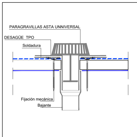
D3- DETALLE DESAGÜE CANALÓN
