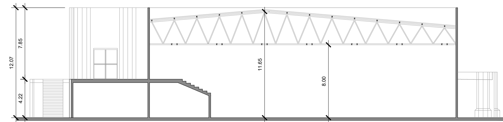
SECCIÓN C-C'
