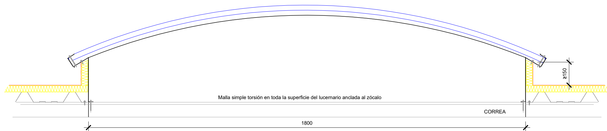
SECCIÓN TRANSVERSAL Lucernarios abovedados de policarbonato multicelular de 16mm radio arco 2m
