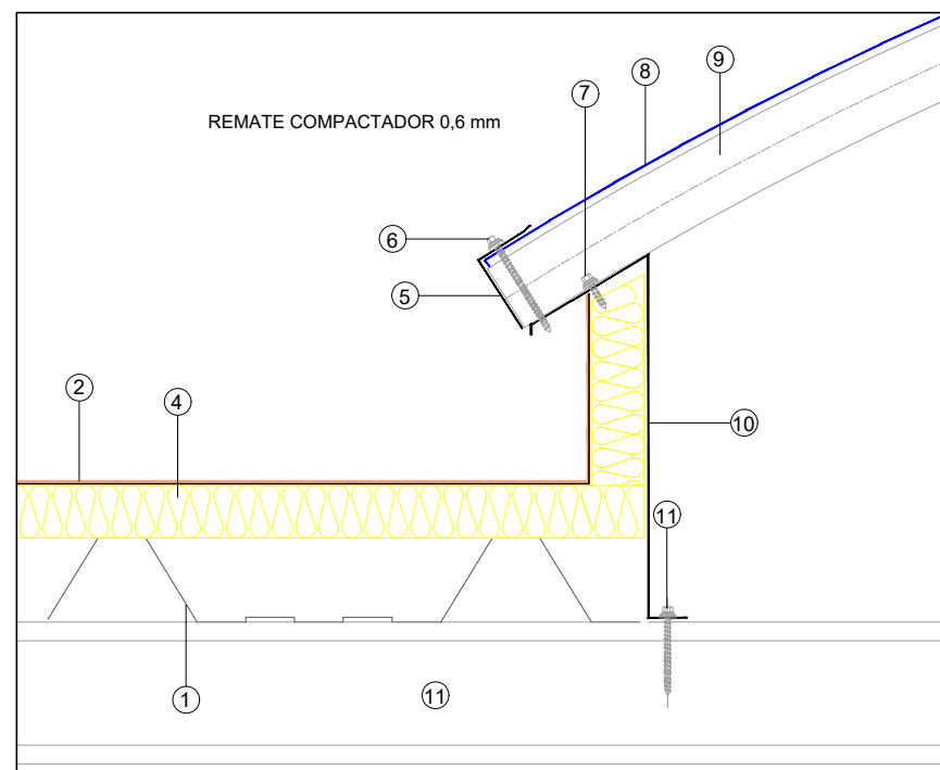
DETALLE ENCUESTRO LUCERNARIO CON LA CUBIERTA DECK TPO
