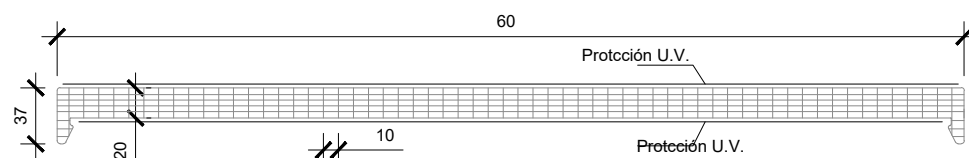
DETALLE PLACA POLICARBONATO MULTICELULAR 20MM
