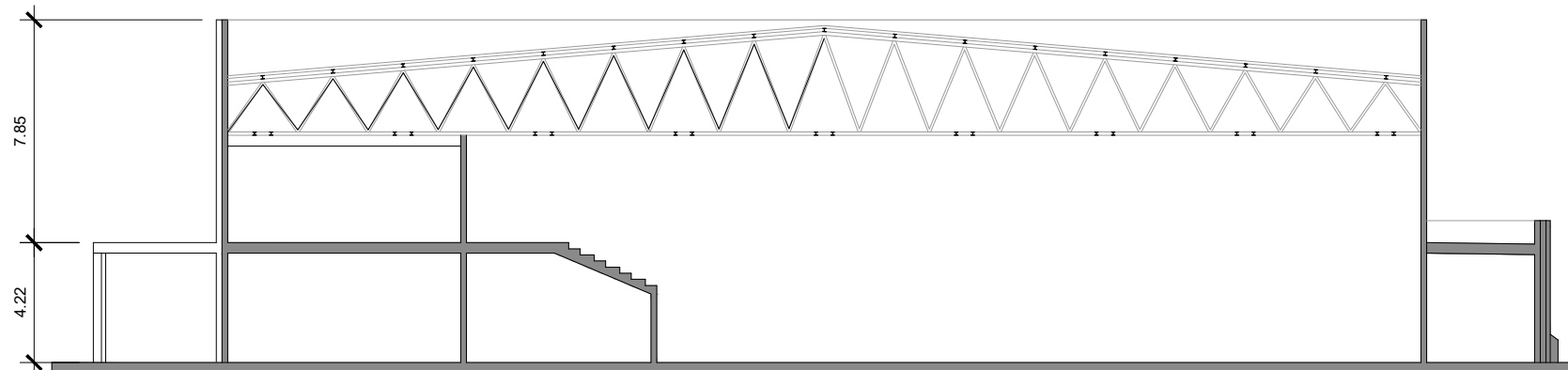
SECCIÓN B-B'
