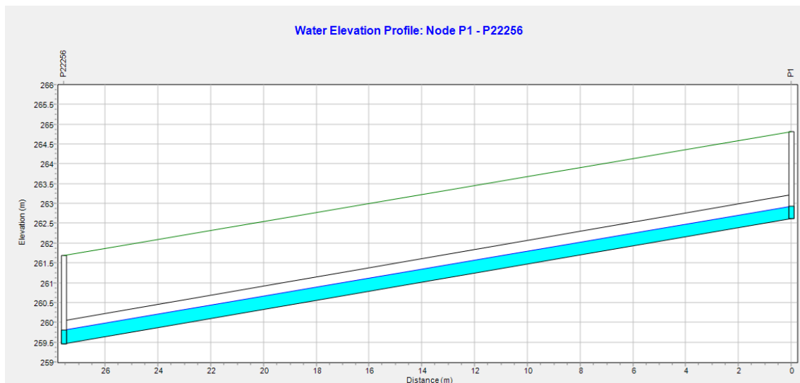
Figura 12. Perfil longitudinal del tram T3 proposat.
