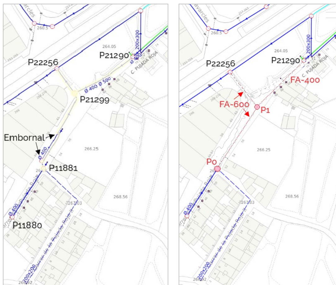
Figura 8. Estat actual, xarxa a eliminar (esquerra). Estat projectat, substitució de xarxa (dreta)
