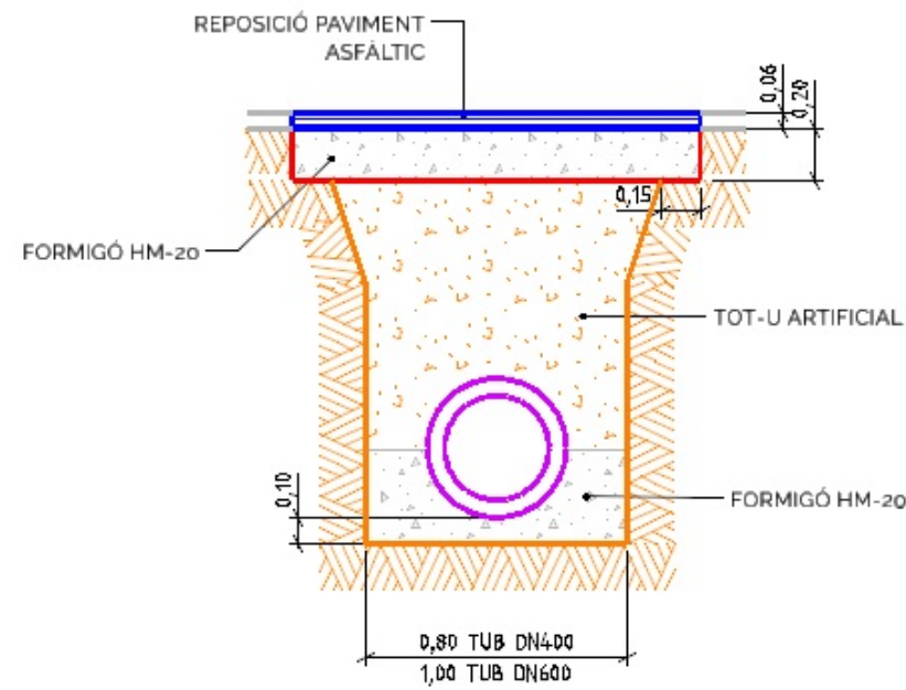
RASA PAVIMENT ASFÀLTIC
