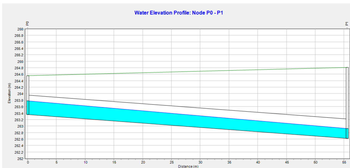
Figura 11. Perfil longitudinal del tram T2 proposat.
