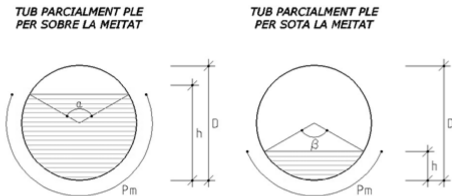
Figura 1. Perímetre mullat en tubs parcialment plens.
