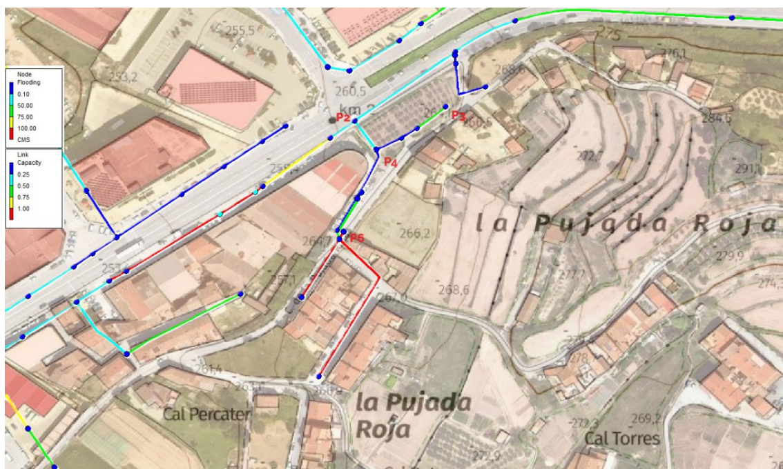
Figura 8. Situació actual amb un escenari amb pluja T10
