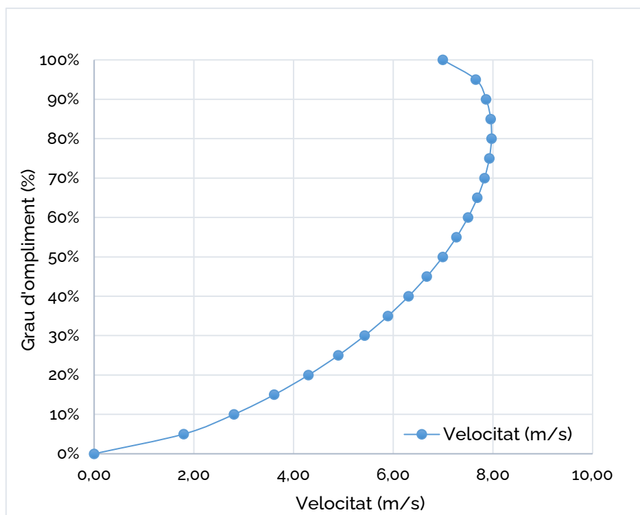
Figura 7. Corba característica de la velocitat del tram T3 proposat.
