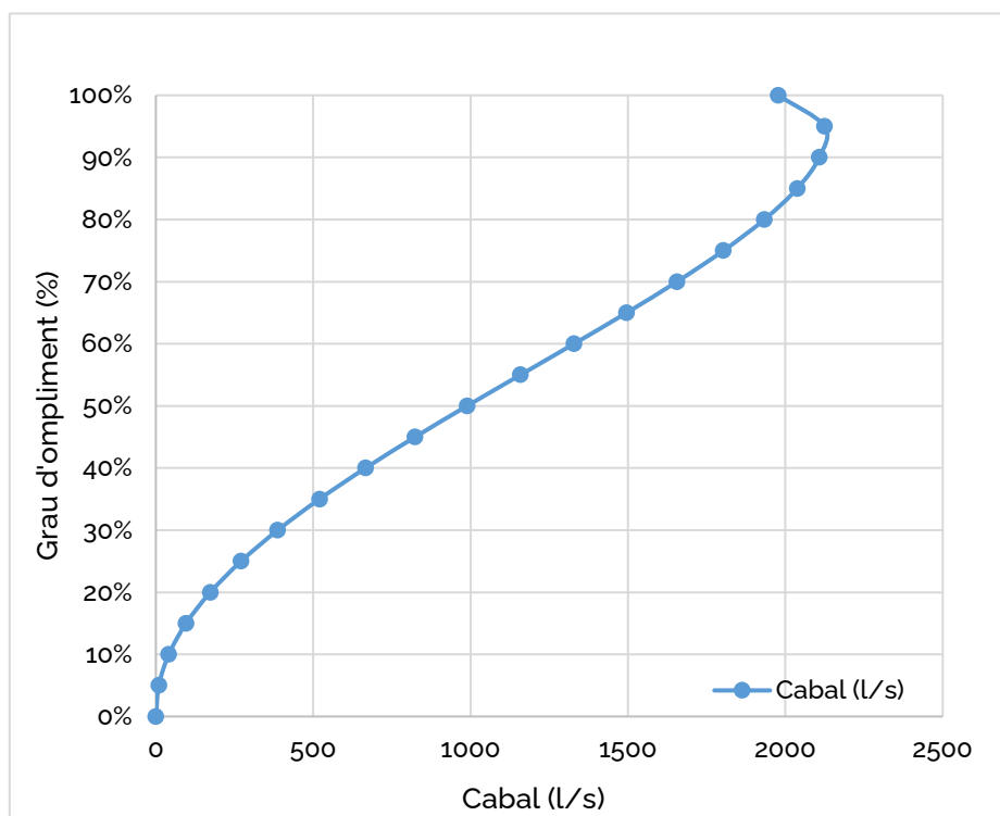
Figura 4. Corba característica de cabal del tram T2 proposat.
