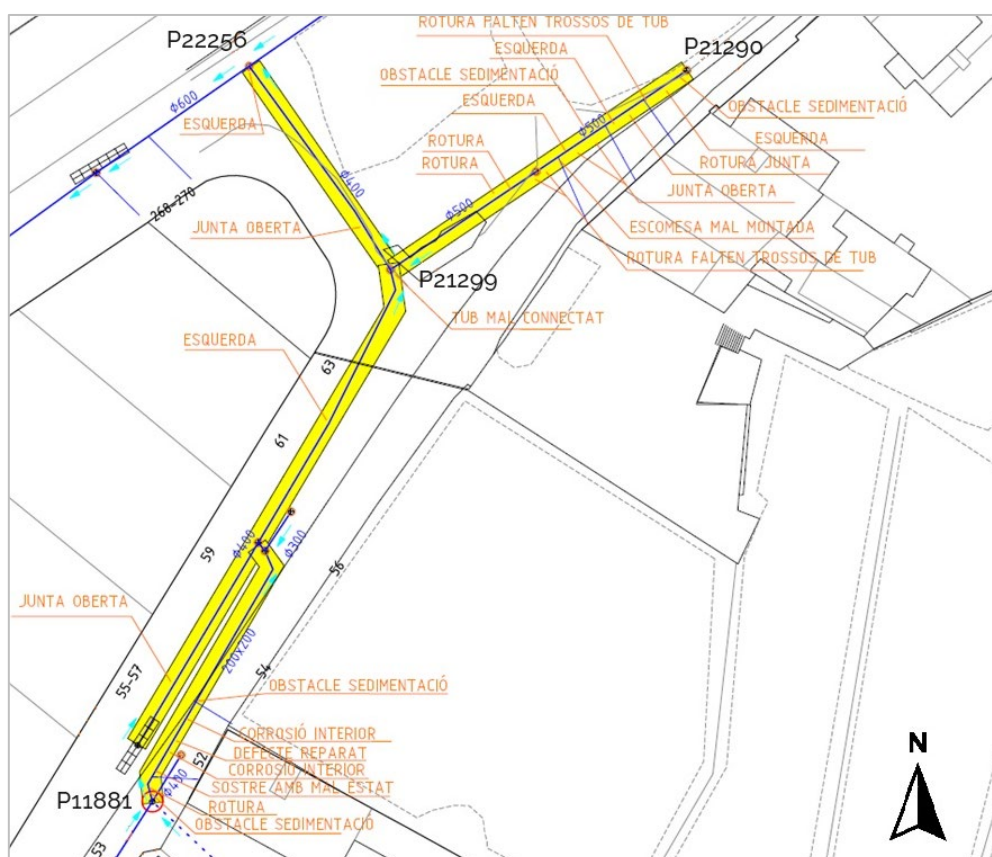
Figura 1. Resultats de les inspeccions amb pas de càmera realitzades l'any 2012
