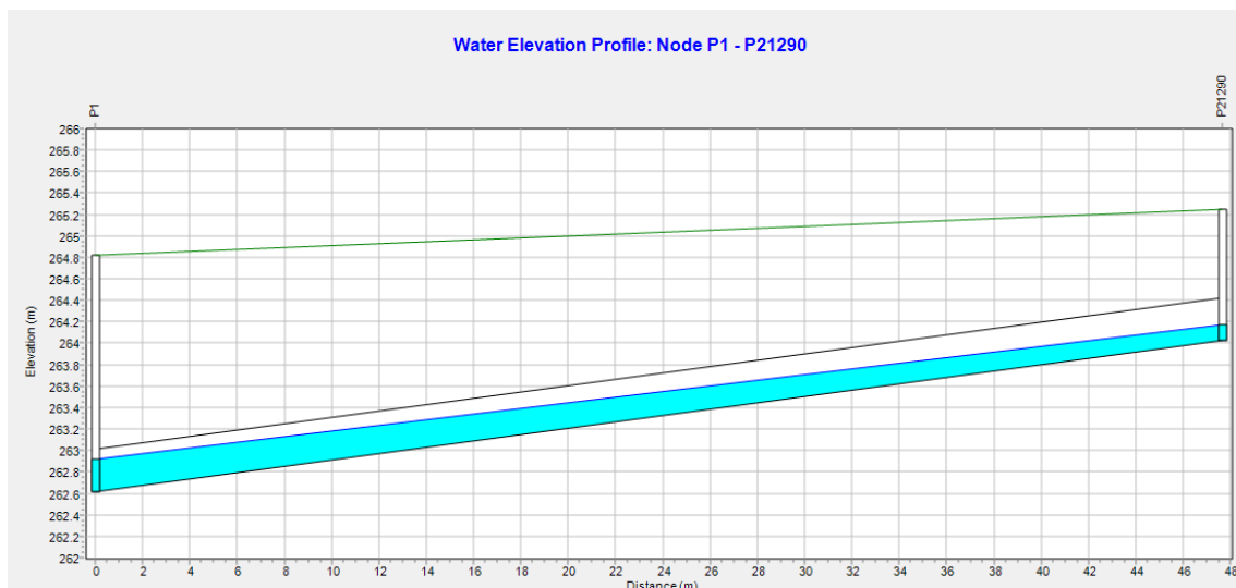
Figura 10. Perfil longitudinal del tram T1 proposat.
