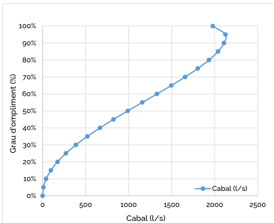
Figura 6. Corba característica de cabal del tram T3 proposat.
