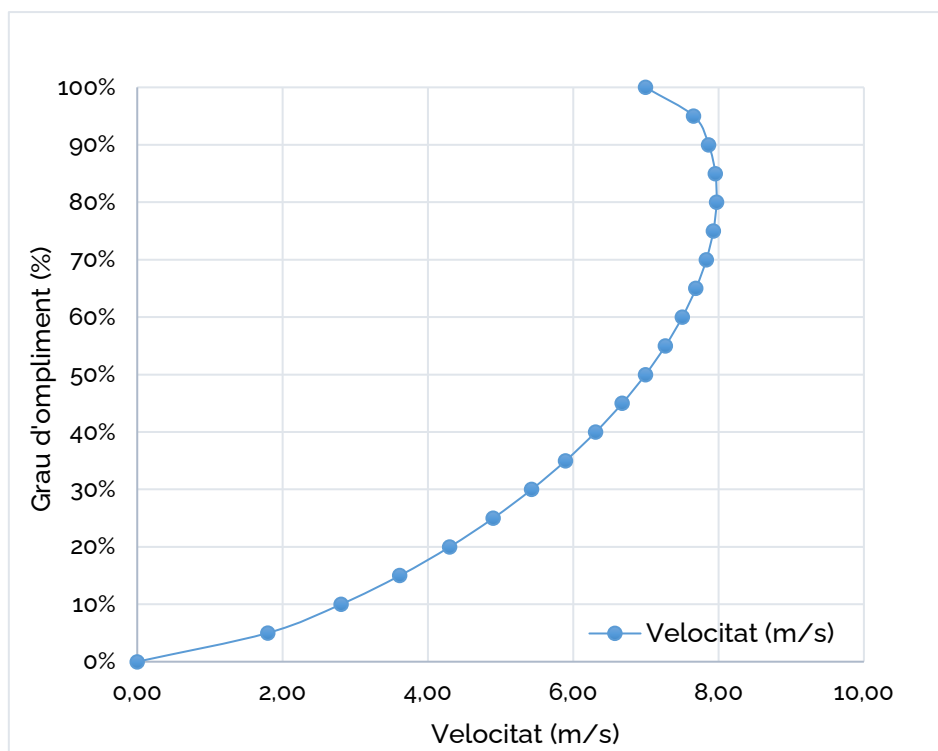
Figura 5. Corba característica de la velocitat del tram T2 proposat.
