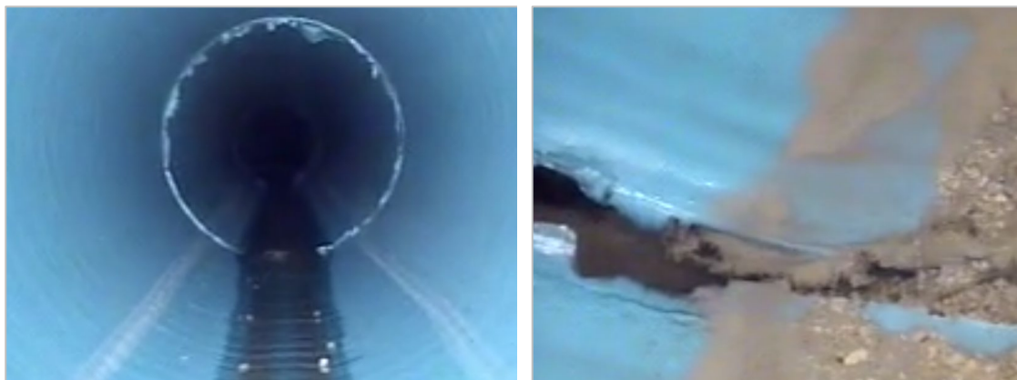
Figura 5. Col·lector P21290-P21299, 1r tram PEC-400, esquerra radial en junta
