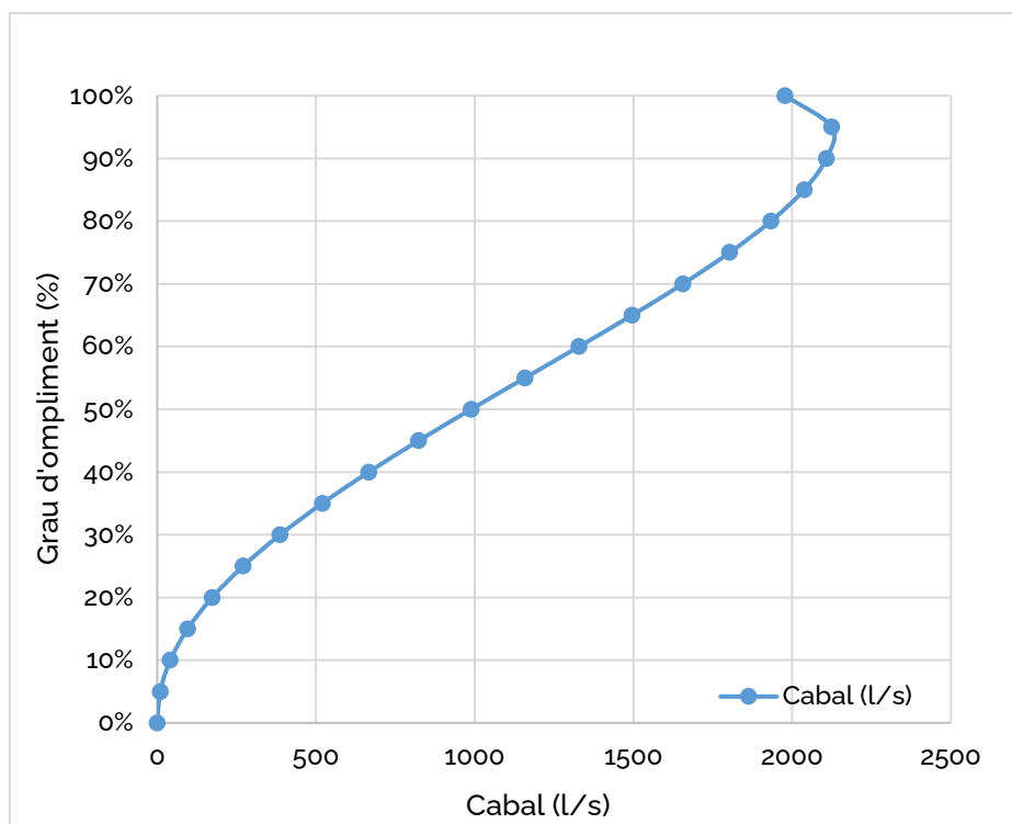
Figura 2. Corba característica de cabal del tram T1 proposat.
