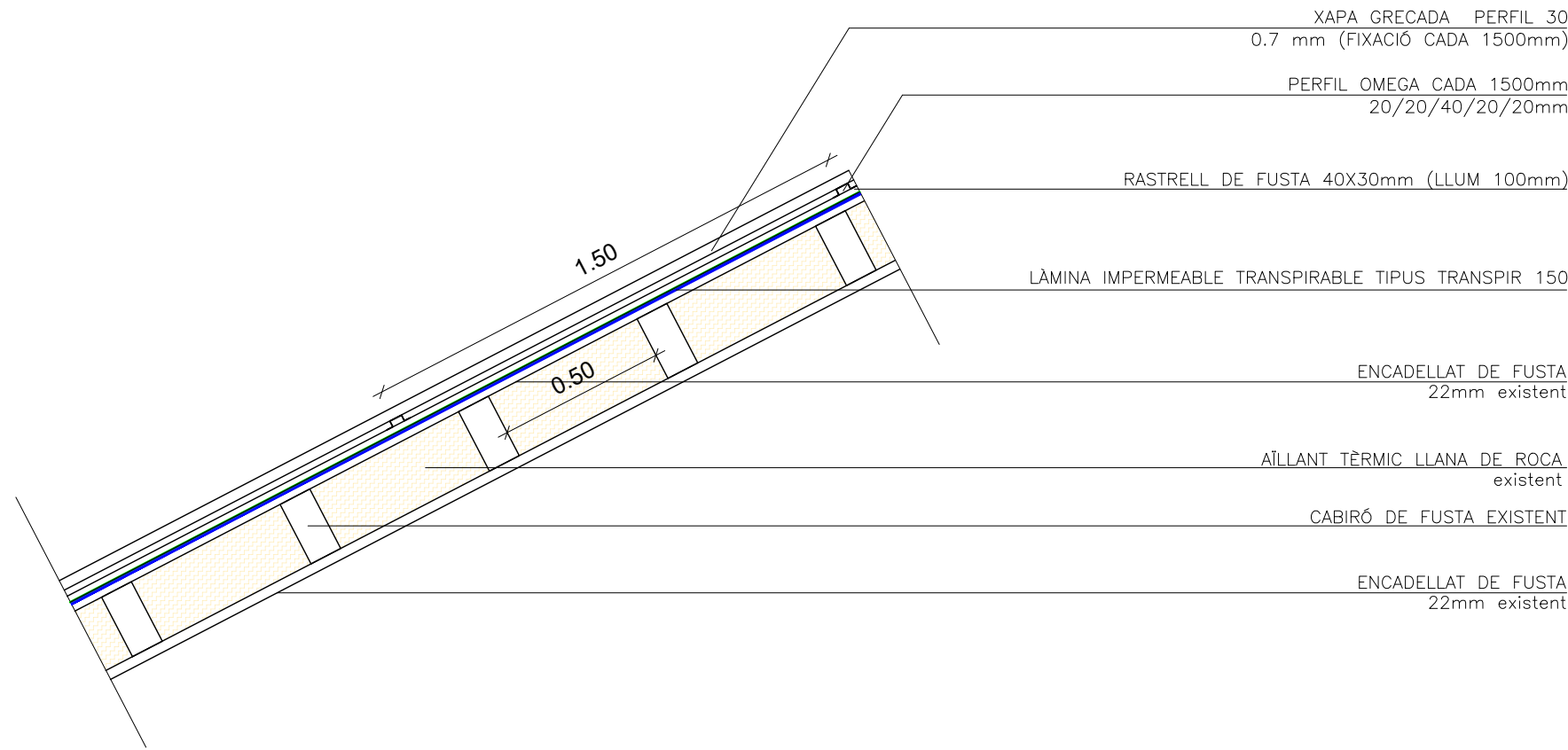
DETALL COBERTA LONGITUDINAL
