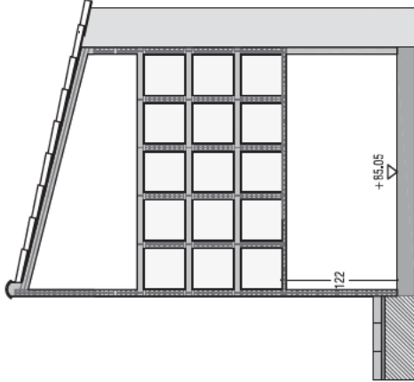
SECCIÓ TRANSVERSAL
