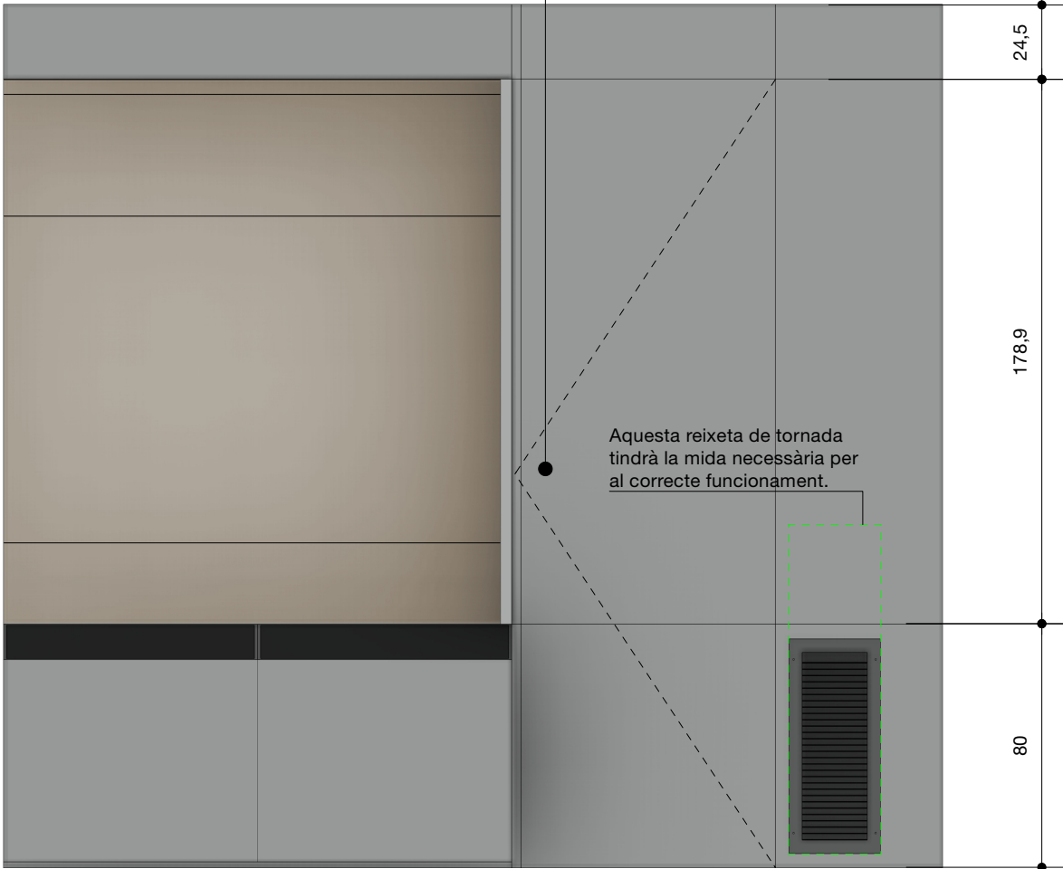
Alçat B - B
