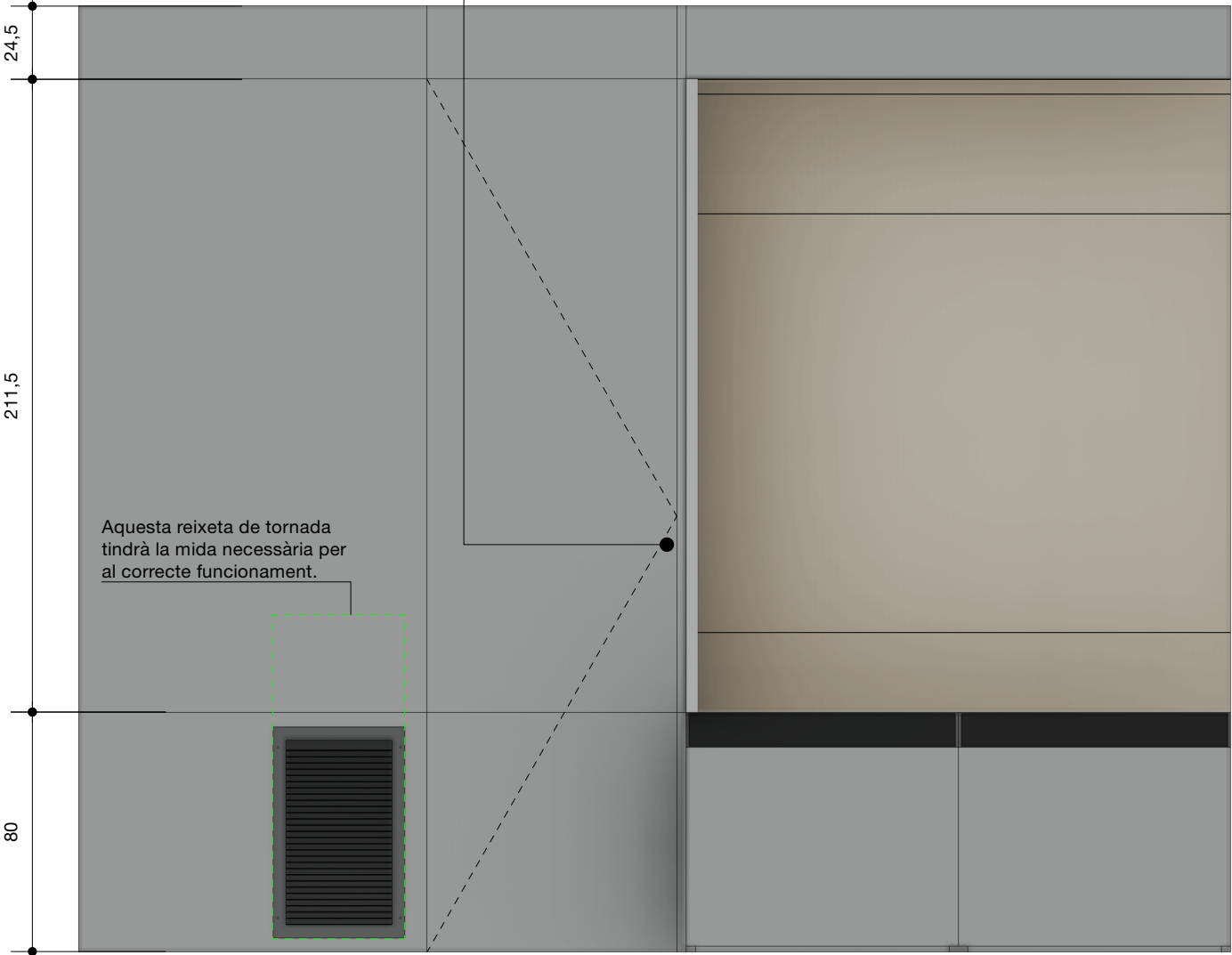
Alçat A - A
