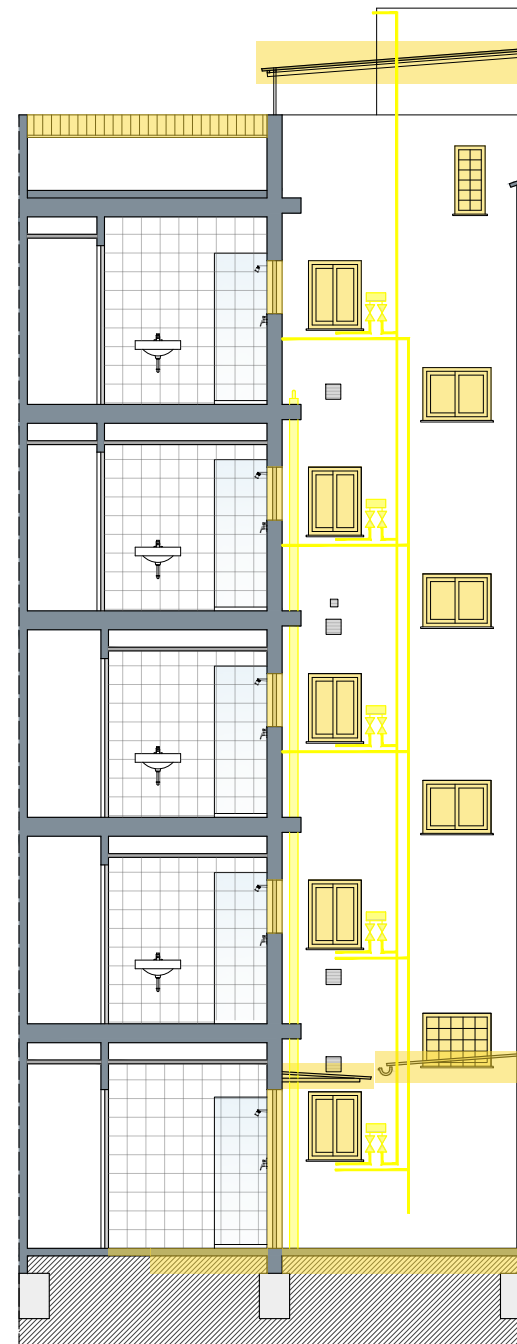
SECCIÓ B-B'
