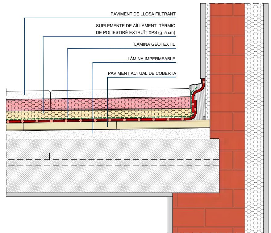
3 DETALL FAÇANA i TERRAT
