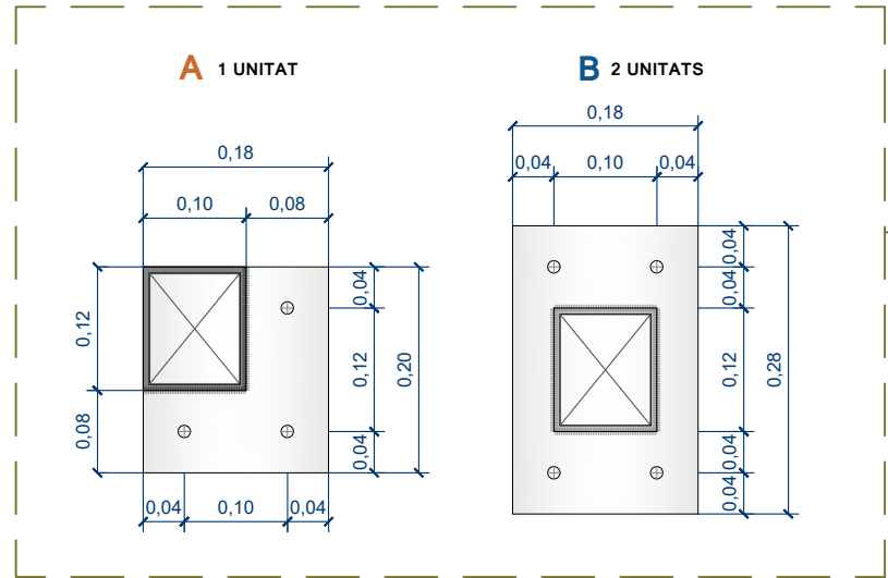
DETALL PLACAS DE ANCORATGE
