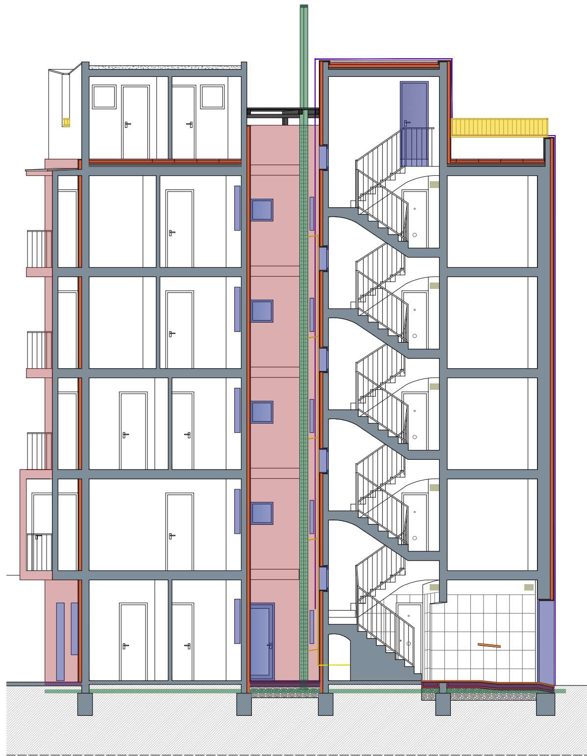
SECCIÓ LONGITUDINAL e=1:100
