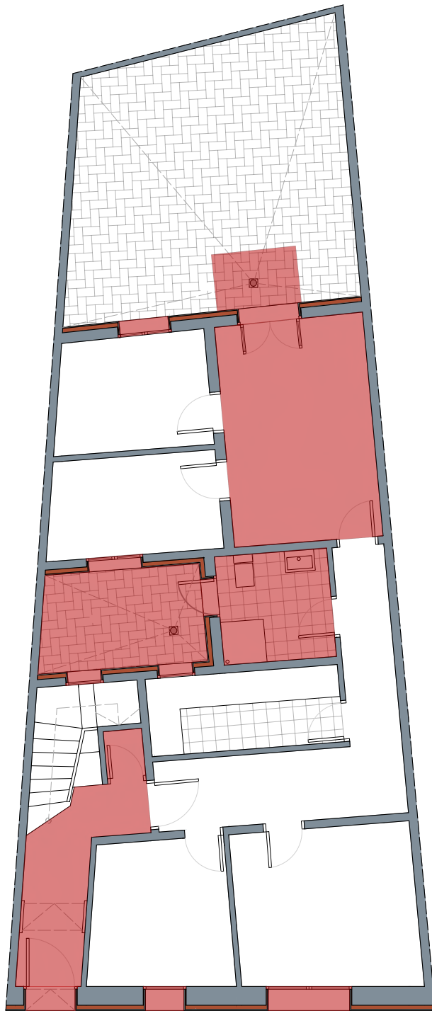
PLANTA BAIXA
