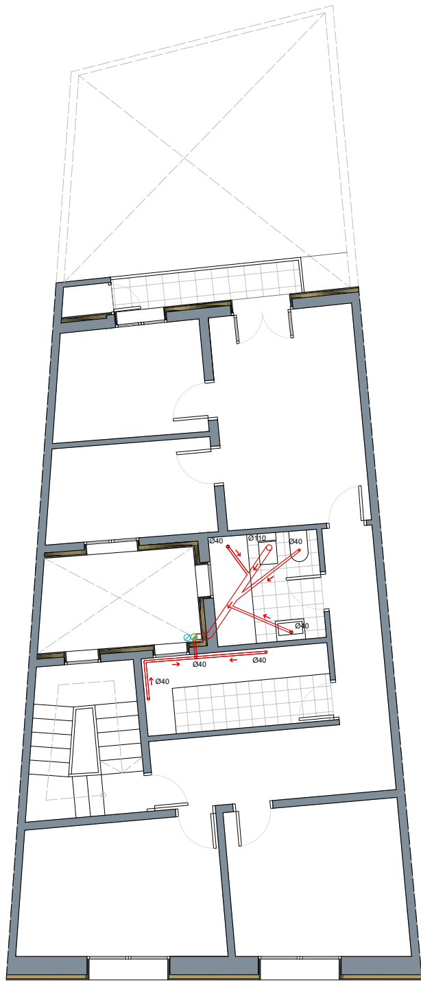
PLANTA TIPUS
