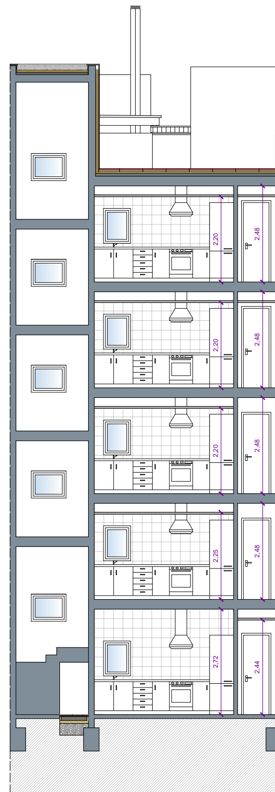
SECCIÓ D-D'
