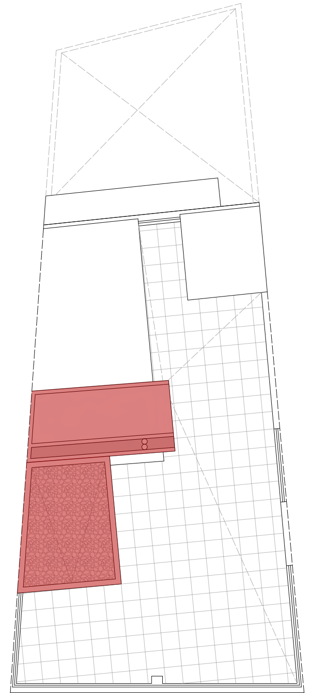
PLANTA COBERTA
