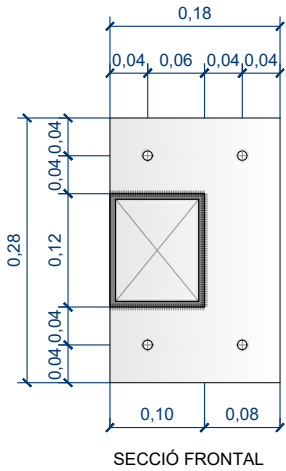
SECCIÓ FRONTAL
