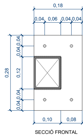
DETALL PLETINES D'ACER PER A UNIÓ DE TUB 120x100x6 A MUR
