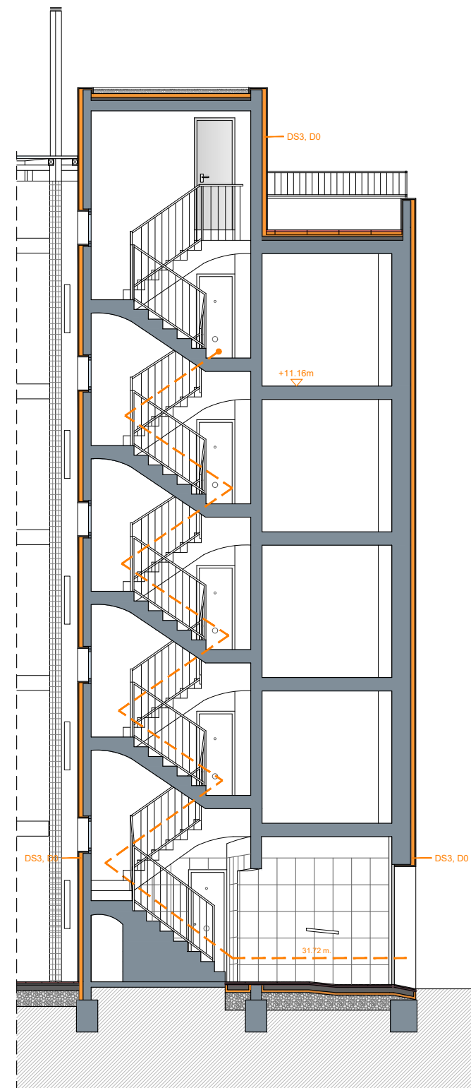
SECCIÓ
