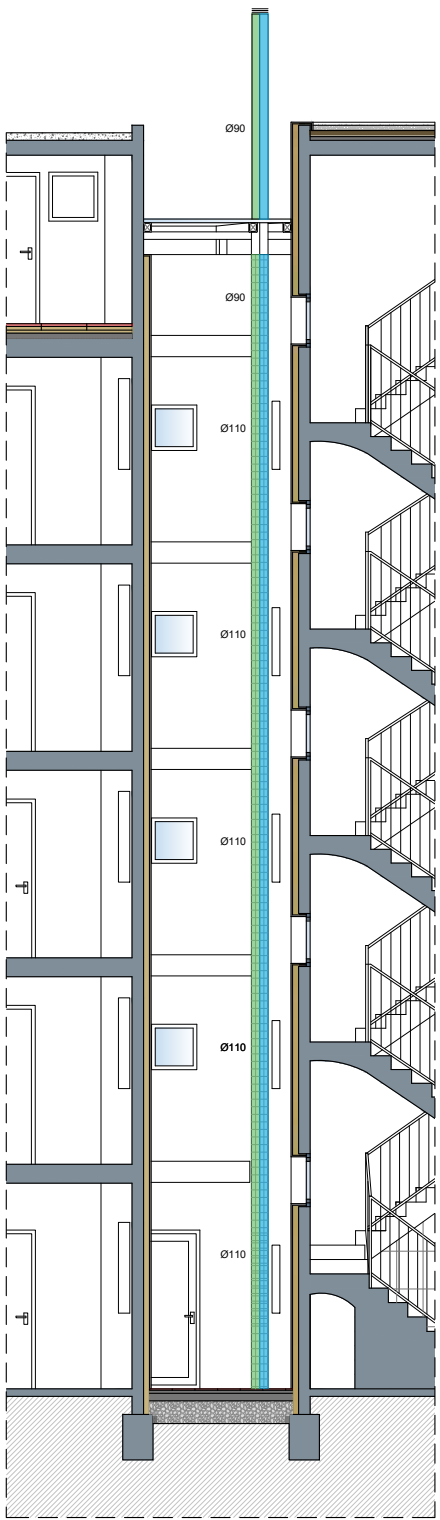
SECCIÓ PER PATI
