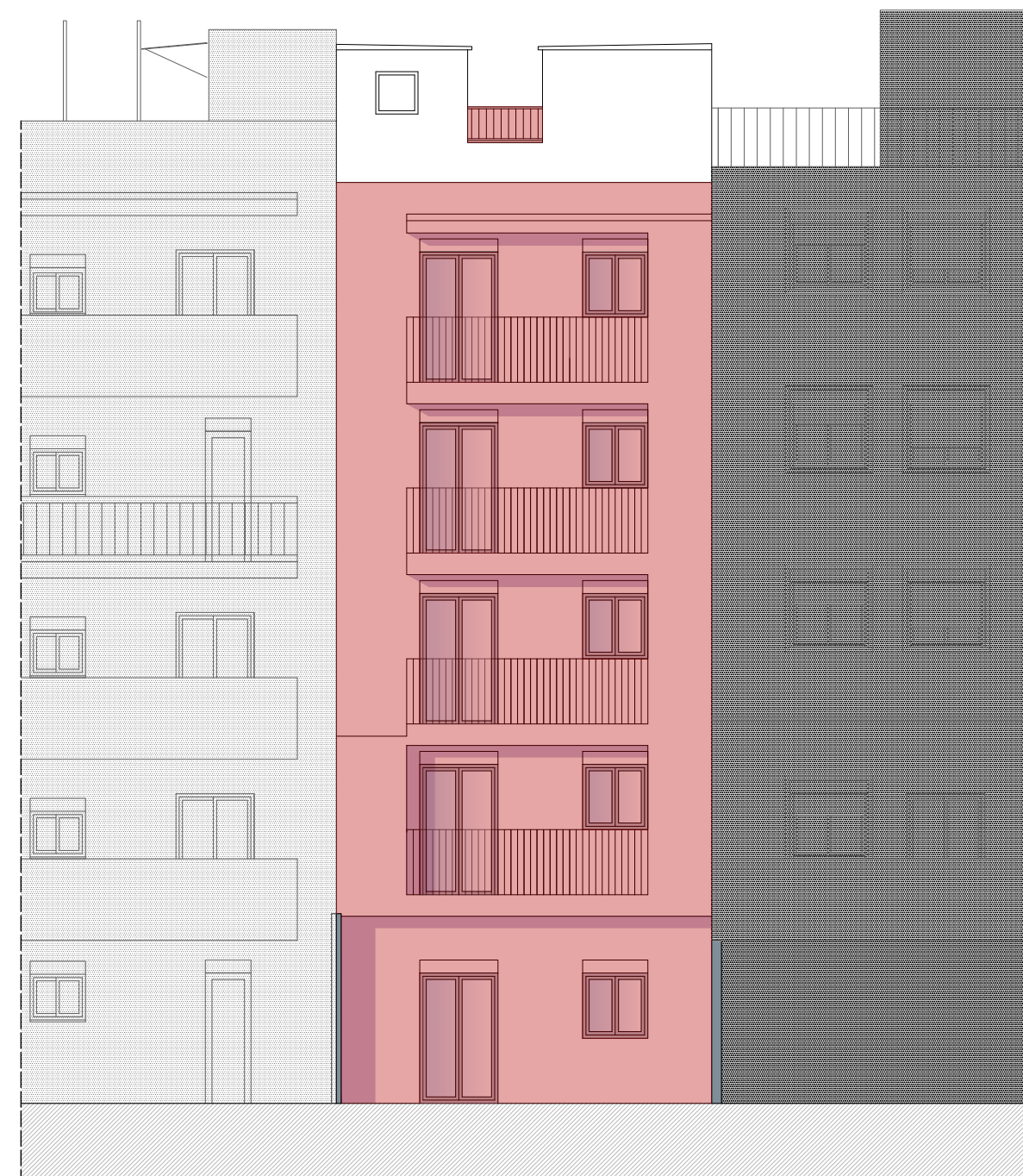
FAÇANA A PATI D' ILLA
