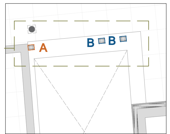
PLANTA GENERAL PLACAS DE ANCORATGE
