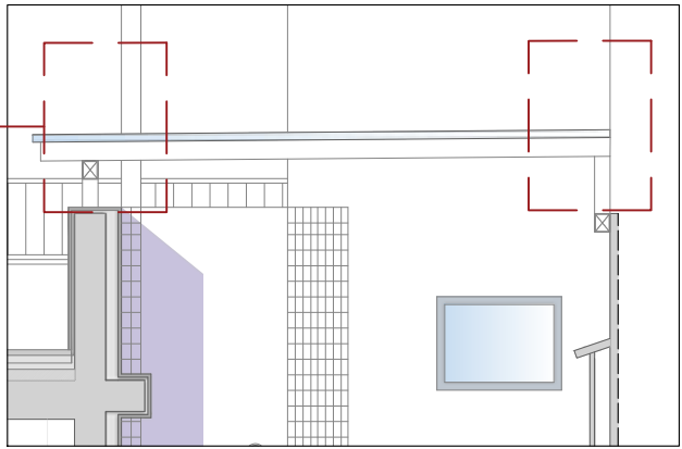
SECCIÓ LATERAL
