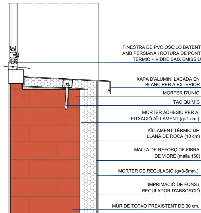
2 DETALL ENCONTRE FAÇANA AMB FUSTERIA
