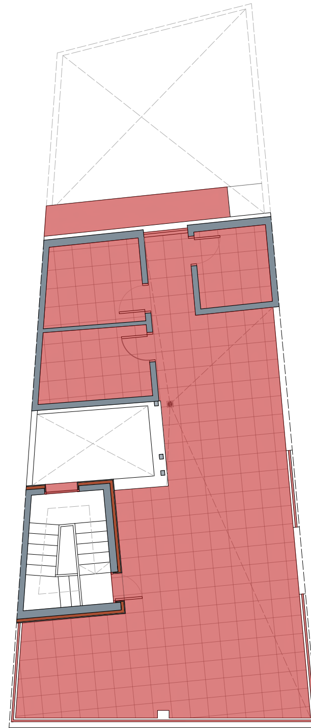
PLANTA TERRAT
