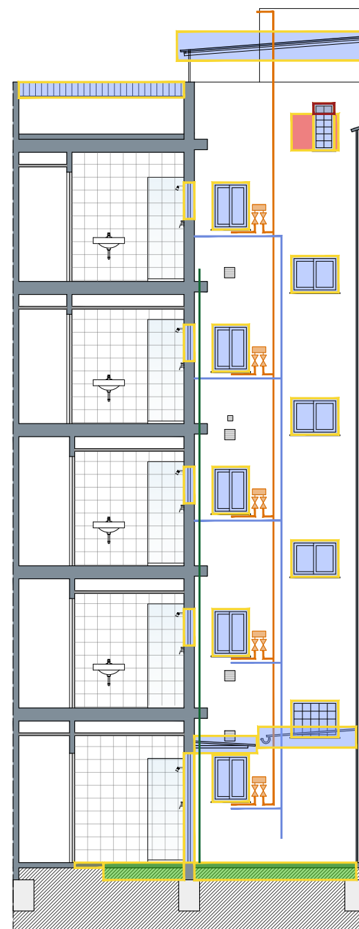
SECCIÓ B-B'
