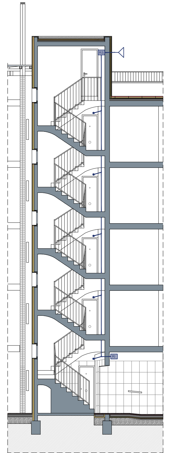
SECCIÓ PER PATI
