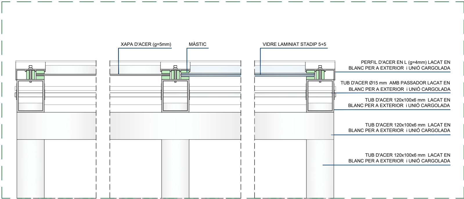
DETALL LLUERNA SECCIÓ FRONTAL
