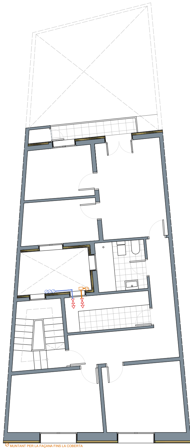
PLANTA TIPUS
