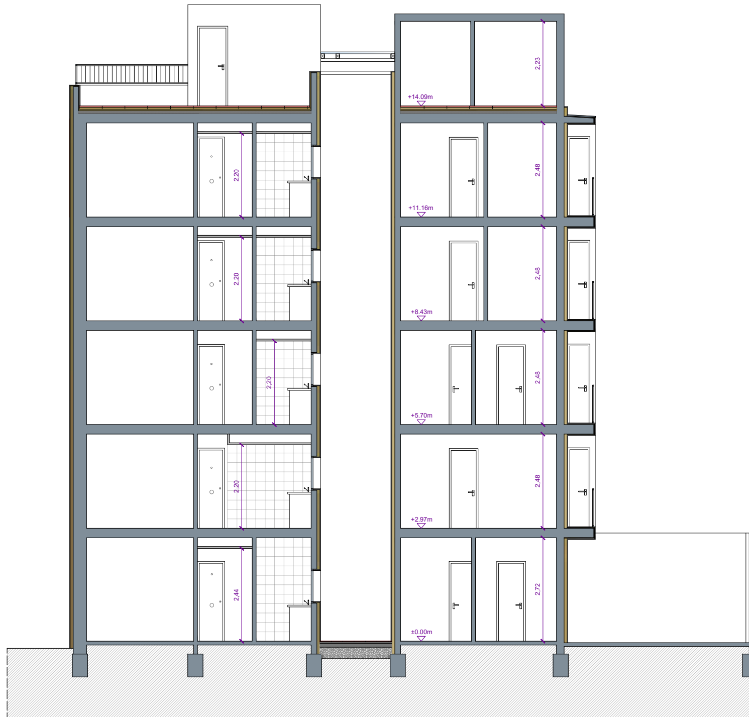
SECCIÓ C-C'
