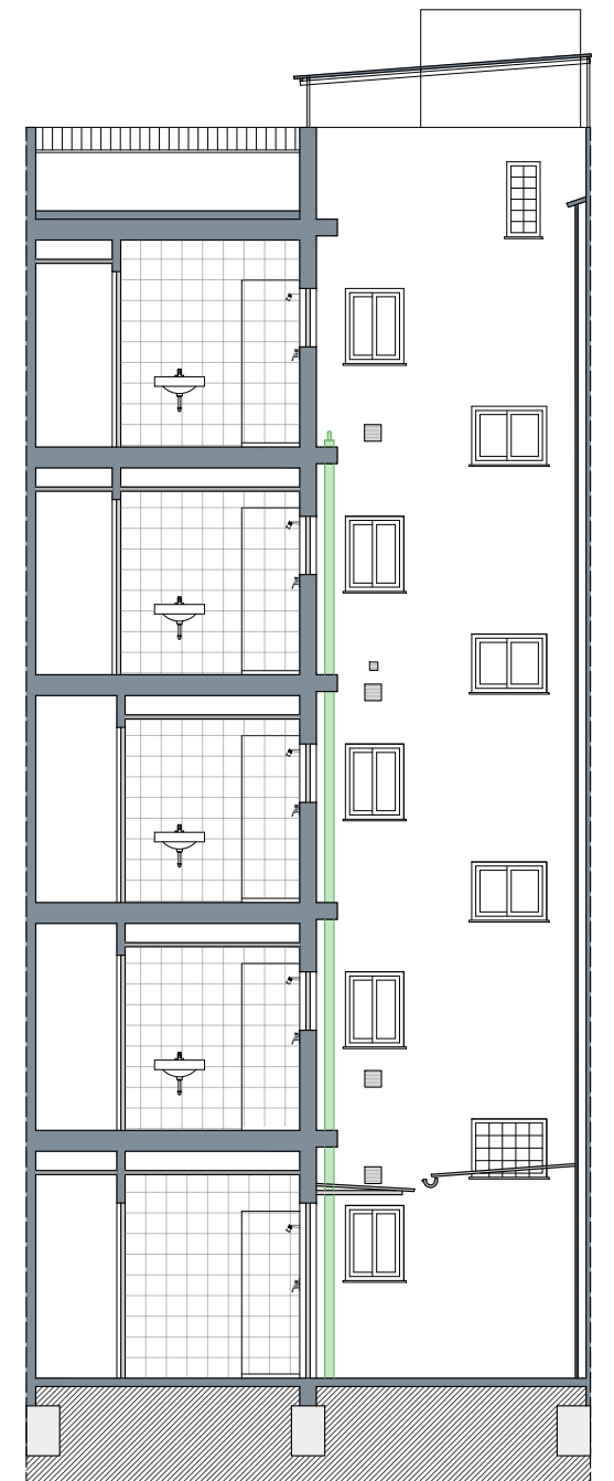
SECCIÓ PER PATI
