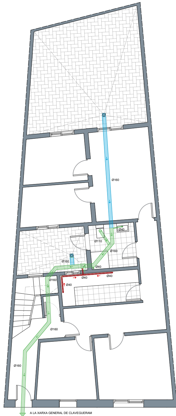
PLANTA BAIXA
