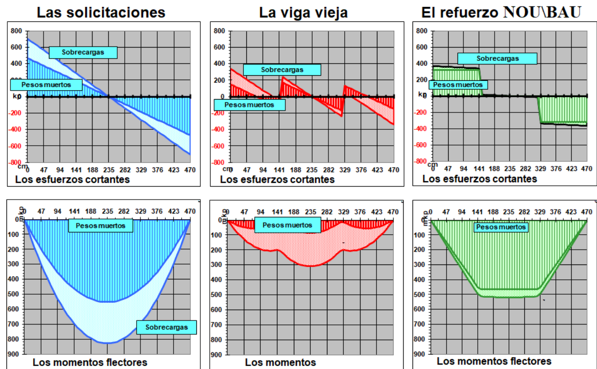
Cálculos hechos con el programa N. B. de elementos finitos para cada viga propuesta.
