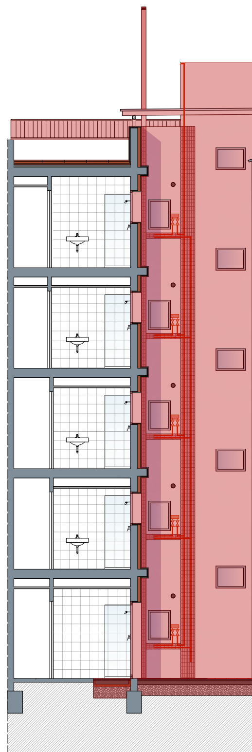
SECCIÓ B-B'
