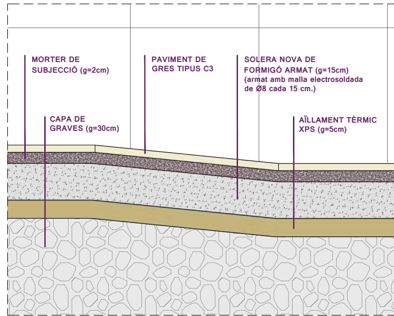
DETALL RAMPA (e=1:10)
