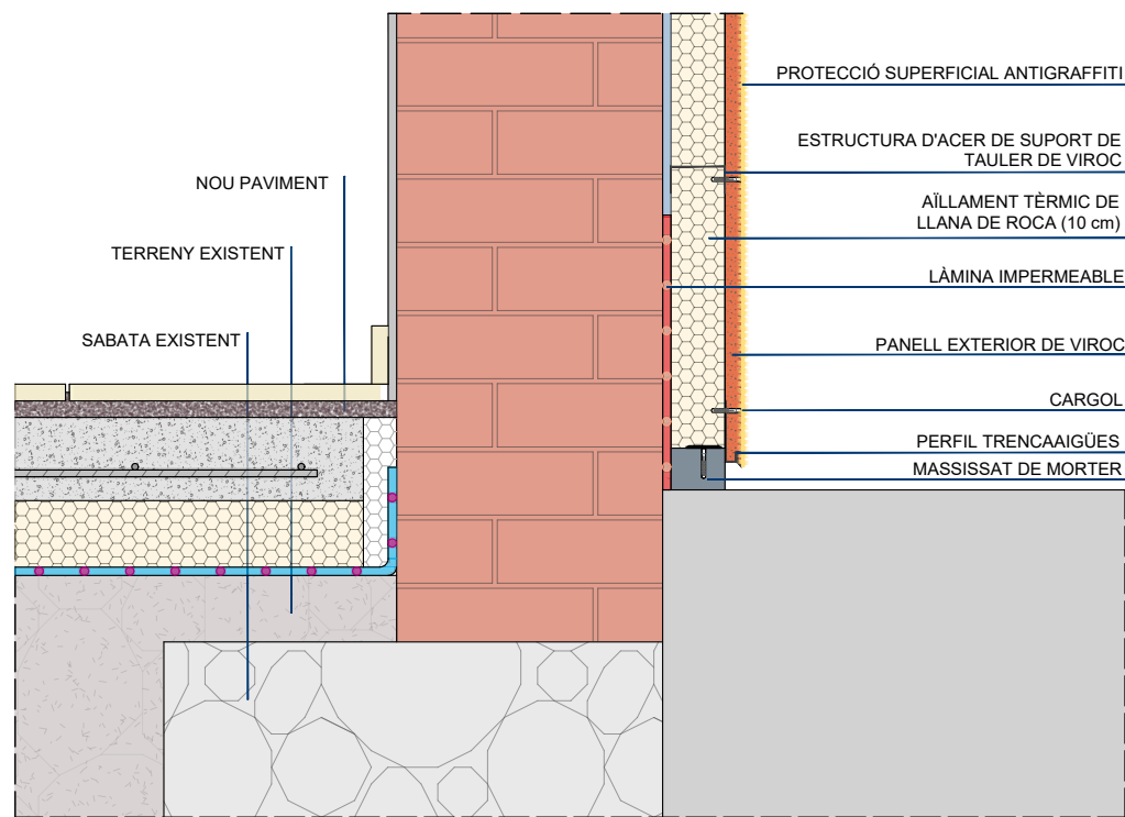
1 DETALL FAÇANA AMB SATE
