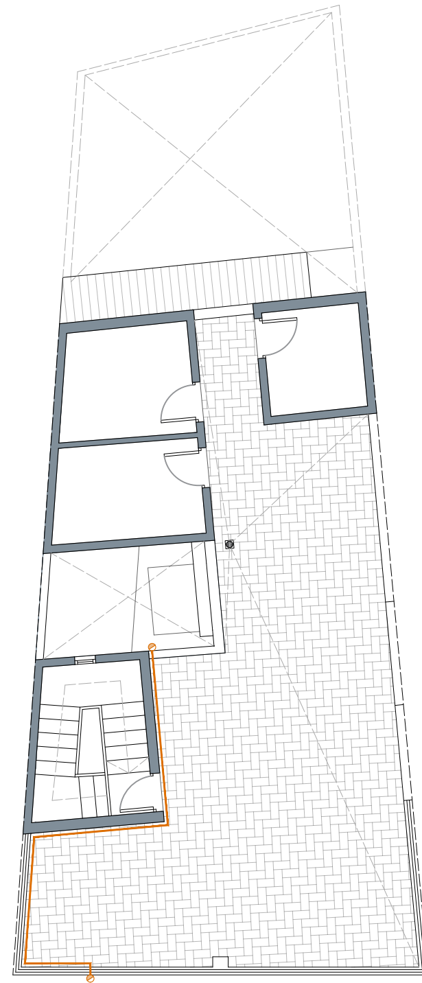
PLANTA TERRAT
