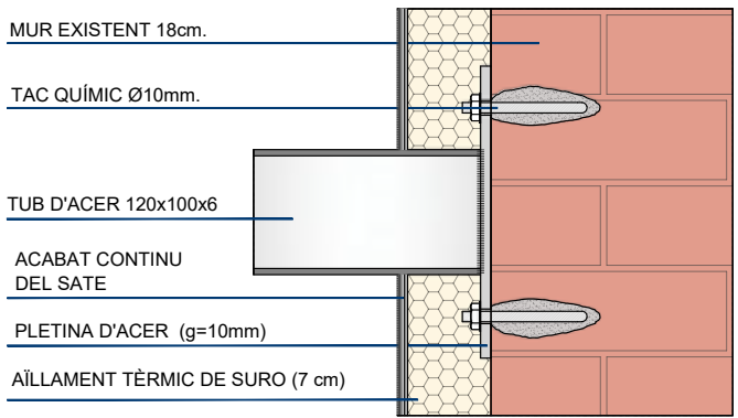
SECCIÓ LATERAL
