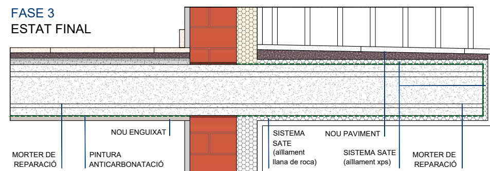
REPARACIÓ BIGUETAS (intervenció parcial)
