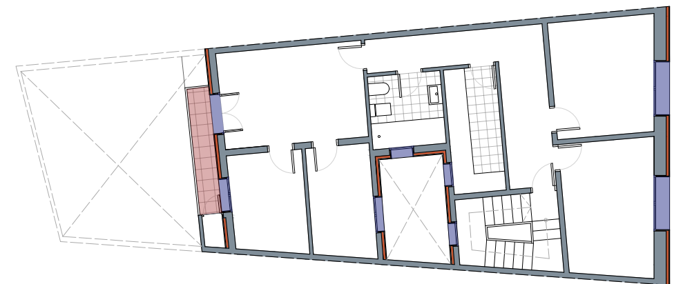
PLANTA TIPUS e=1:150
