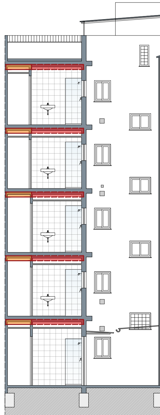
SECCIÓ B-B'
