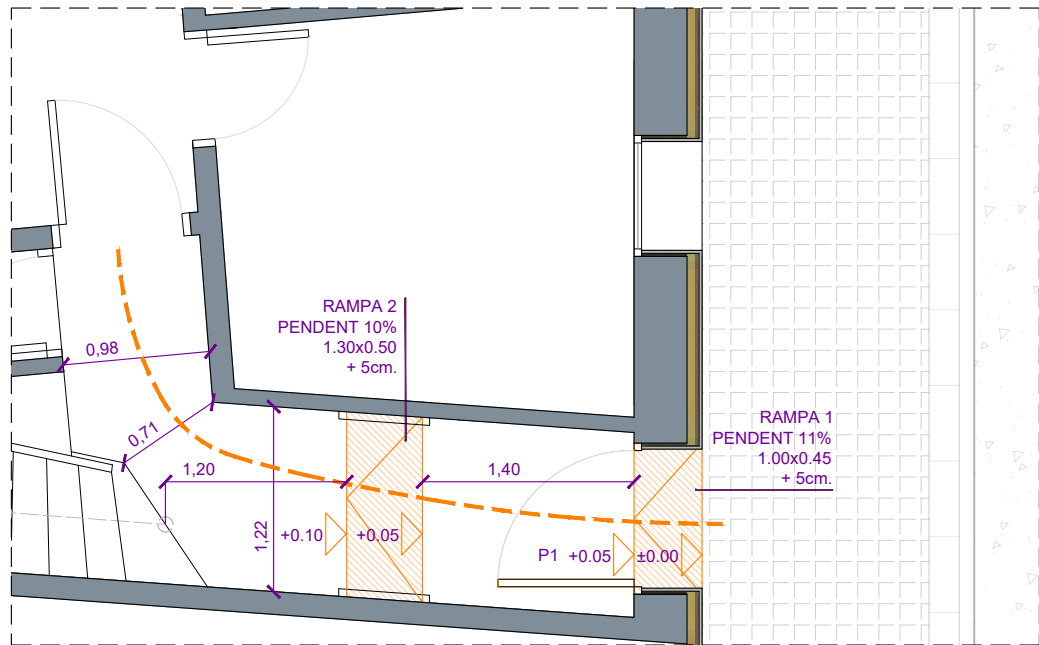
PLANTA (e=1:50)
