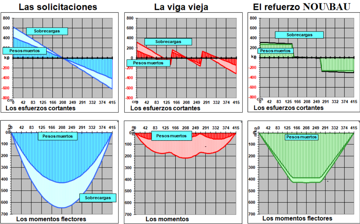
Cálculos hechos con el programa N. B. de elementos finitos para cada viga propuesta.
