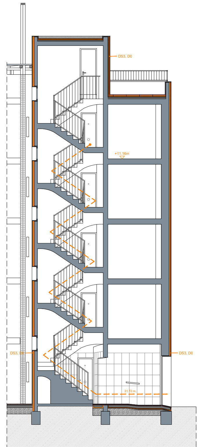
SECCIÓ
