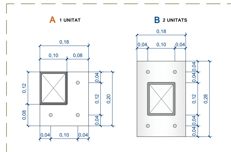
DETALL PLACAS DE ANCORATGE
