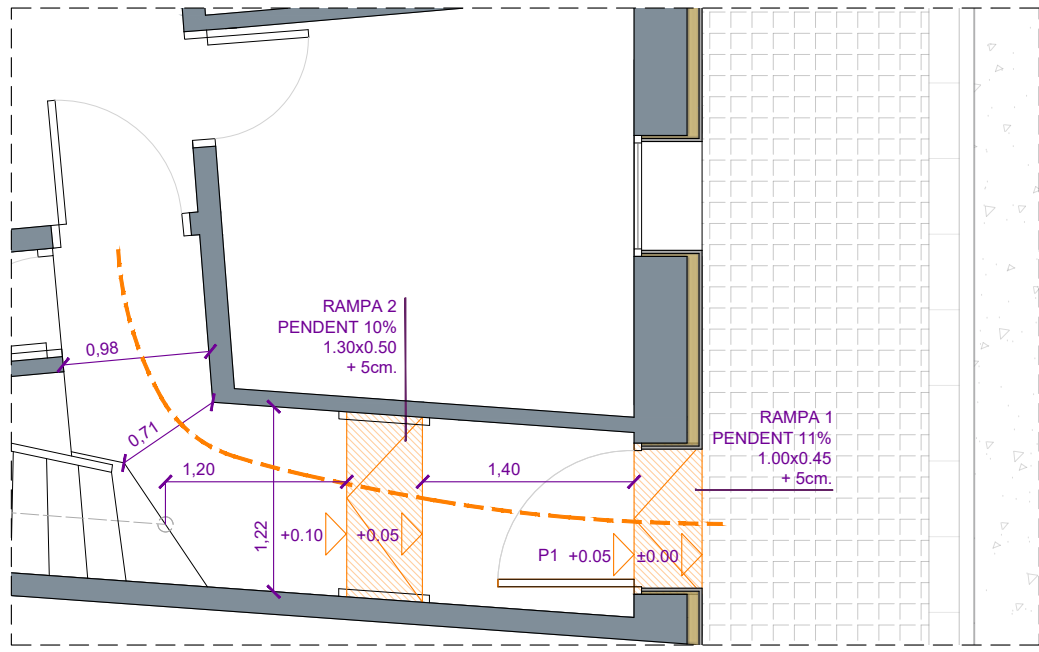
PLANTA (e=1:50)
