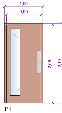
PORTA D'ACCÉS A L'EDIFICI (e=1:50)
