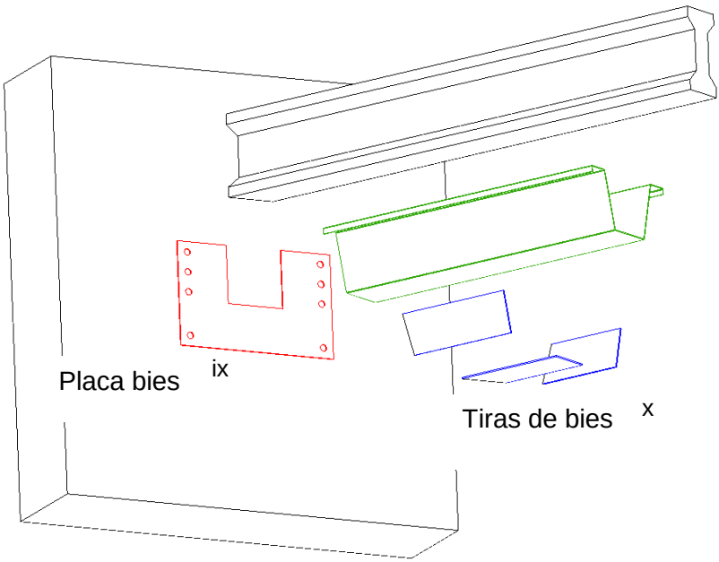
Elementos que conforman el soporte especial
