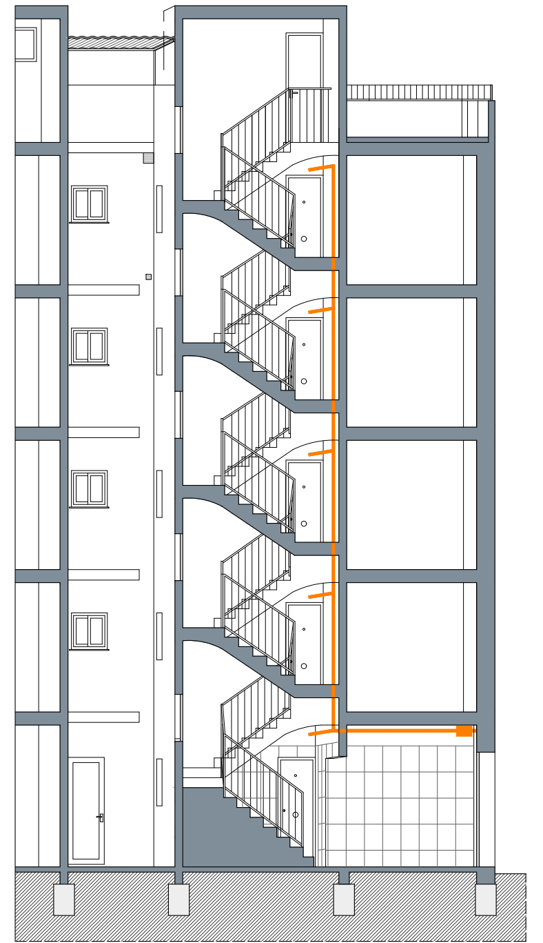
SECCIÓ PEL PATI
