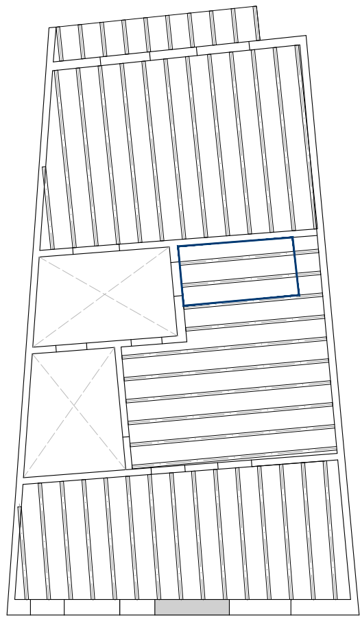
PLANTA FORJAT TIPUS
