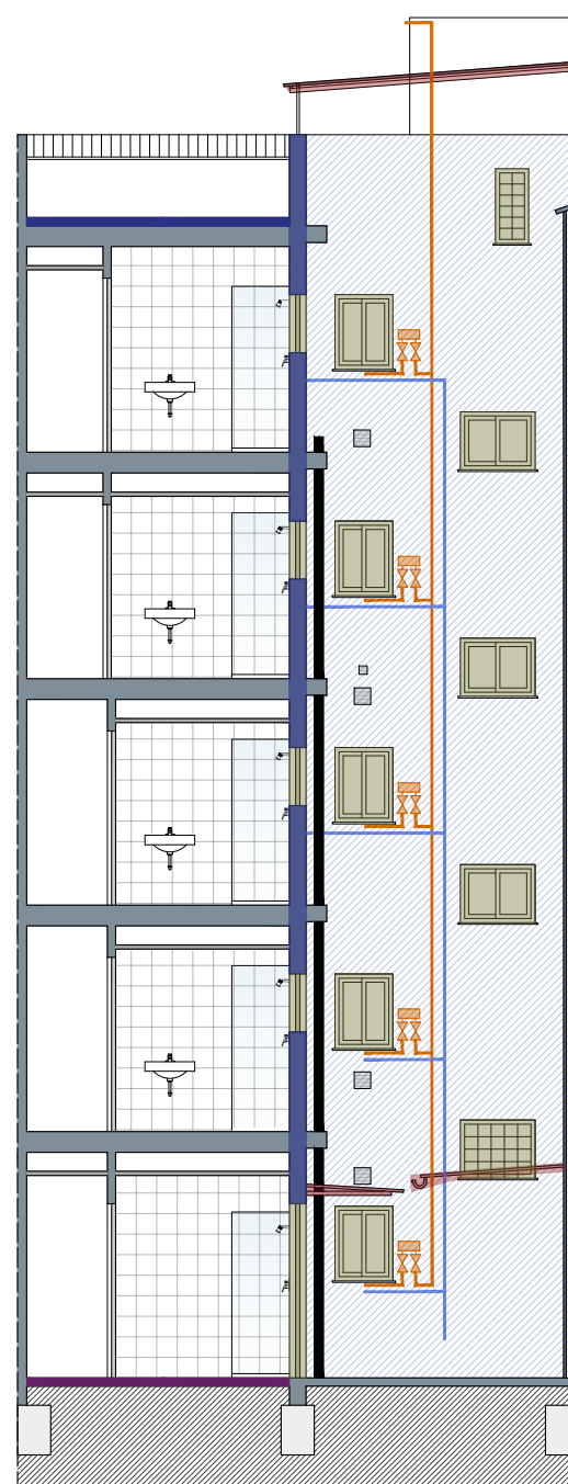
SECCIÓ B-B'
