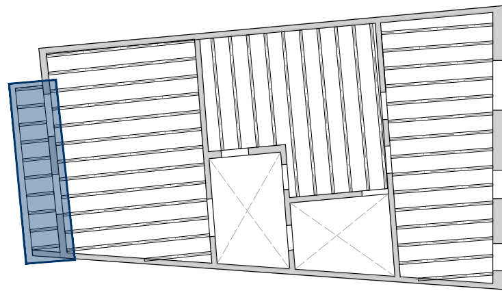
PLANTA FORJAT TIPUS
