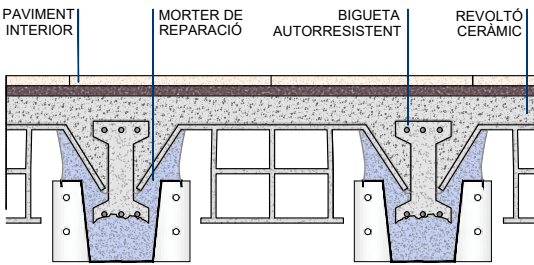
SECCIÓ FRONTAL
