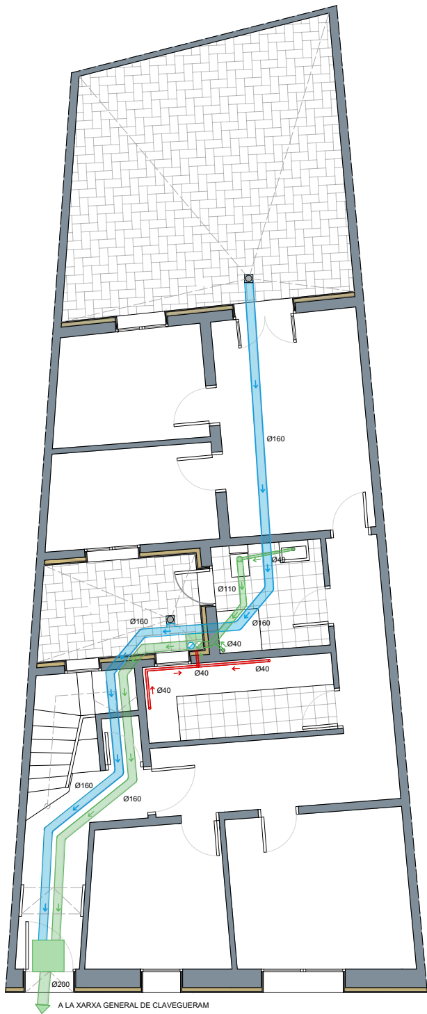
PLANTA BAIXA
