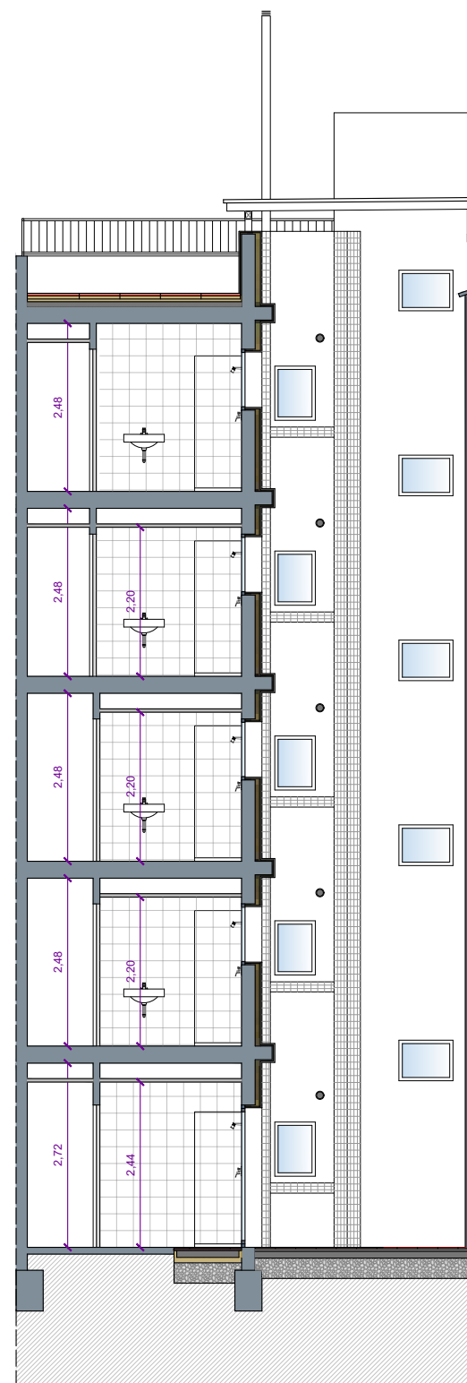
SECCIÓ B-B'
