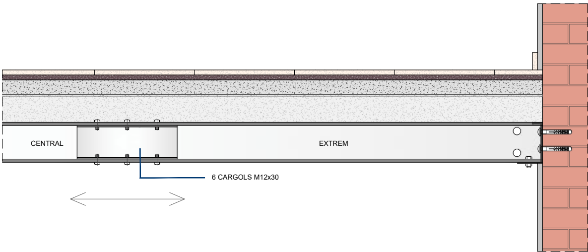
INTERVENCIÓ PROFUNDA (reforç per baix del forjat)
