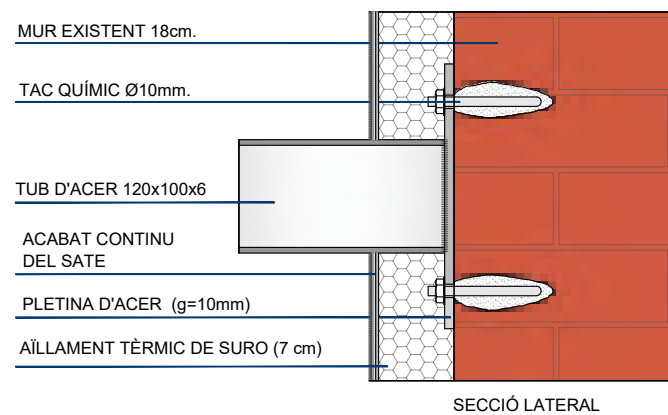
DETALL PLETINES D'ACER PER A UNIÓ DE TUB 120x100x6 A MUR
