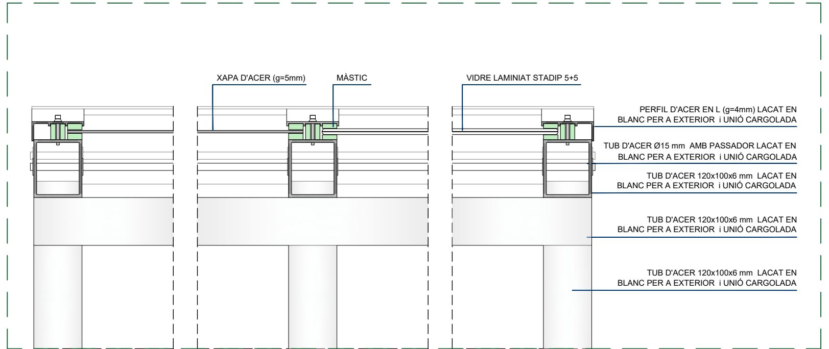
DETALL LLUERNA SECCIÓ FRONTAL
