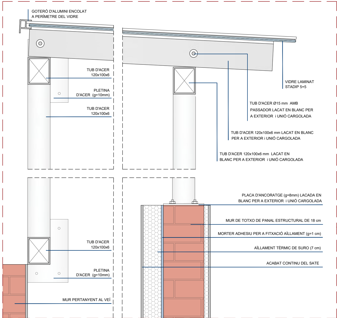
DETALL LLUERNA SECCIÓ LATERAL
