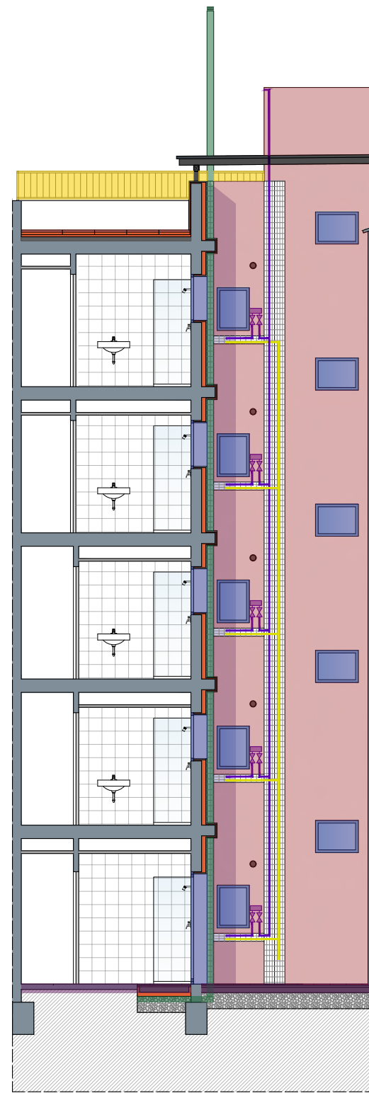
SECCIÓ TRANSVERSAL e=1:100
