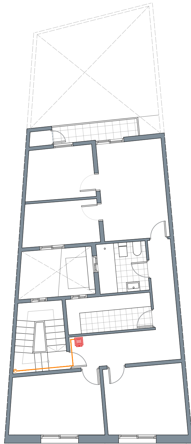
PLANTA TIPUS
