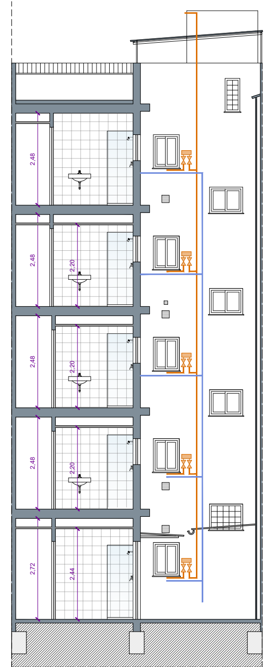
SECCIÓ PEL PATI
