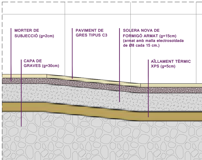
DETALL RAMPA (e=1:10)
