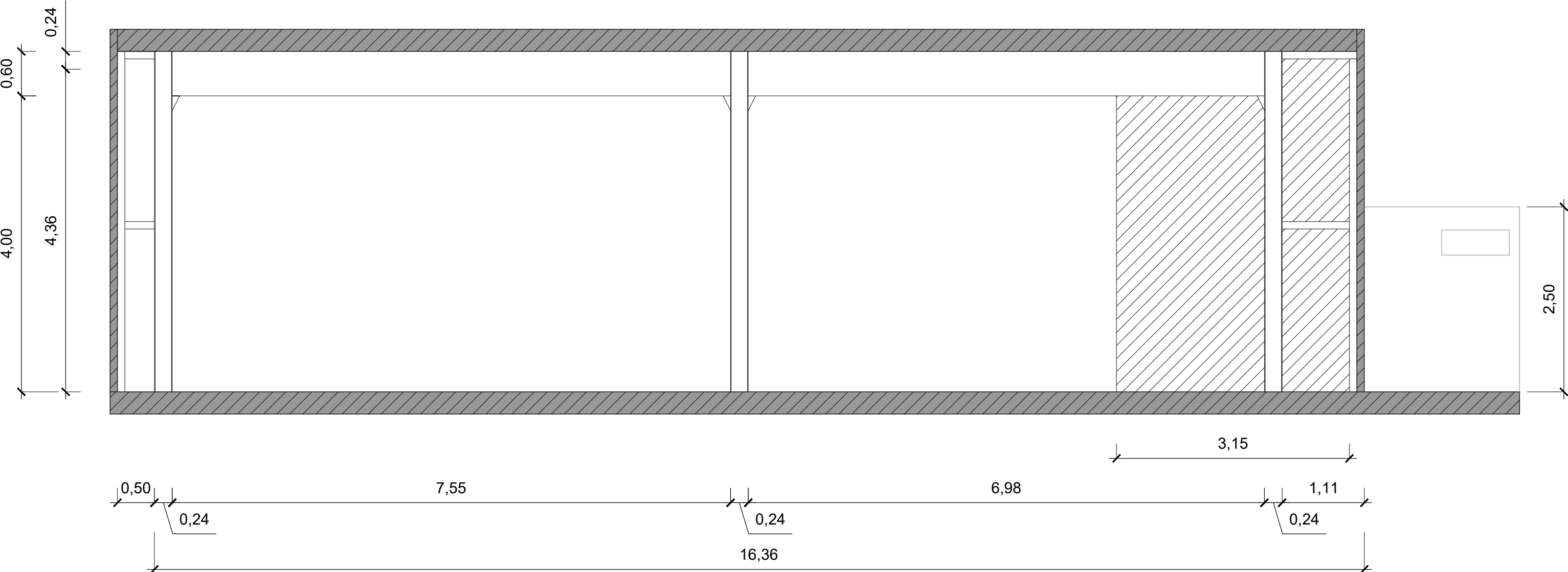
SECCIÓ B-B'
