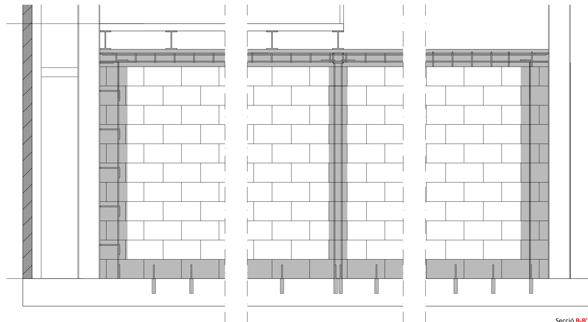
Secció B-B' E 1:20
